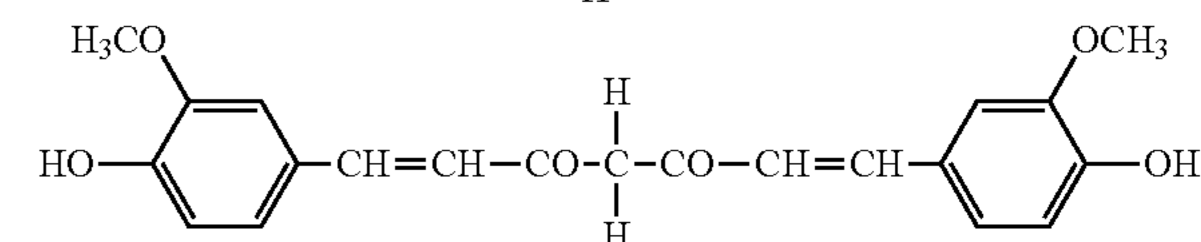
Curcumin
