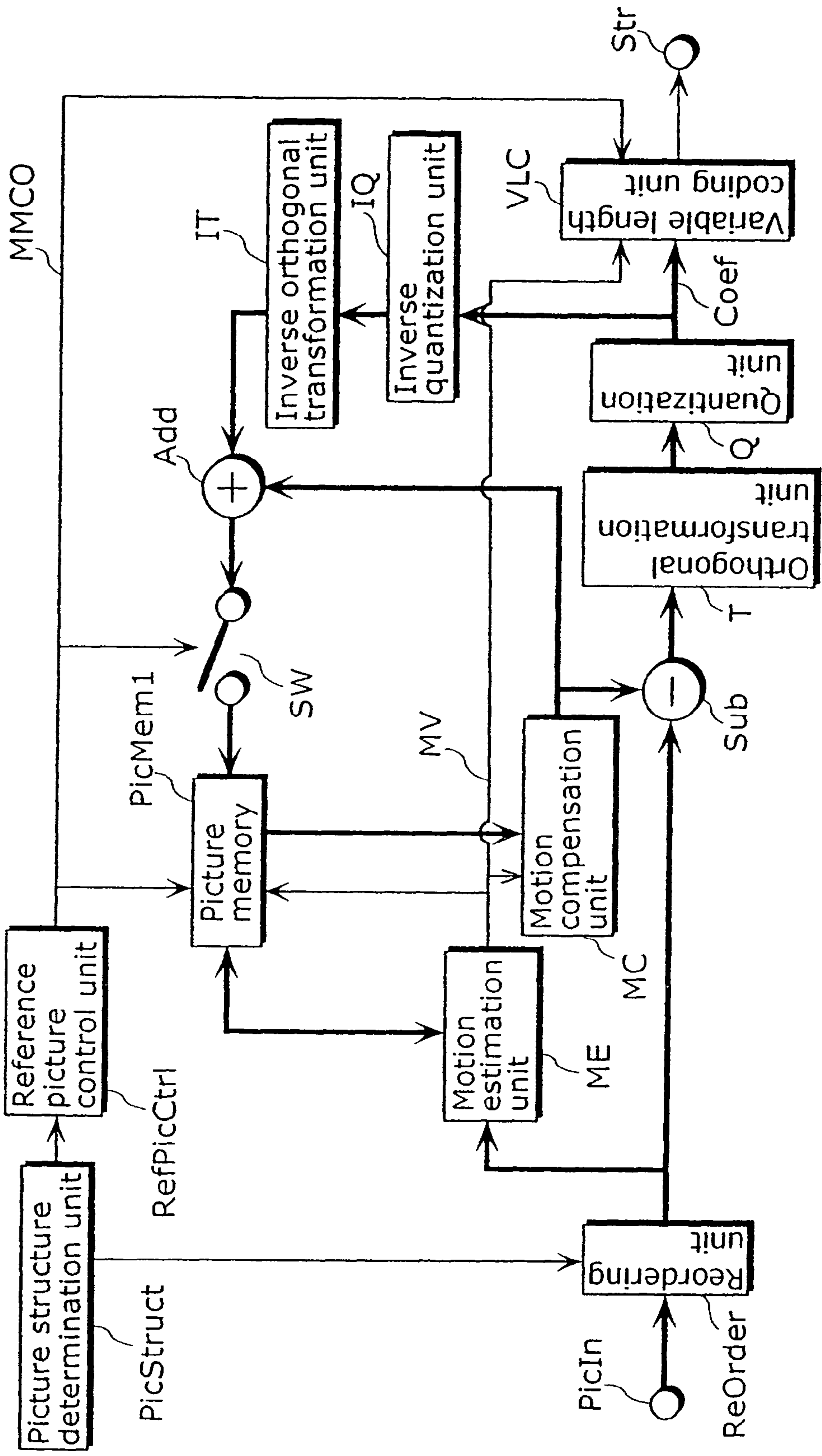
Fig. 26
