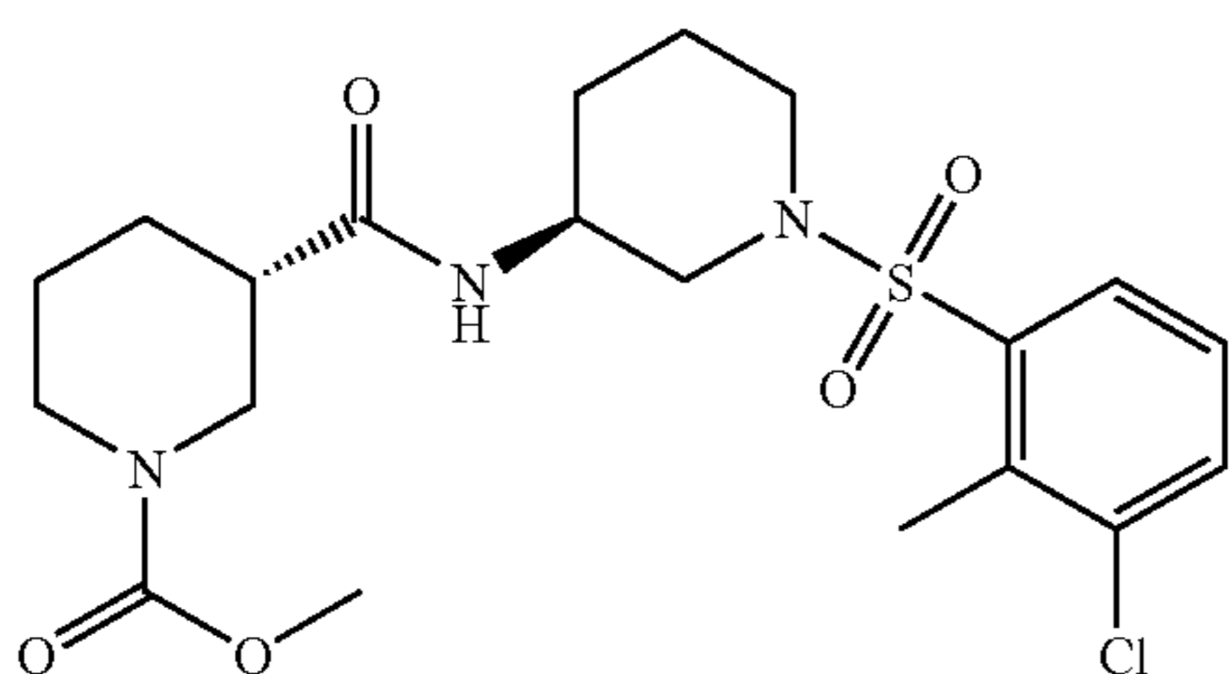
Example 174
