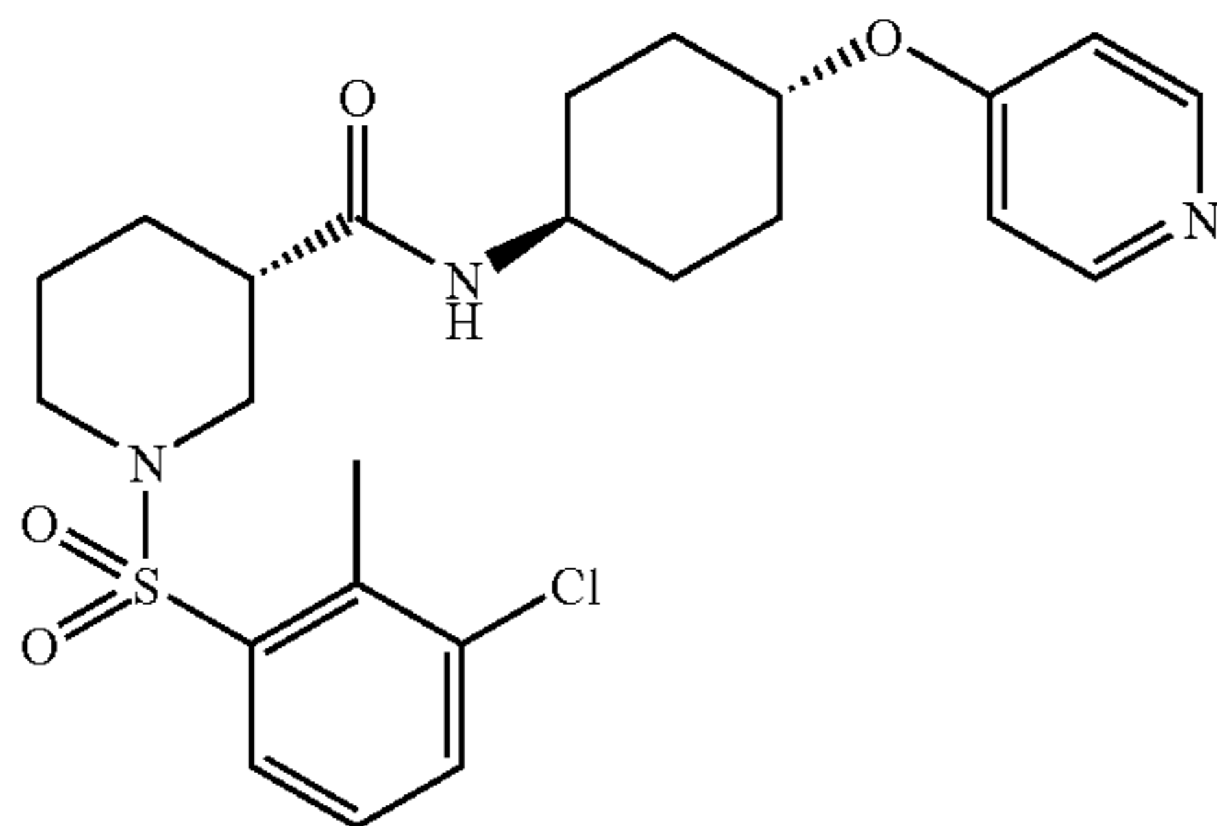
Example 127
