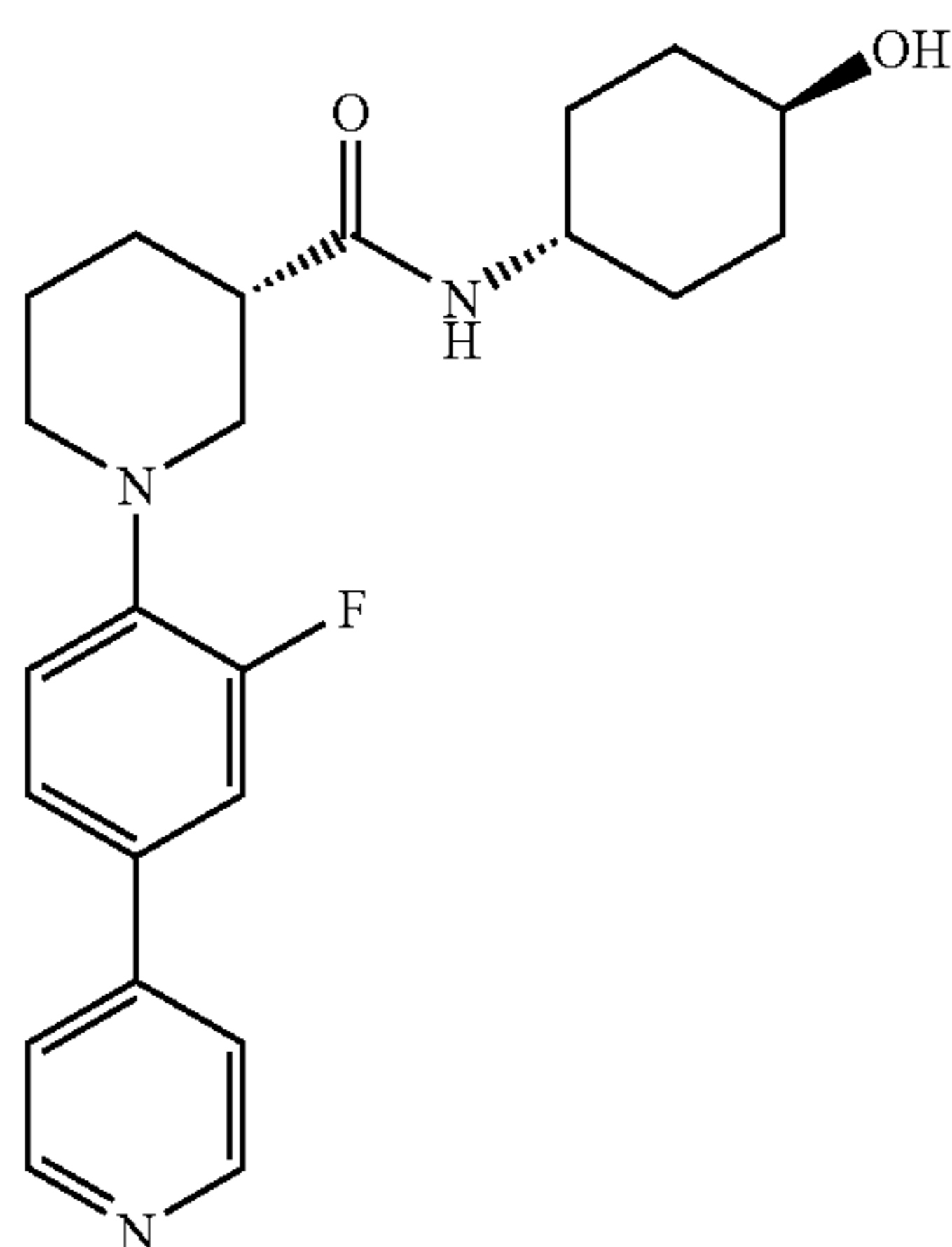
Example 170
