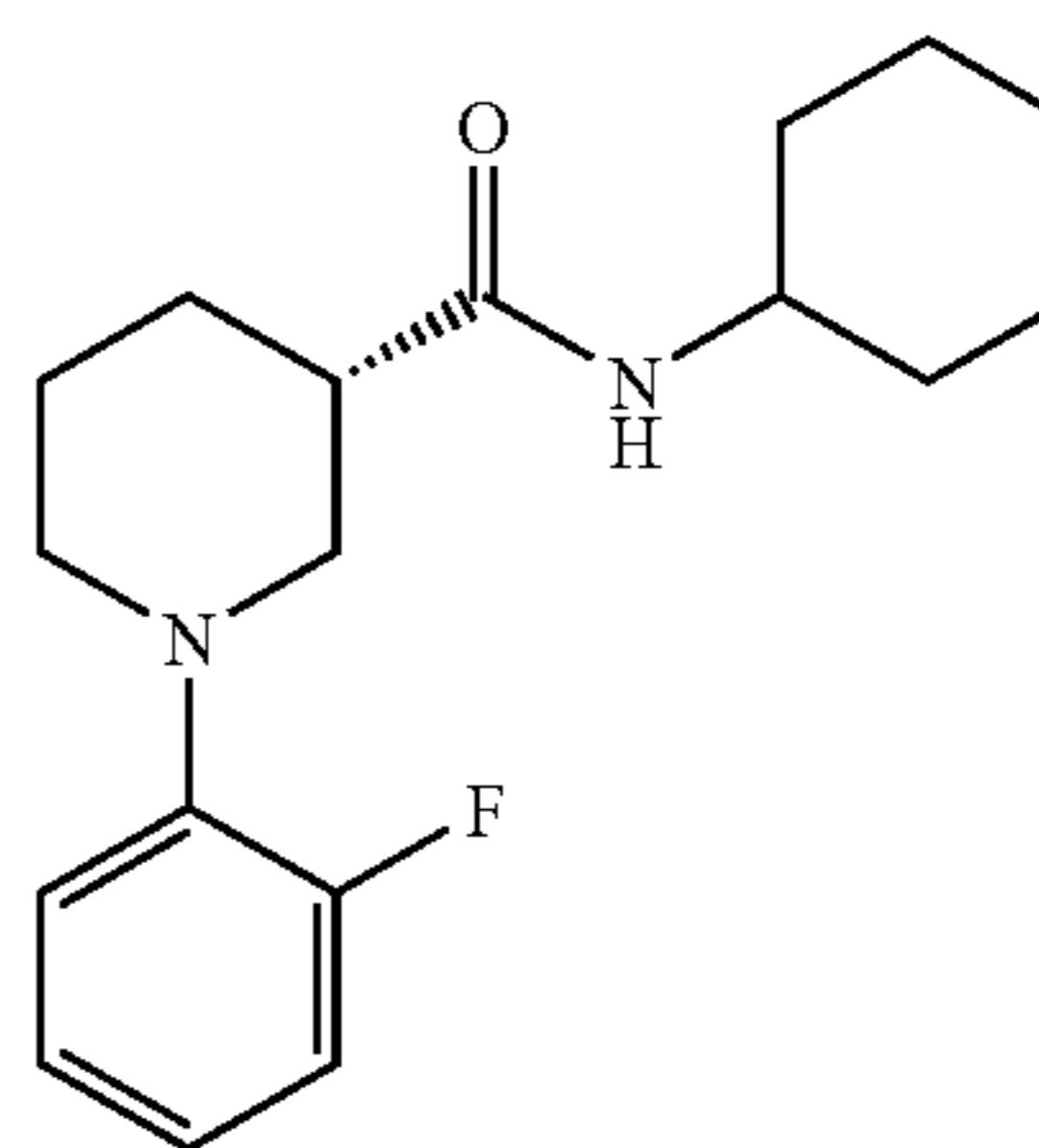
Example 133
