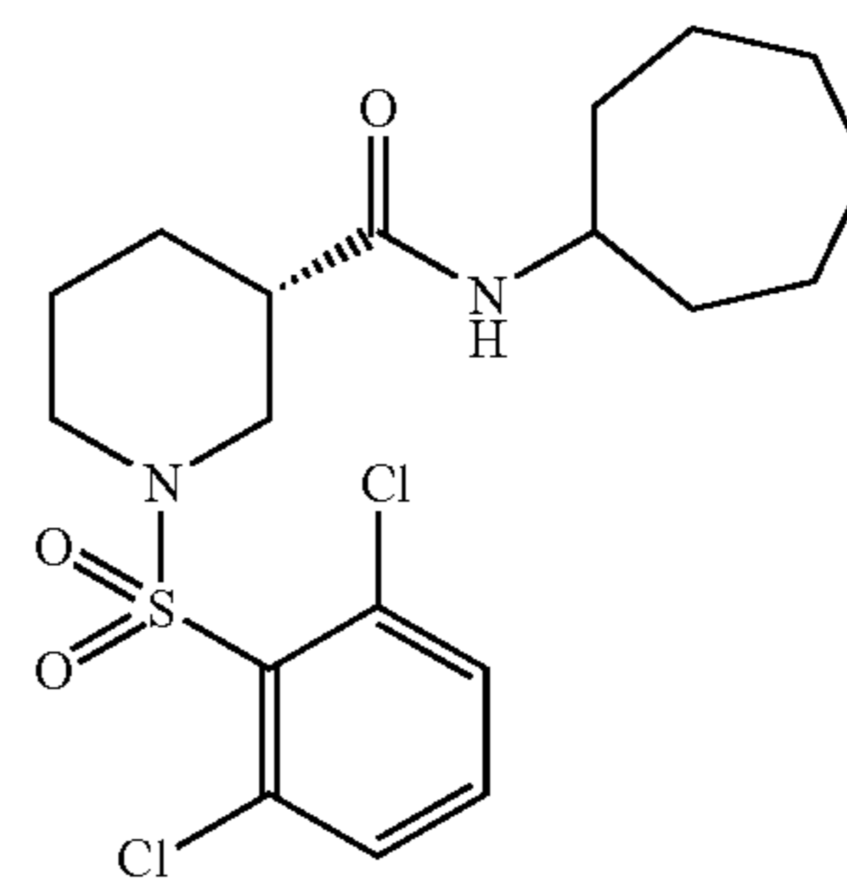
Example 108
