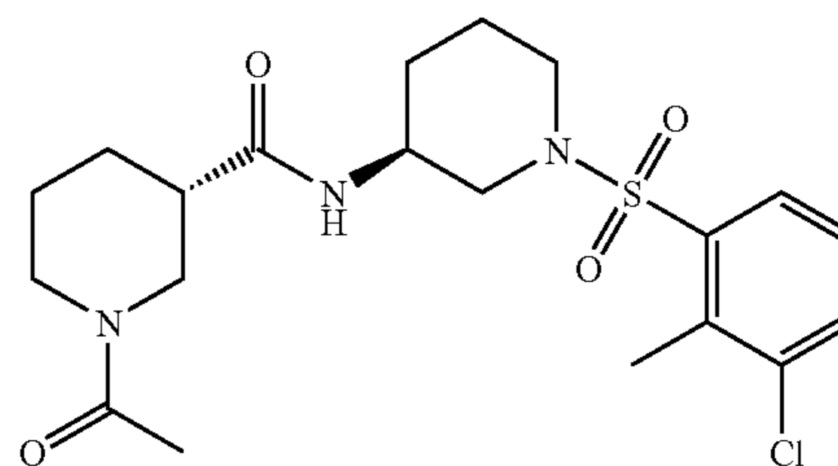
Example 173
