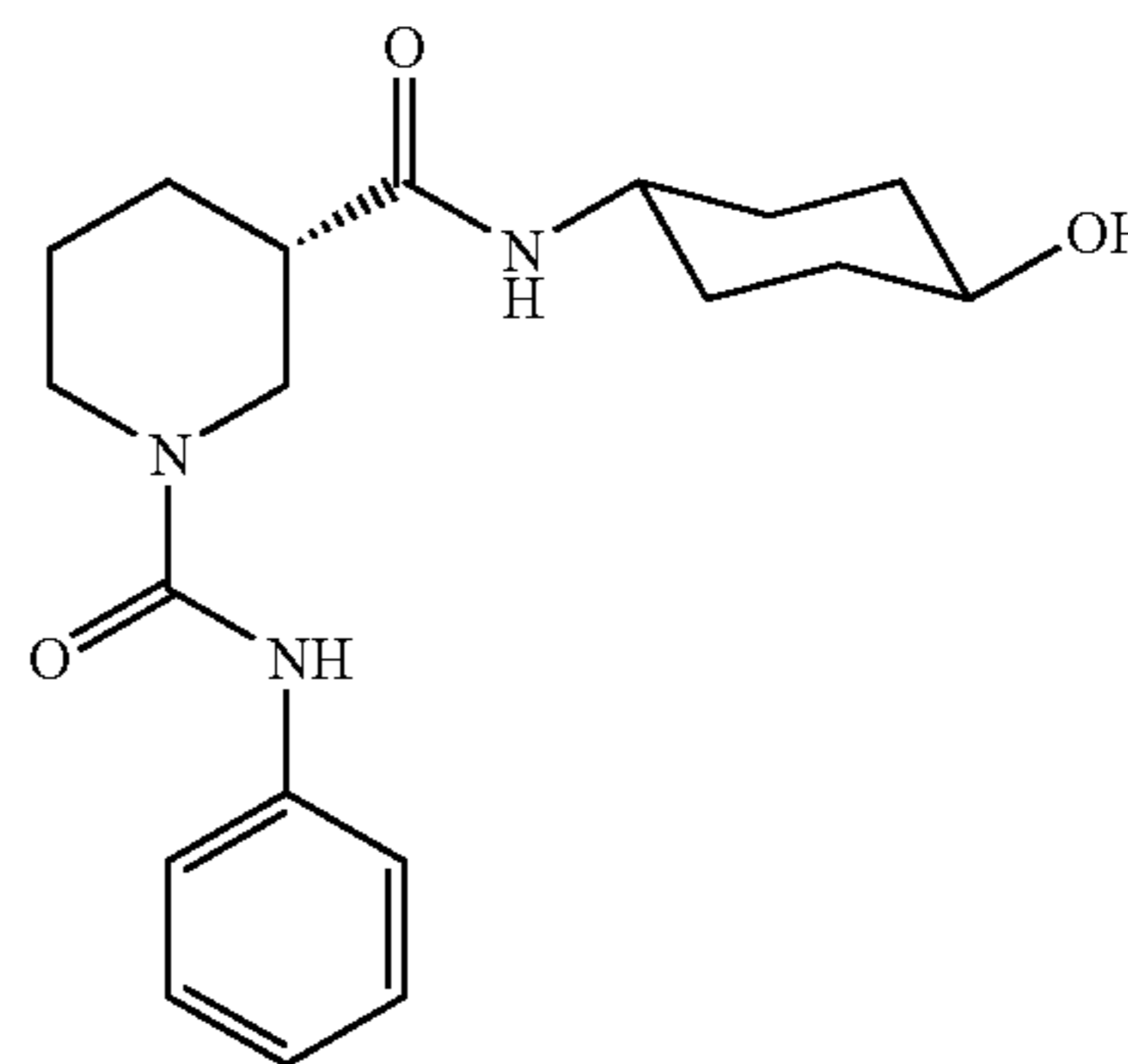
Example 178
