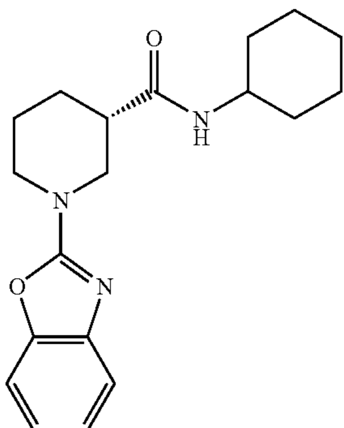
(3S)-1-(1,3-Benzoxazol-2-yl)-N-cyclohexylpiperidine-3-carboxamide
