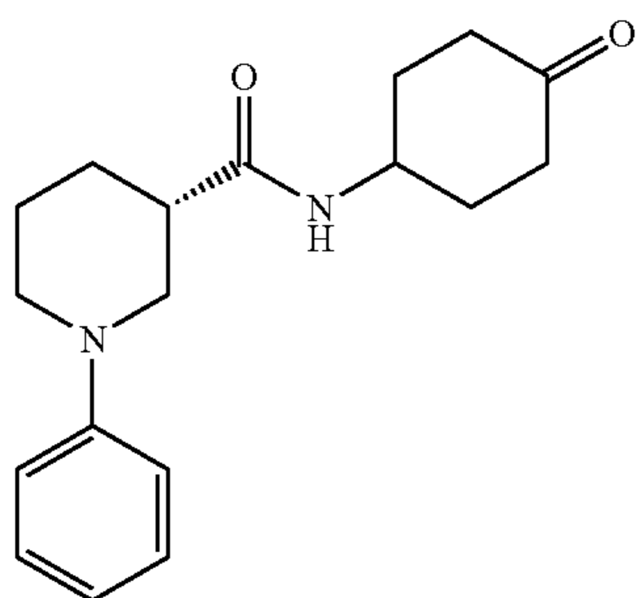
Example 171
