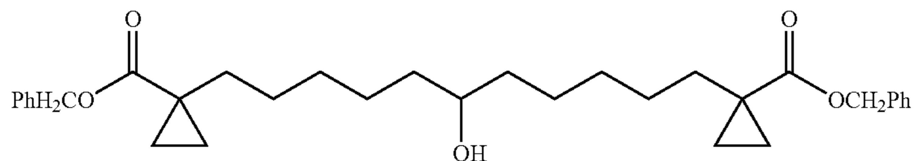
1,11-Bis-(1-benzyloxycarbonyl-cyclopropyl)-undecan-6-ol
