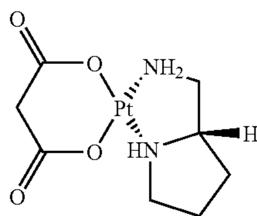
Miboplatin
