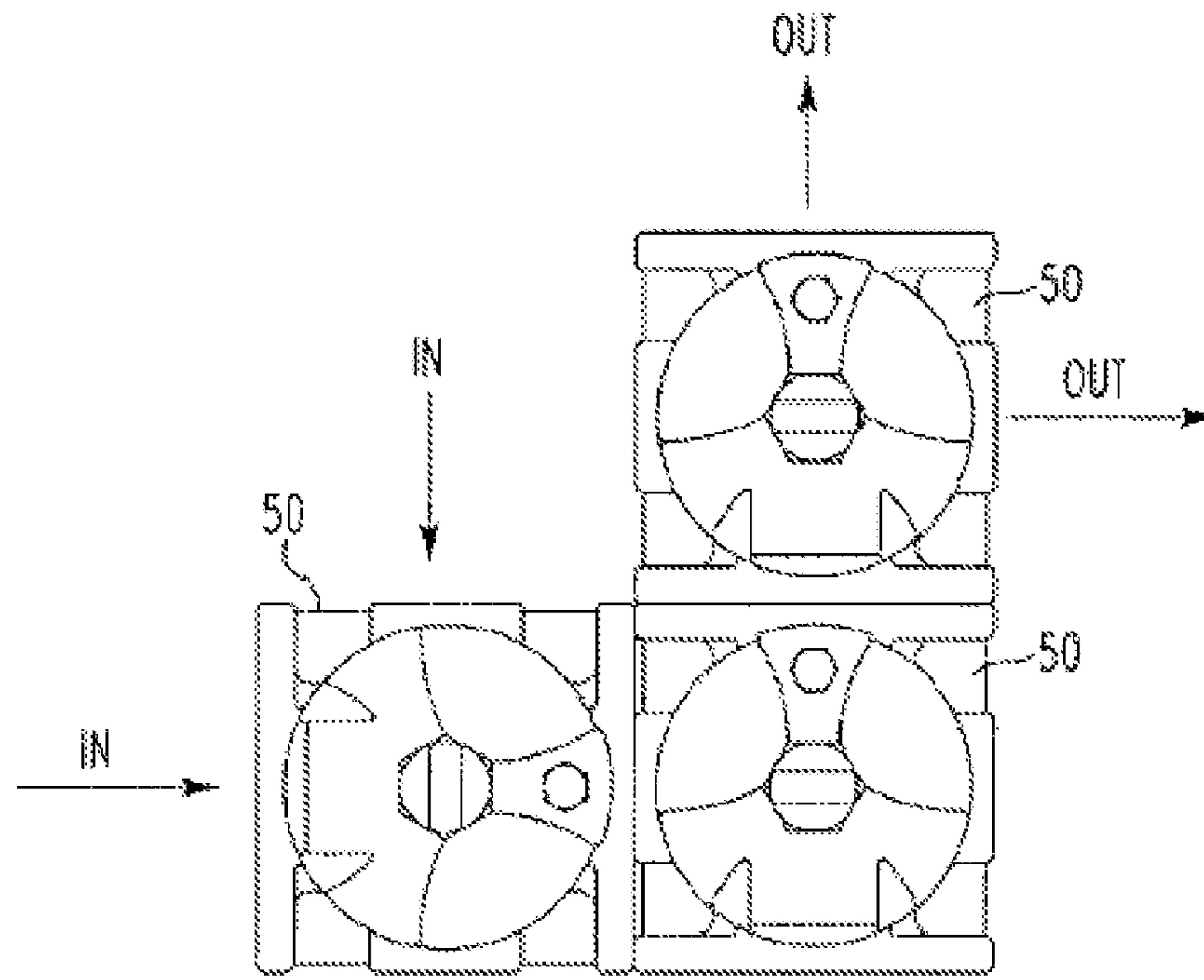
FIG. 13-A
