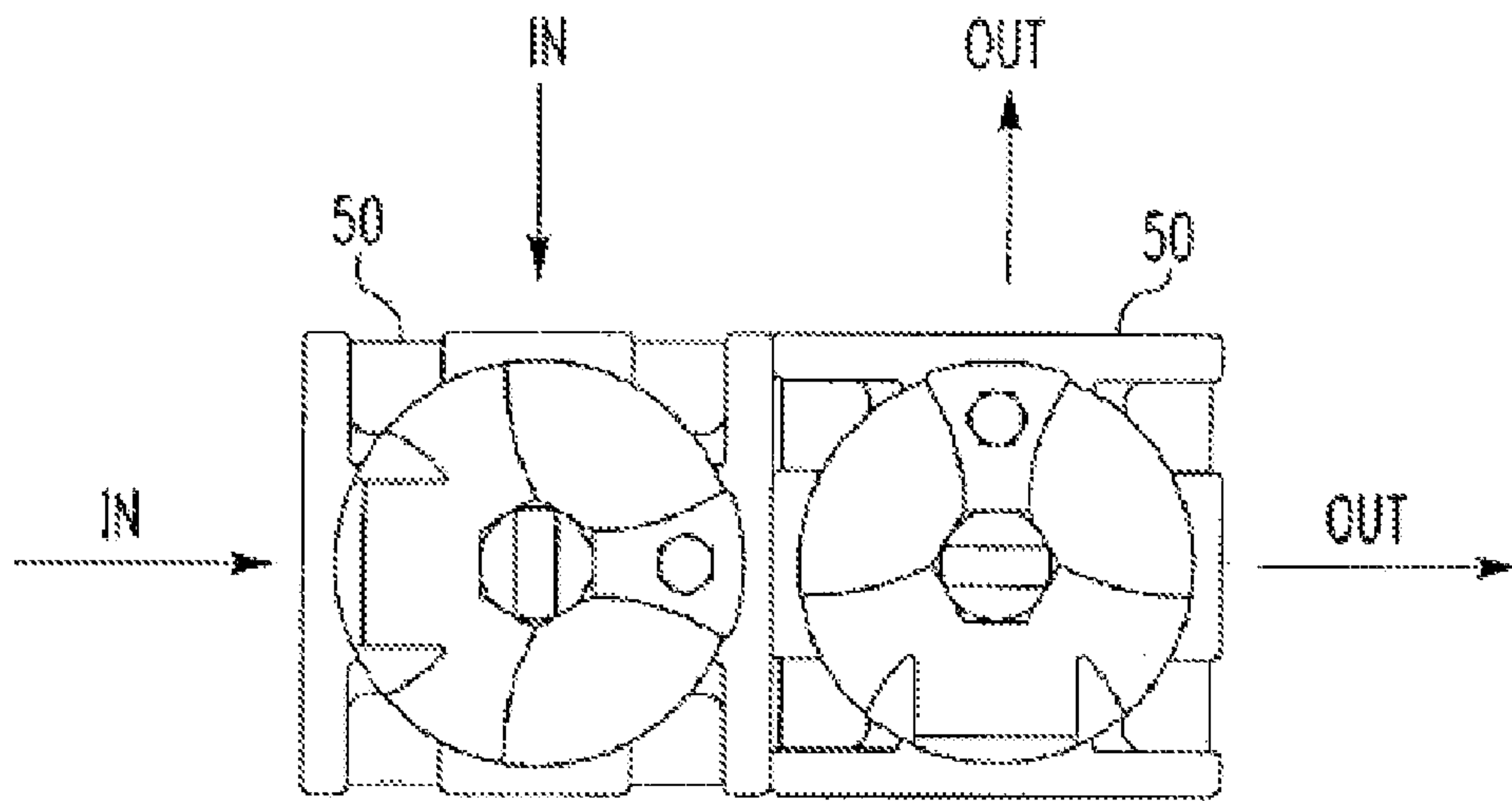
FIG. 8-A
