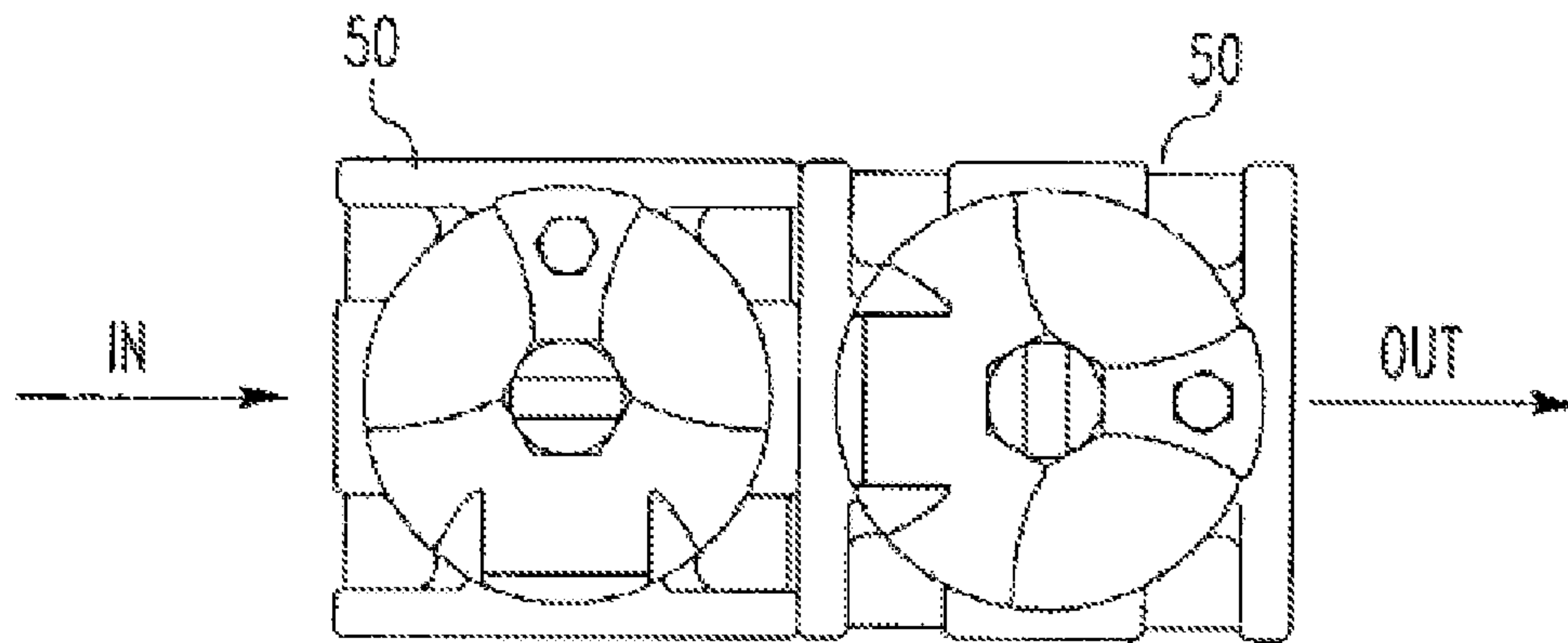
FIG. 10-A ↑ IN ↓ OUT
