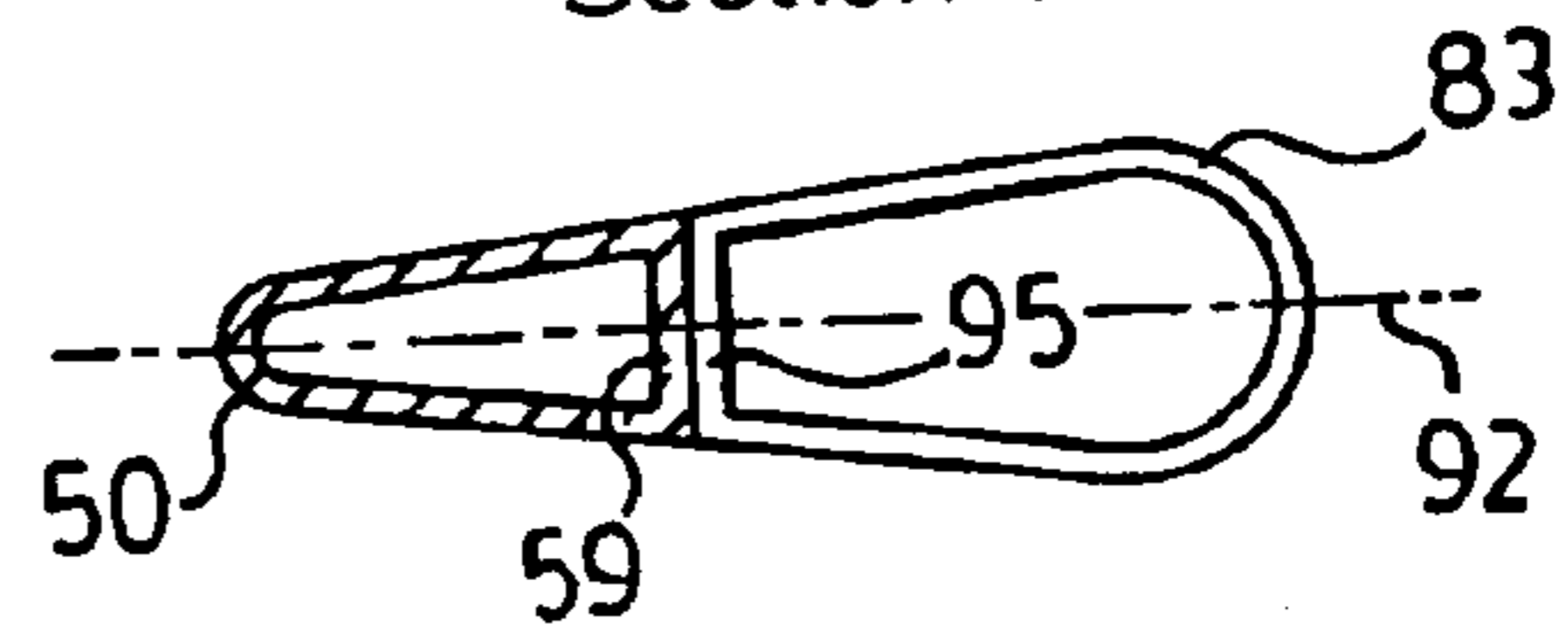
FIG. 18. Section C-C
