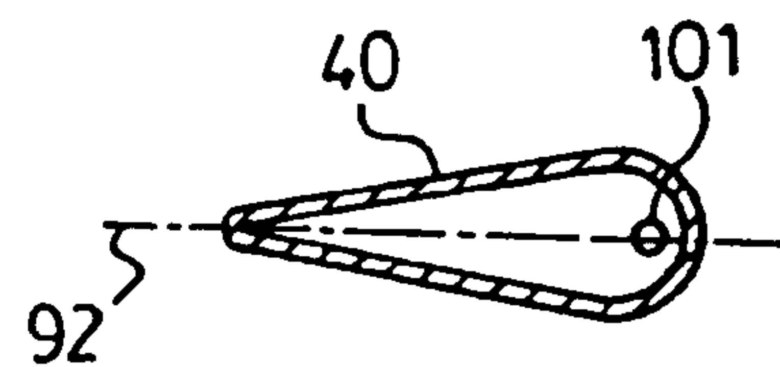
FIG. 10. Section F-F
