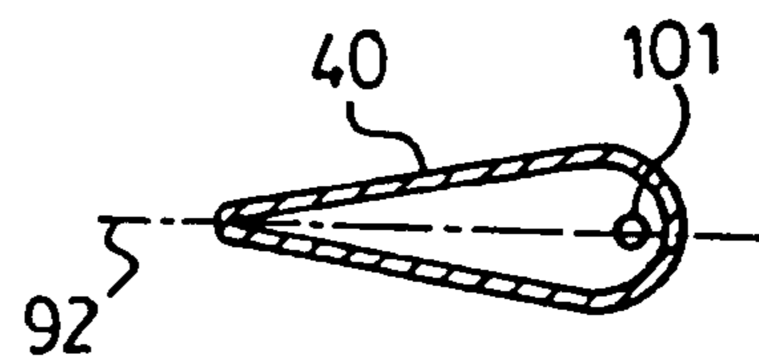
FIG. 10. Section F-F
