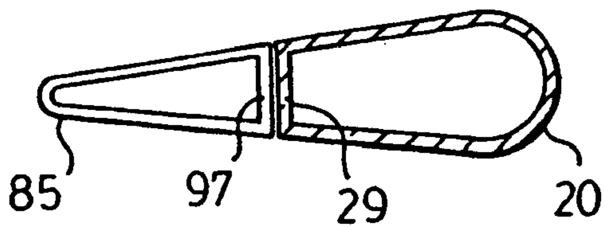
FIG. 26. Section A-A
