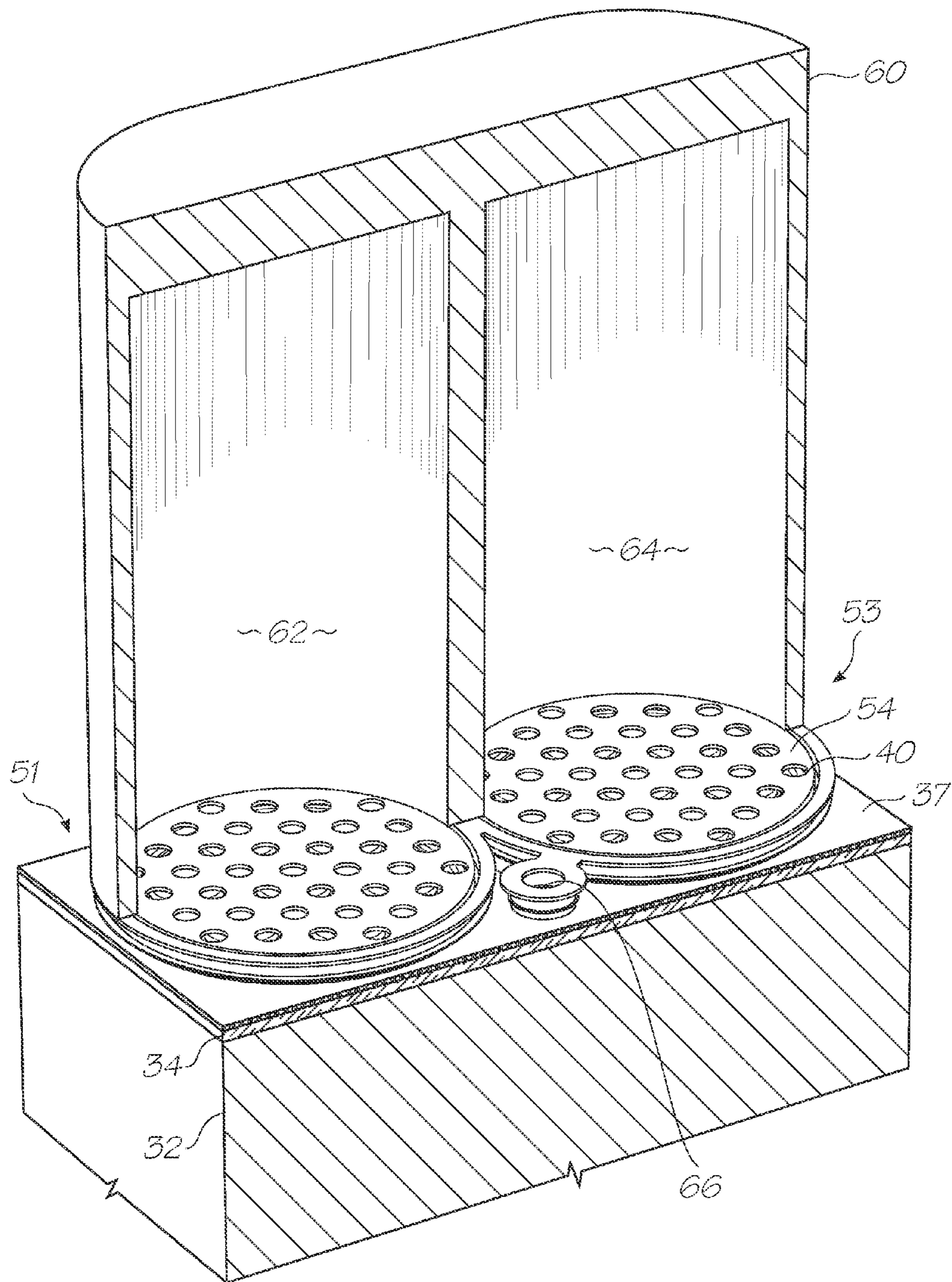
FIG. 27(B)
