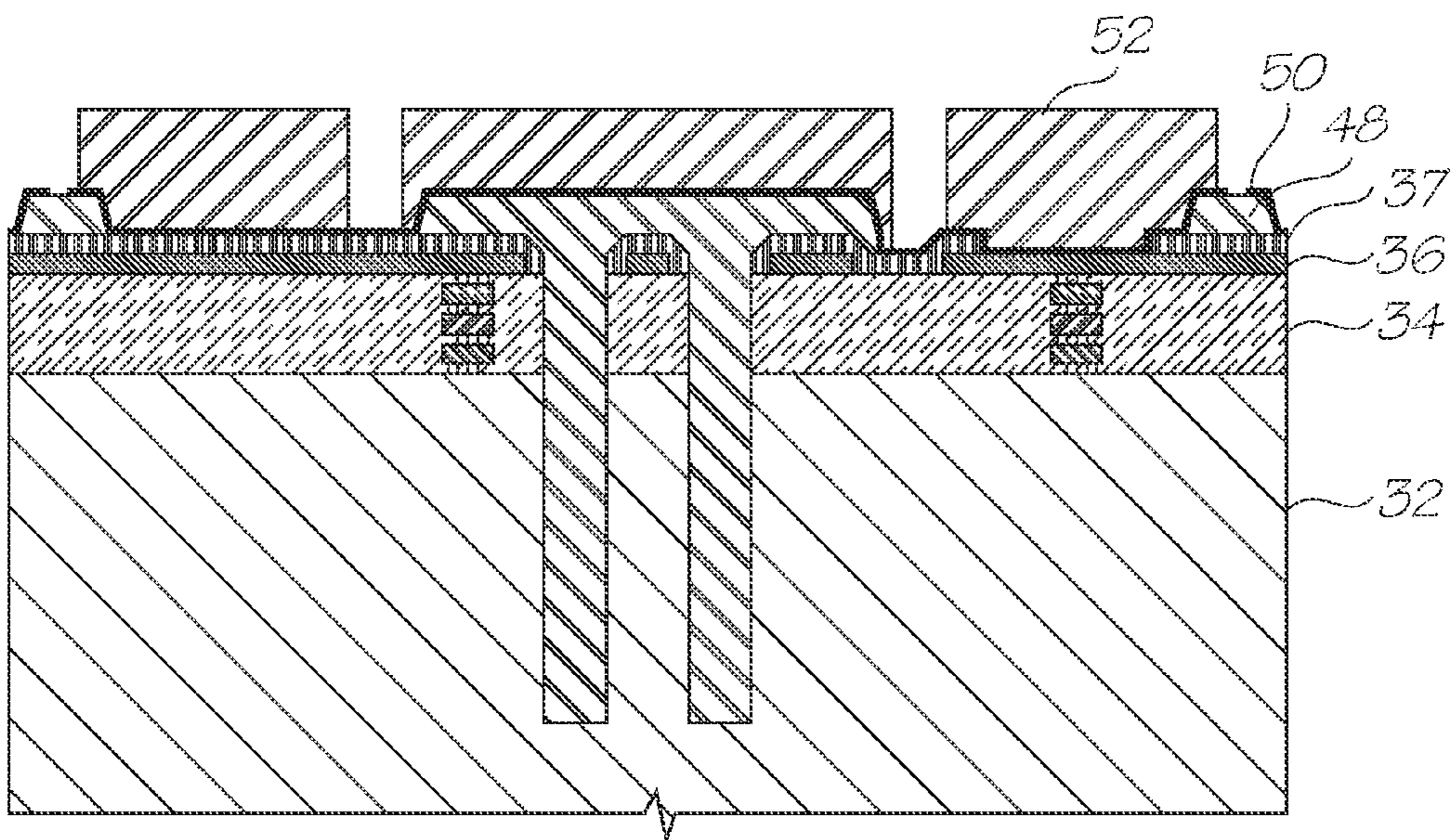
FIG. 16
