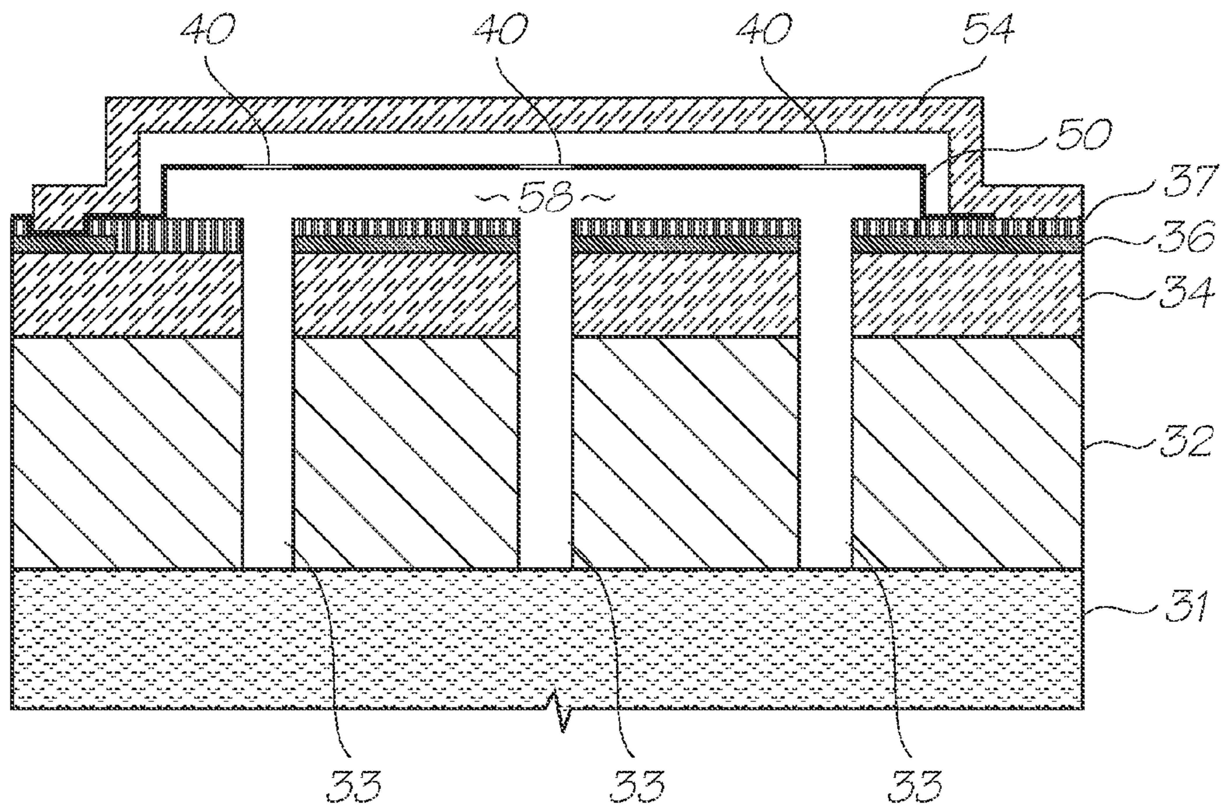
FIG. 24
