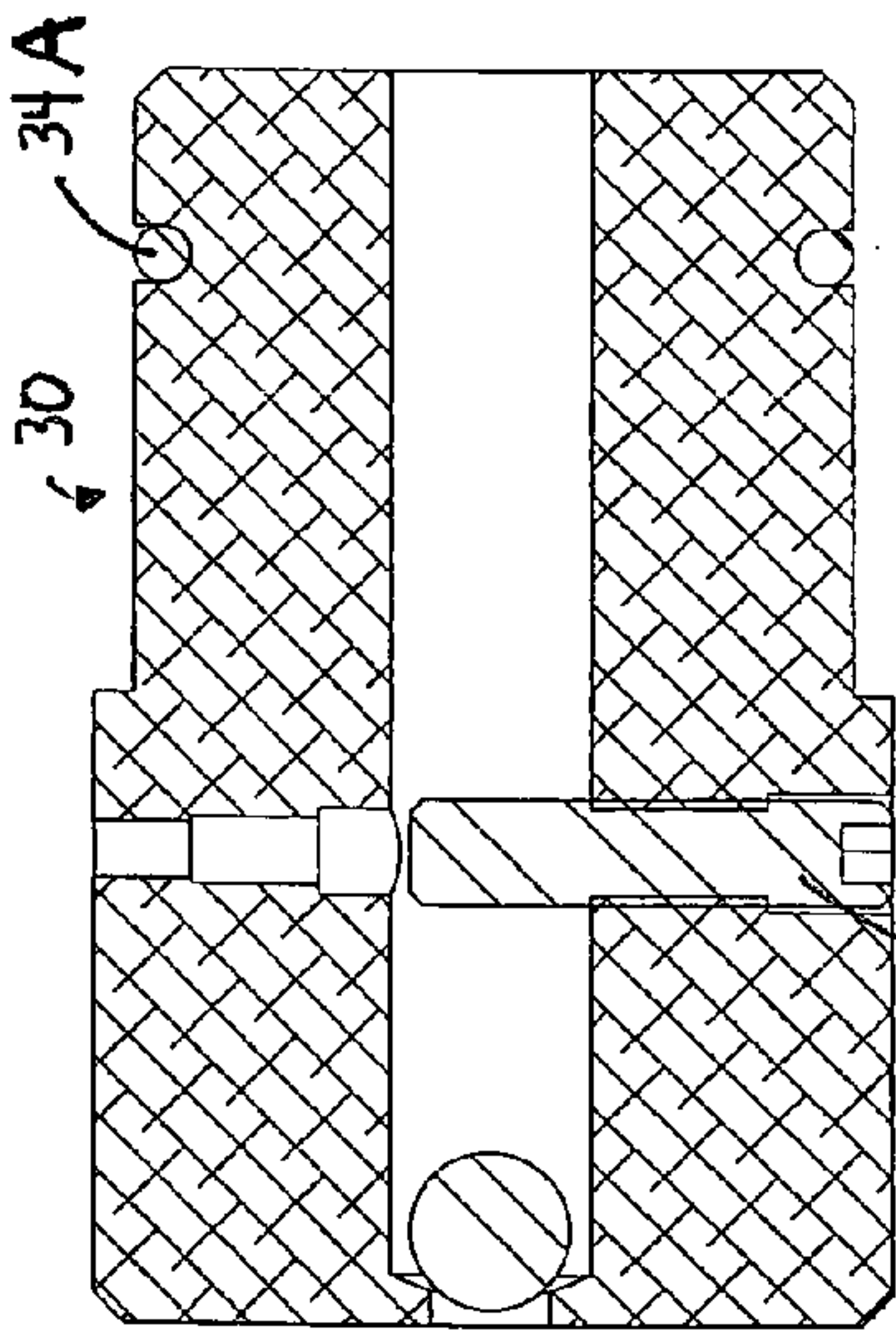
FIG. 4C SECTION J-J SCALE 2:1
