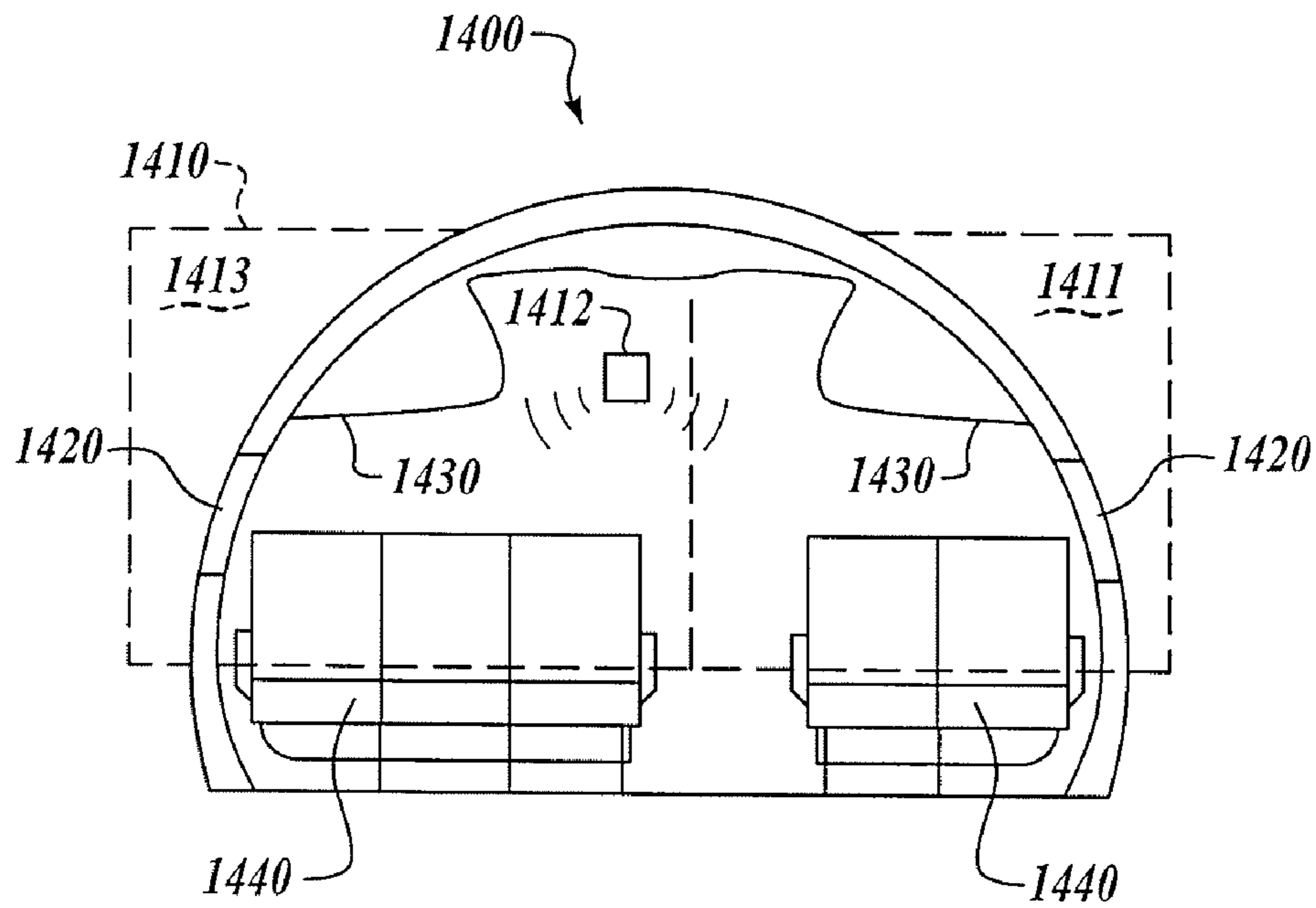
FIG. 15A
