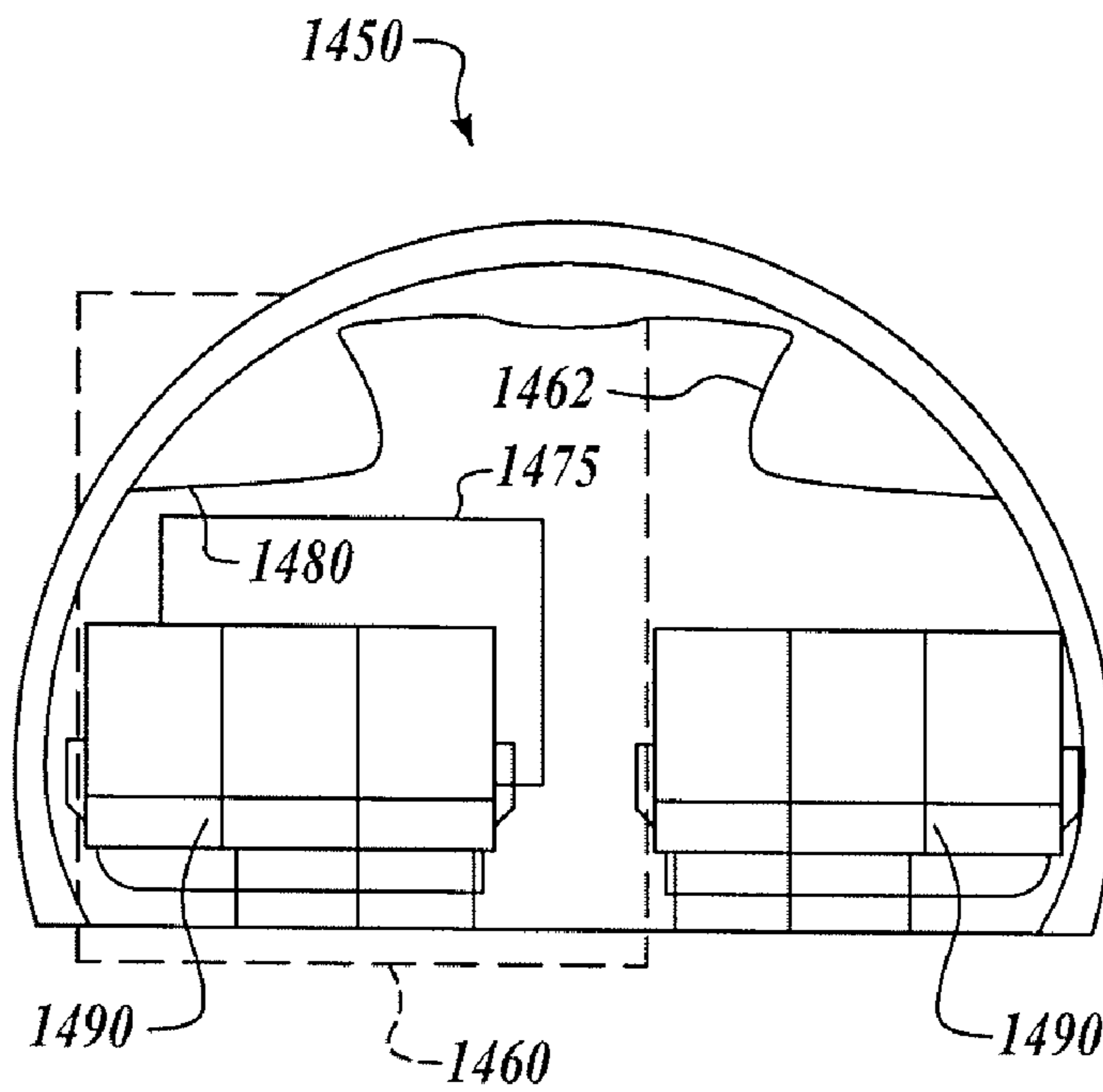
FIG. 15B
