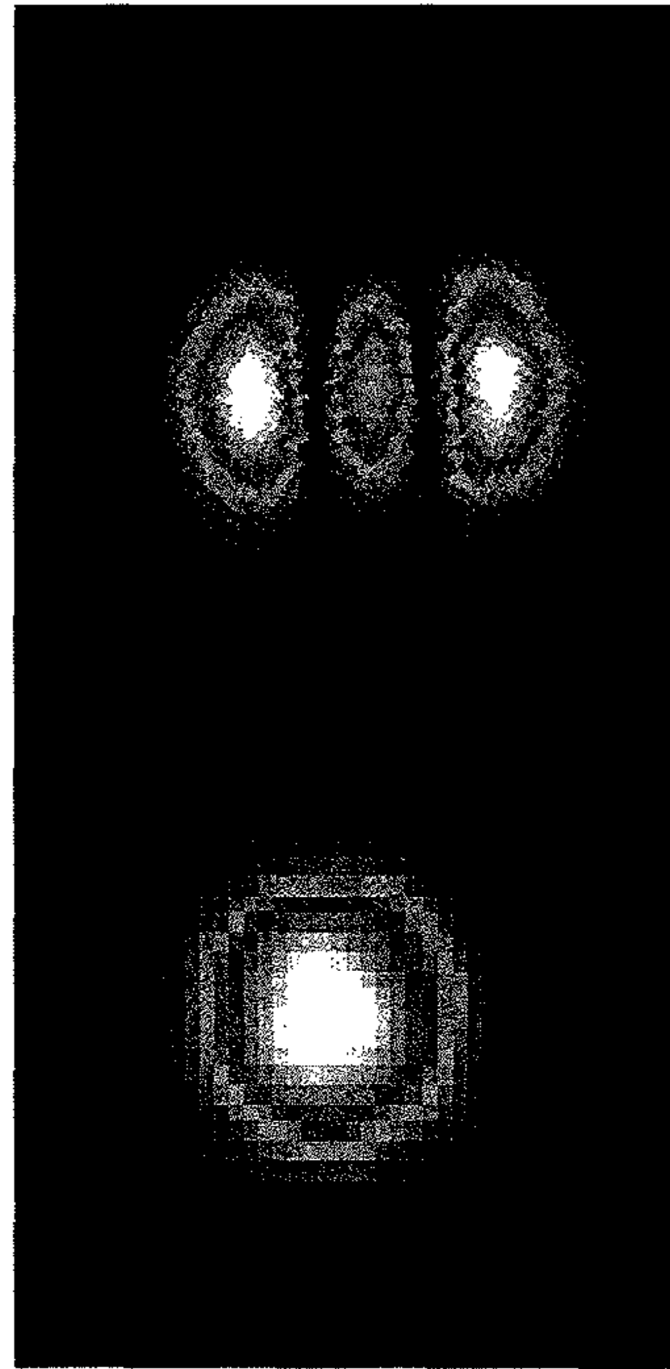
TEM_{00} TEM_{02}
