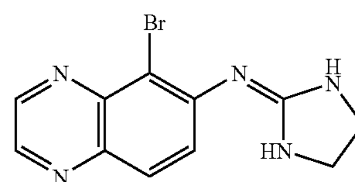
brimonidine
