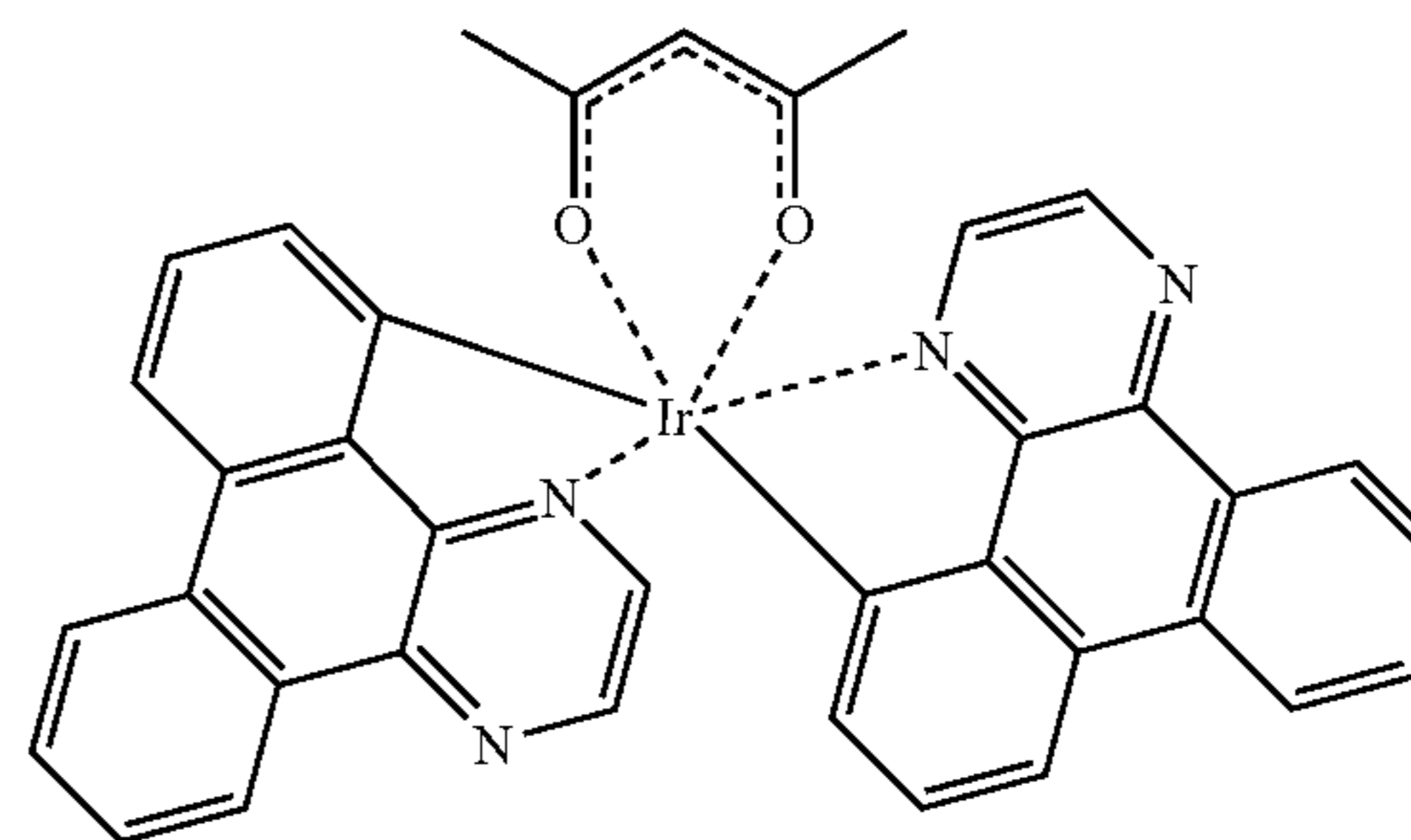
Ir(DBQ) 2 (acac) 4
