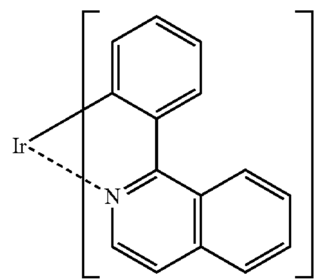
Ir(pi q) 3 6
