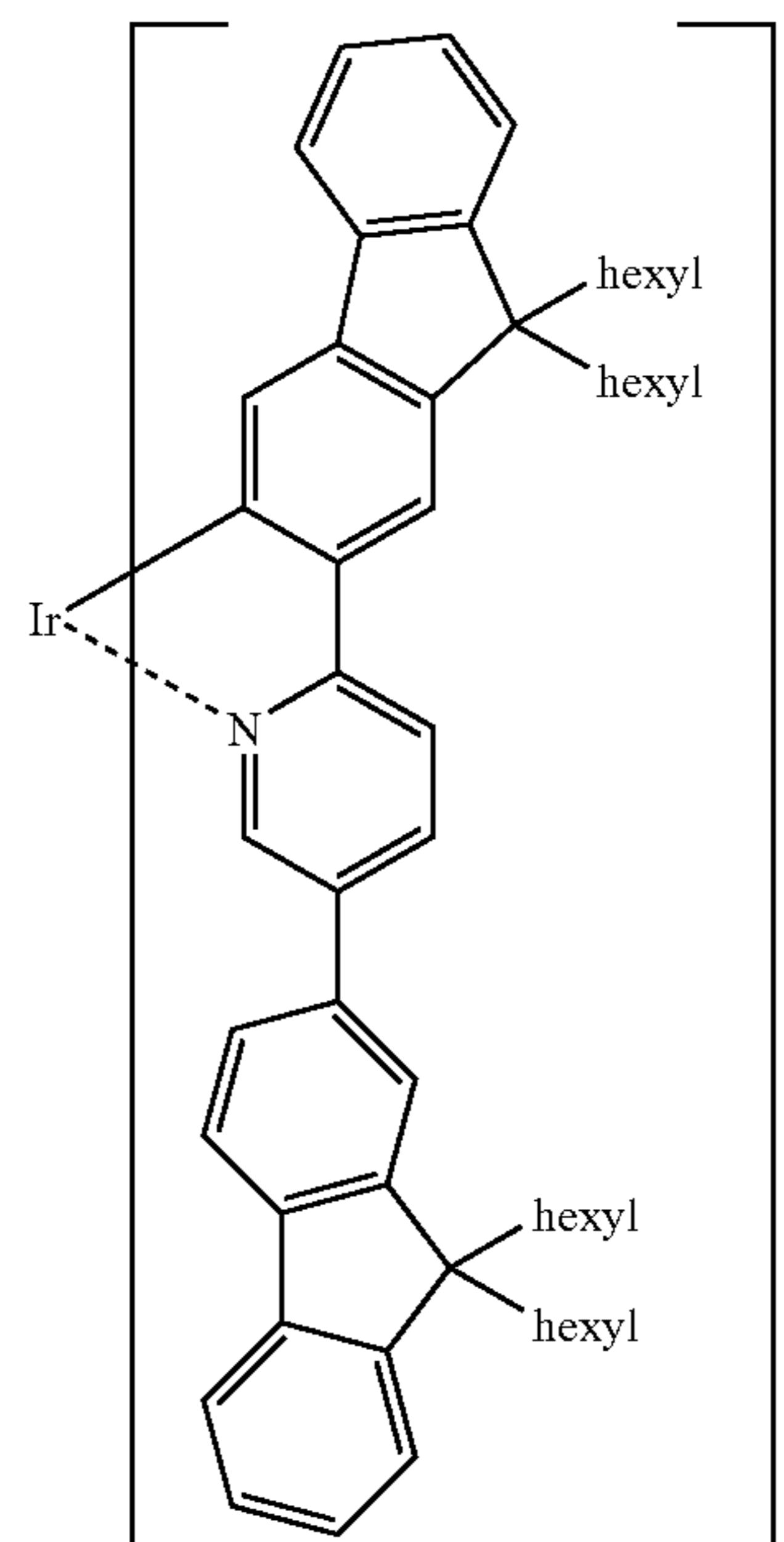
Ir(HFP) 3 5
