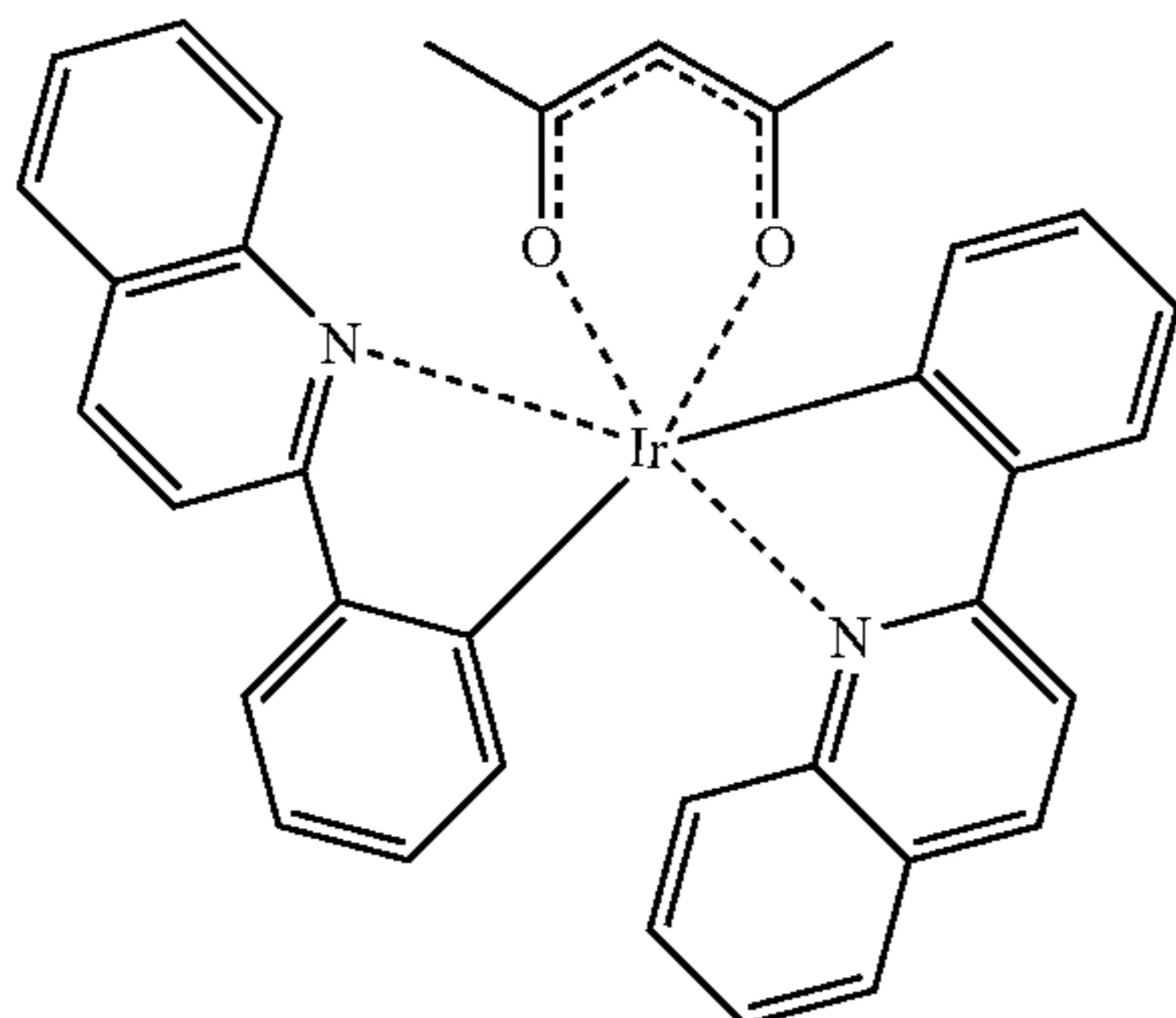
Ir(pq) 2 (acac) 2
