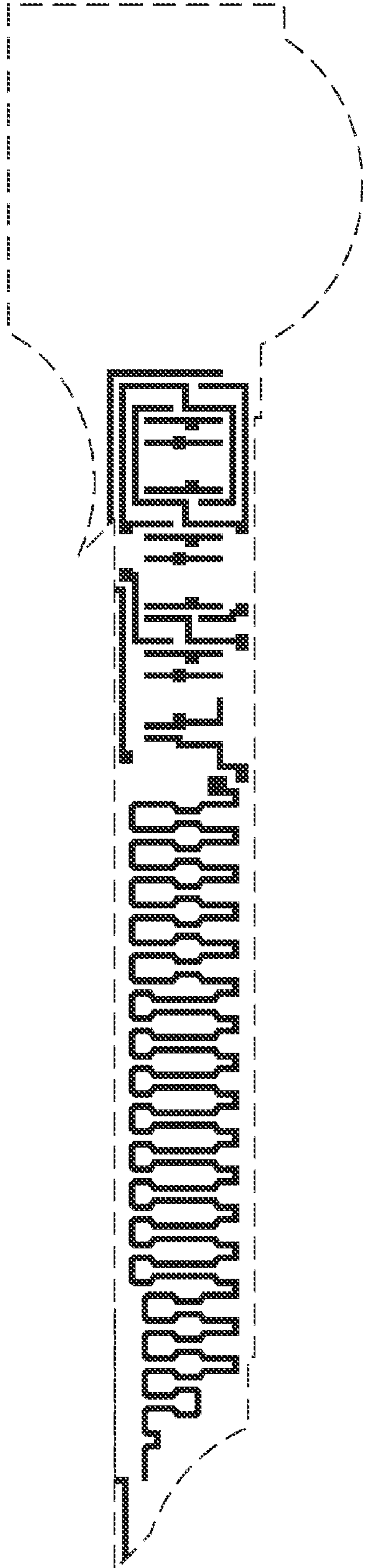
Poly mask
