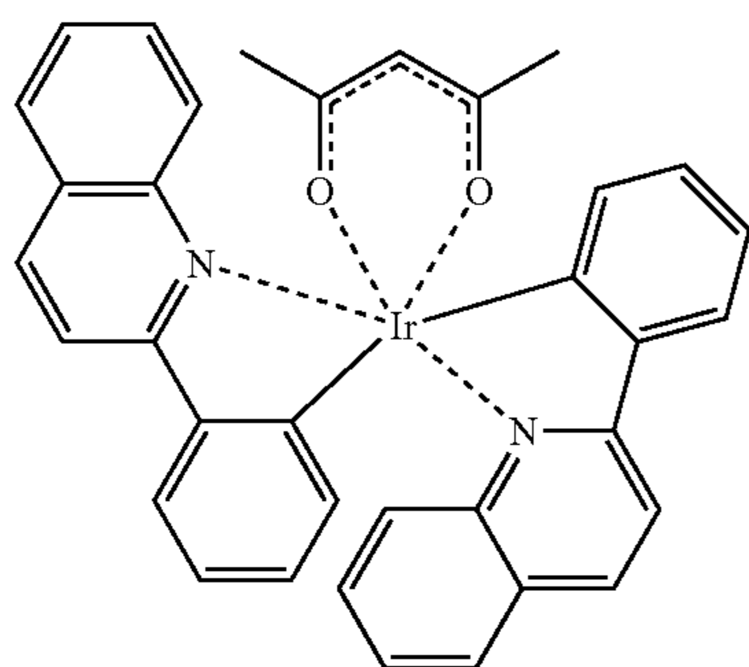
Ir(pq) 2 (acac)
