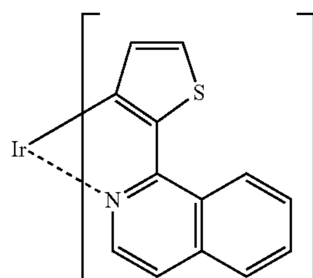
Ir(tiq) 3
