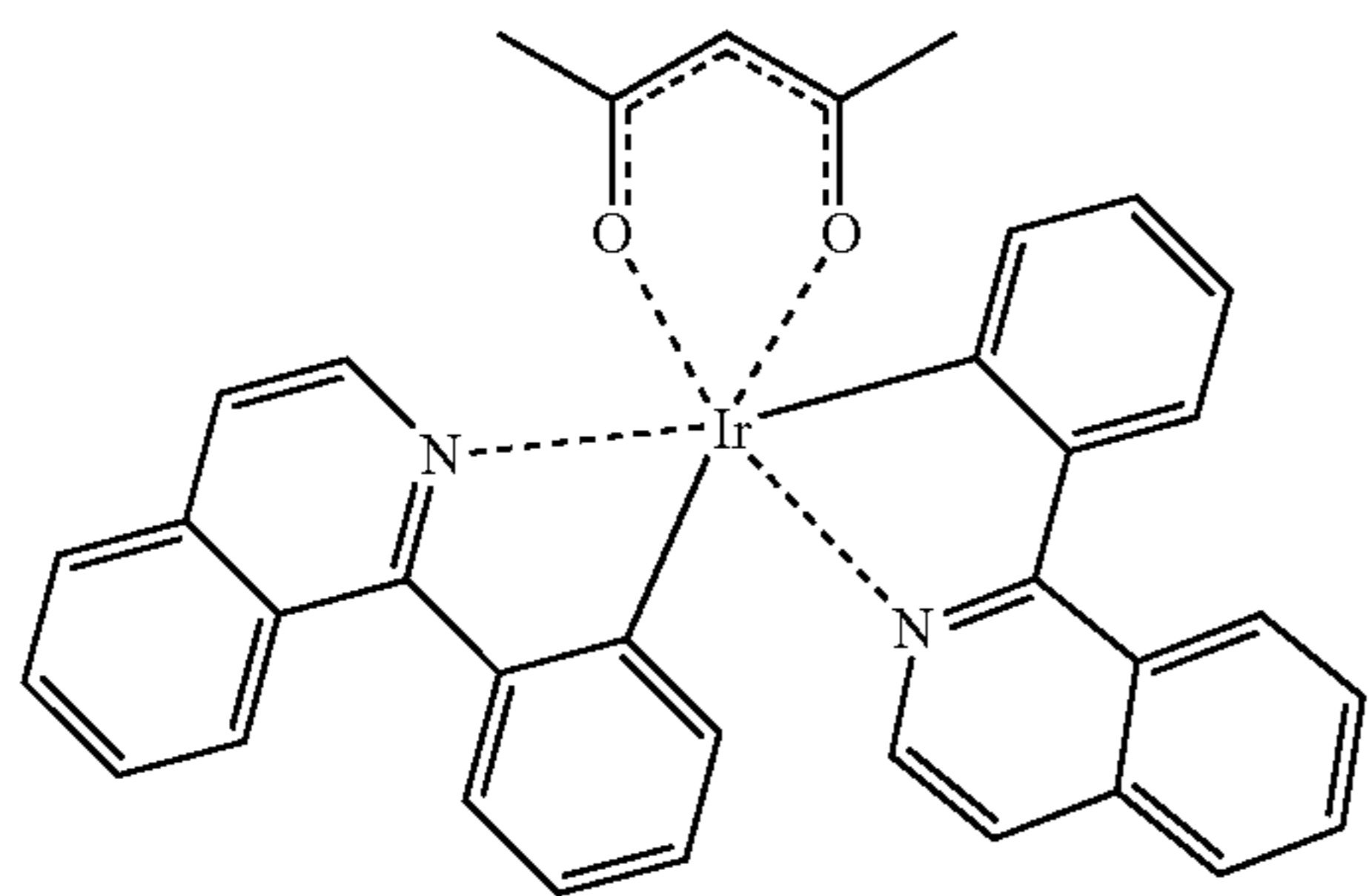
Ir(piq) 2 (acac)
