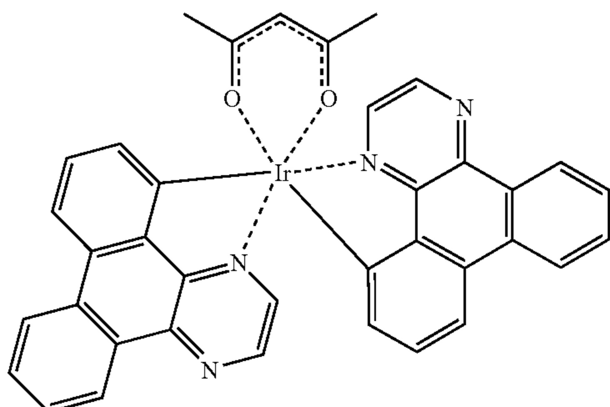
Ir(DBQ) 2 (acac)
