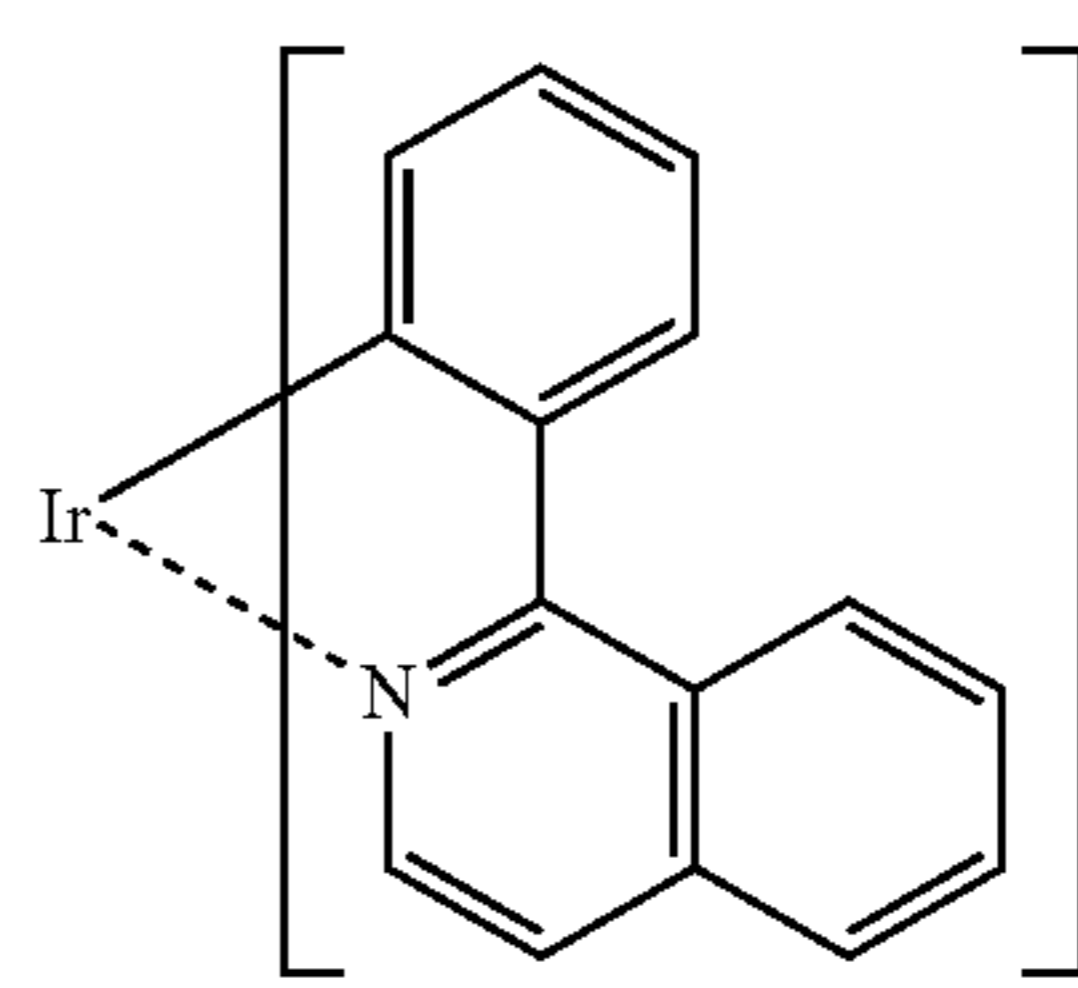
Ir(piq) 3
