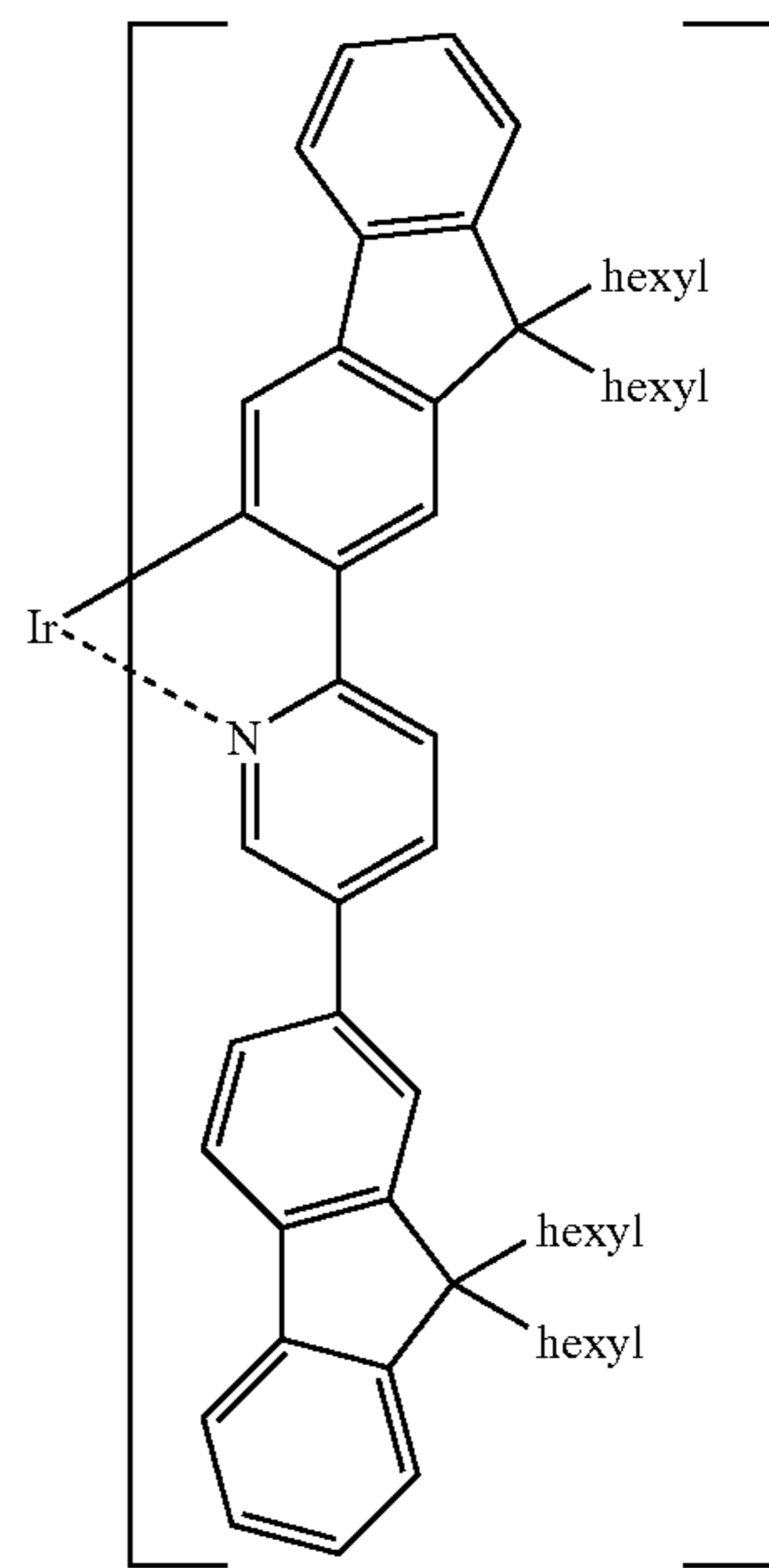
Ir(HFP) 3
