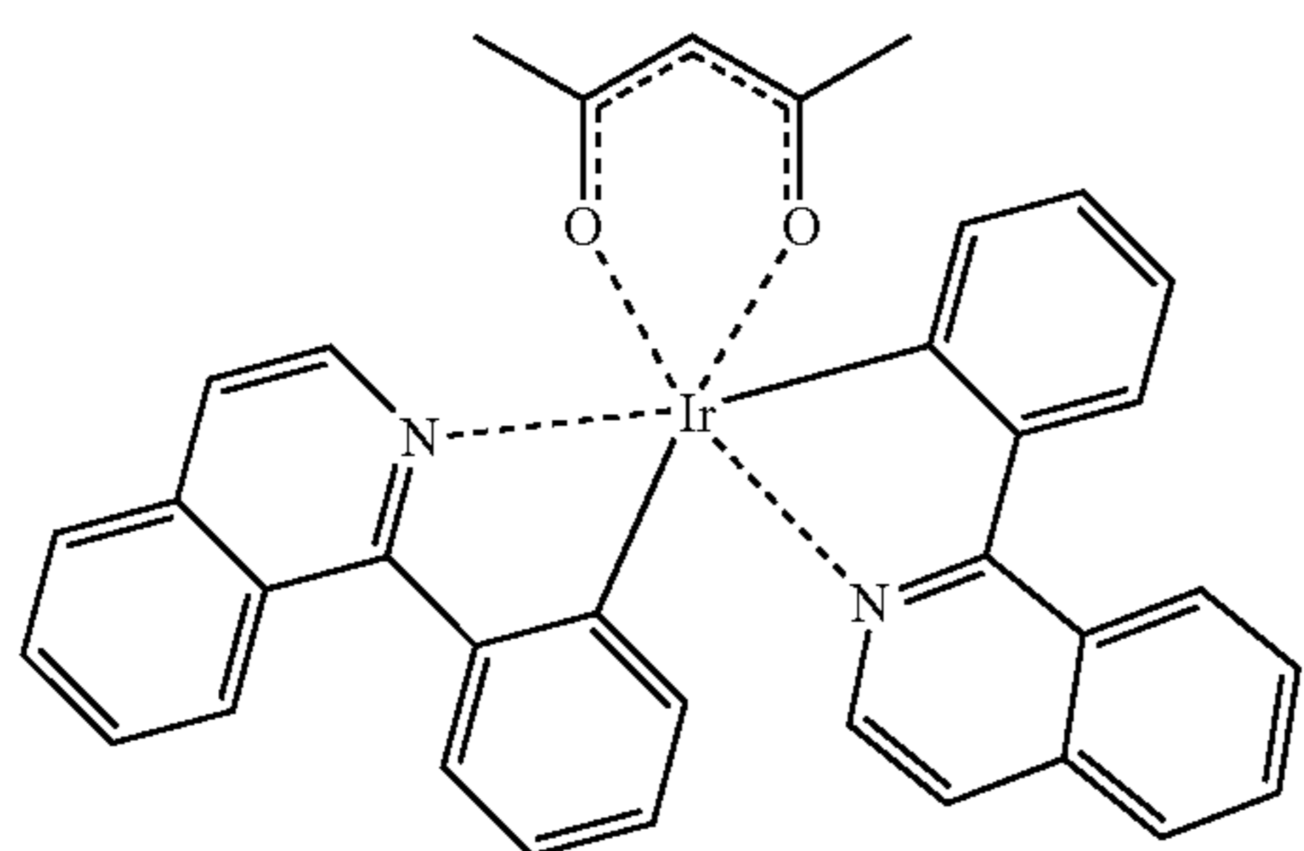
Ir(piq) 2 (acac)
