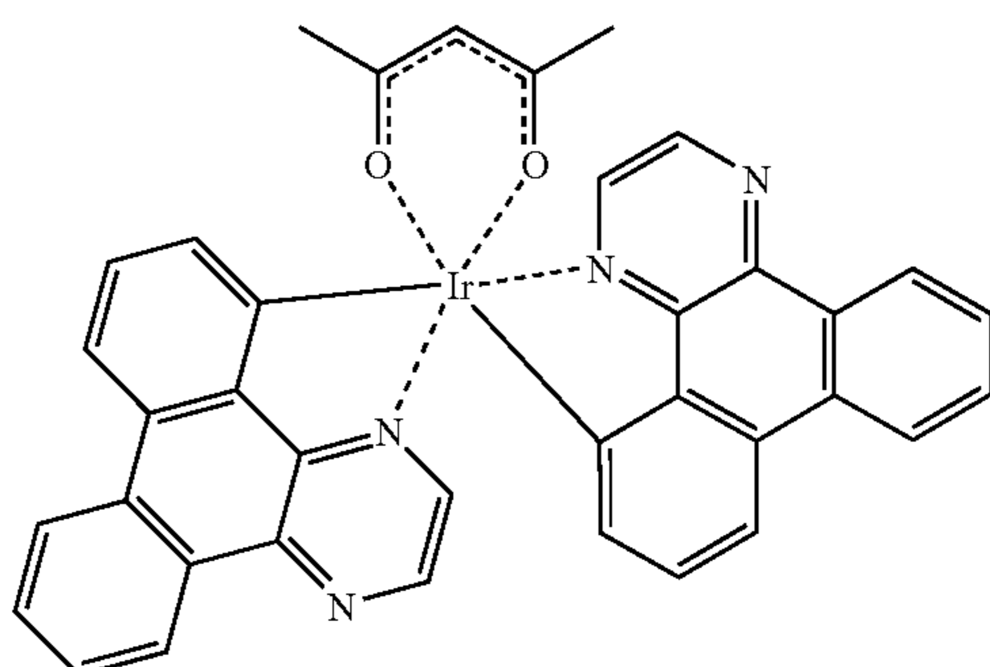
Ir(DBQ) 2 (acac)
