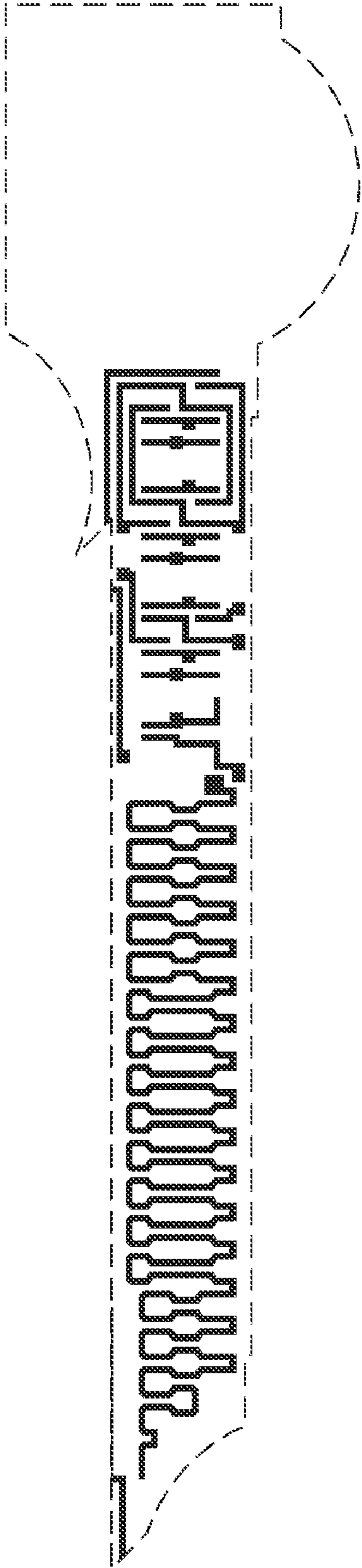
Poly mask
