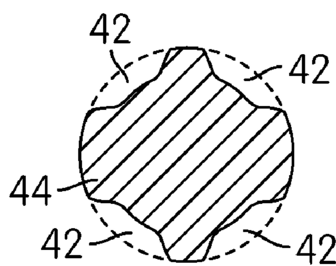
SECTION D-D
