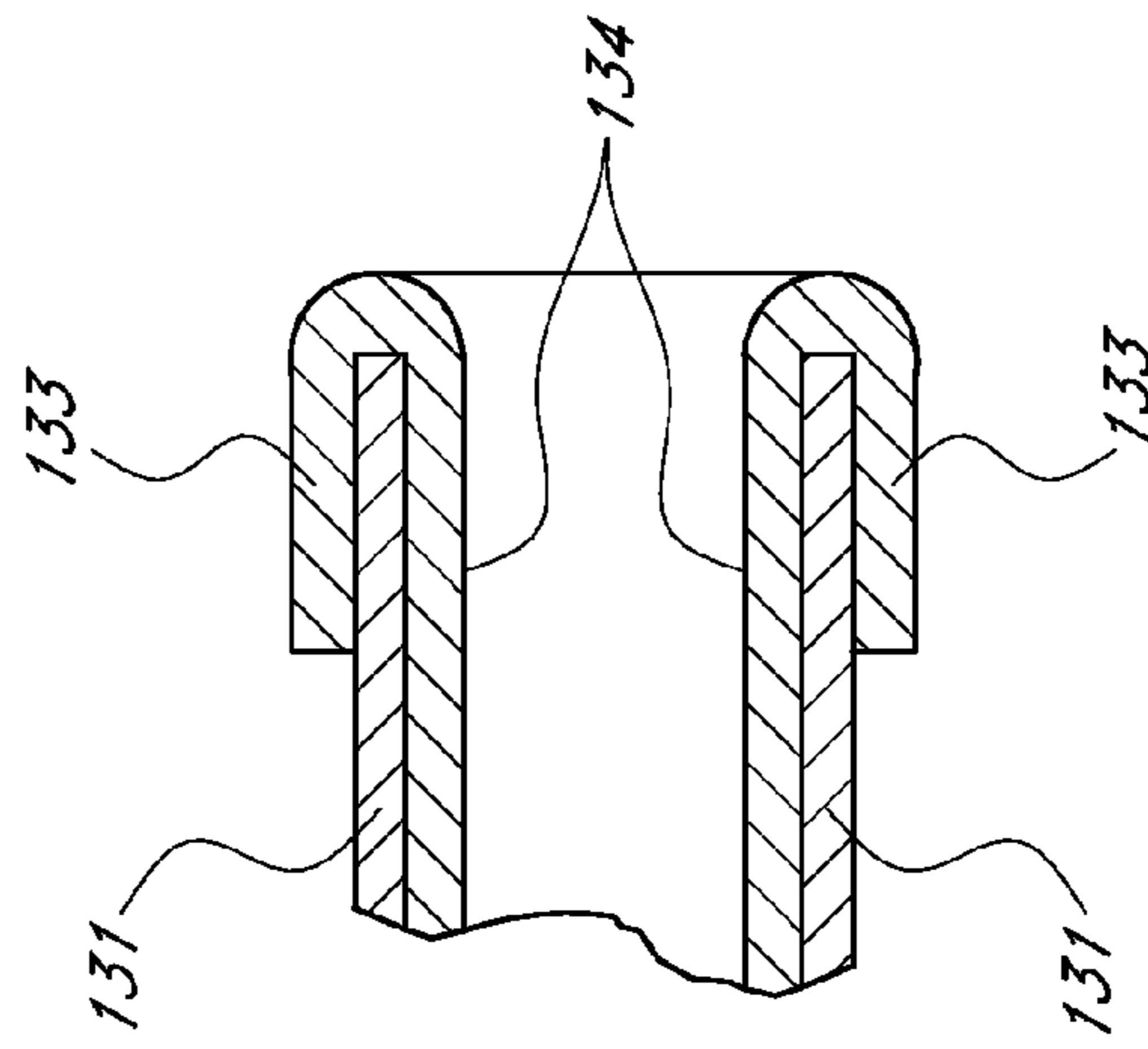
FIG. 10E
