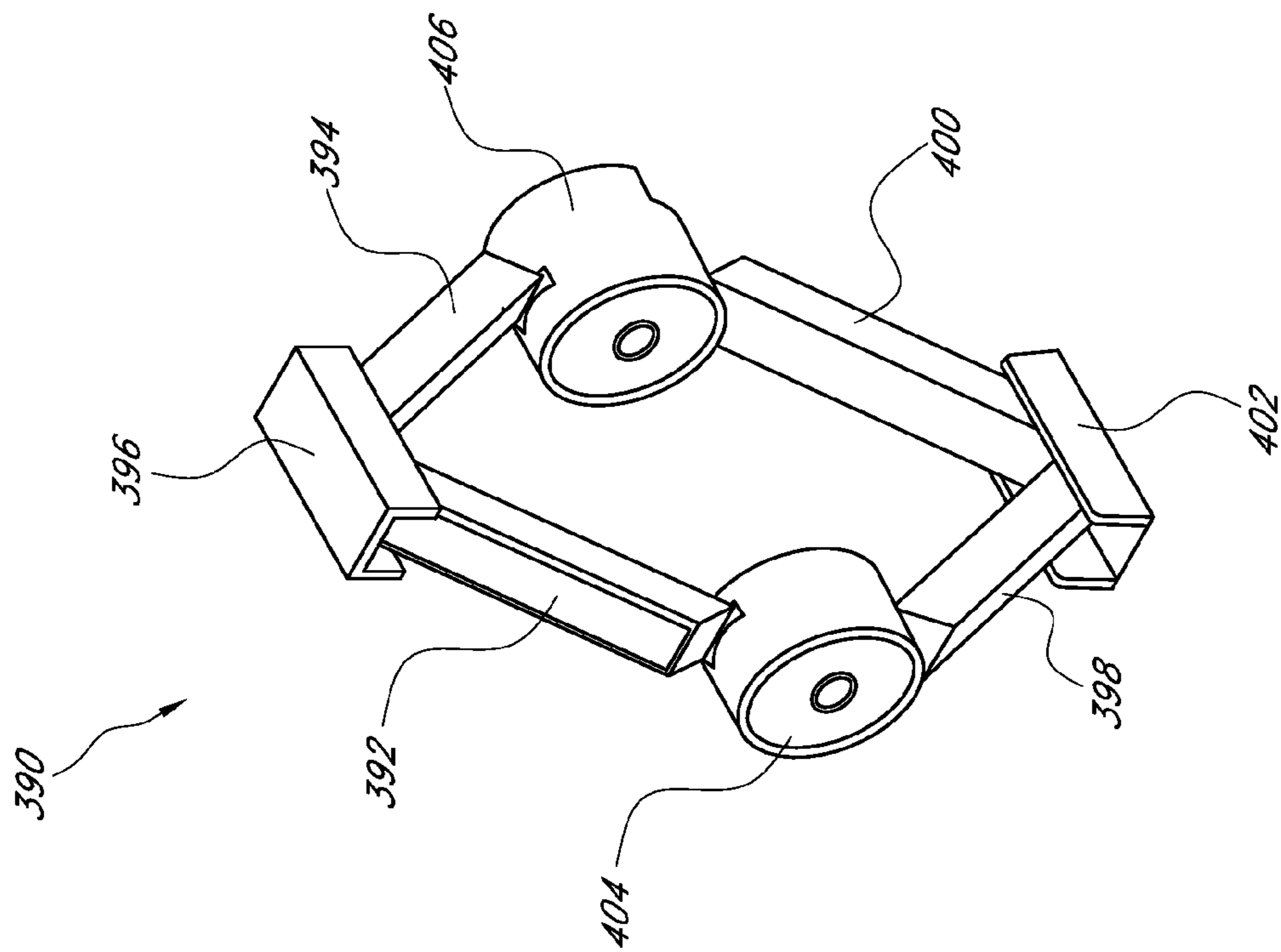
FIG. 28A
