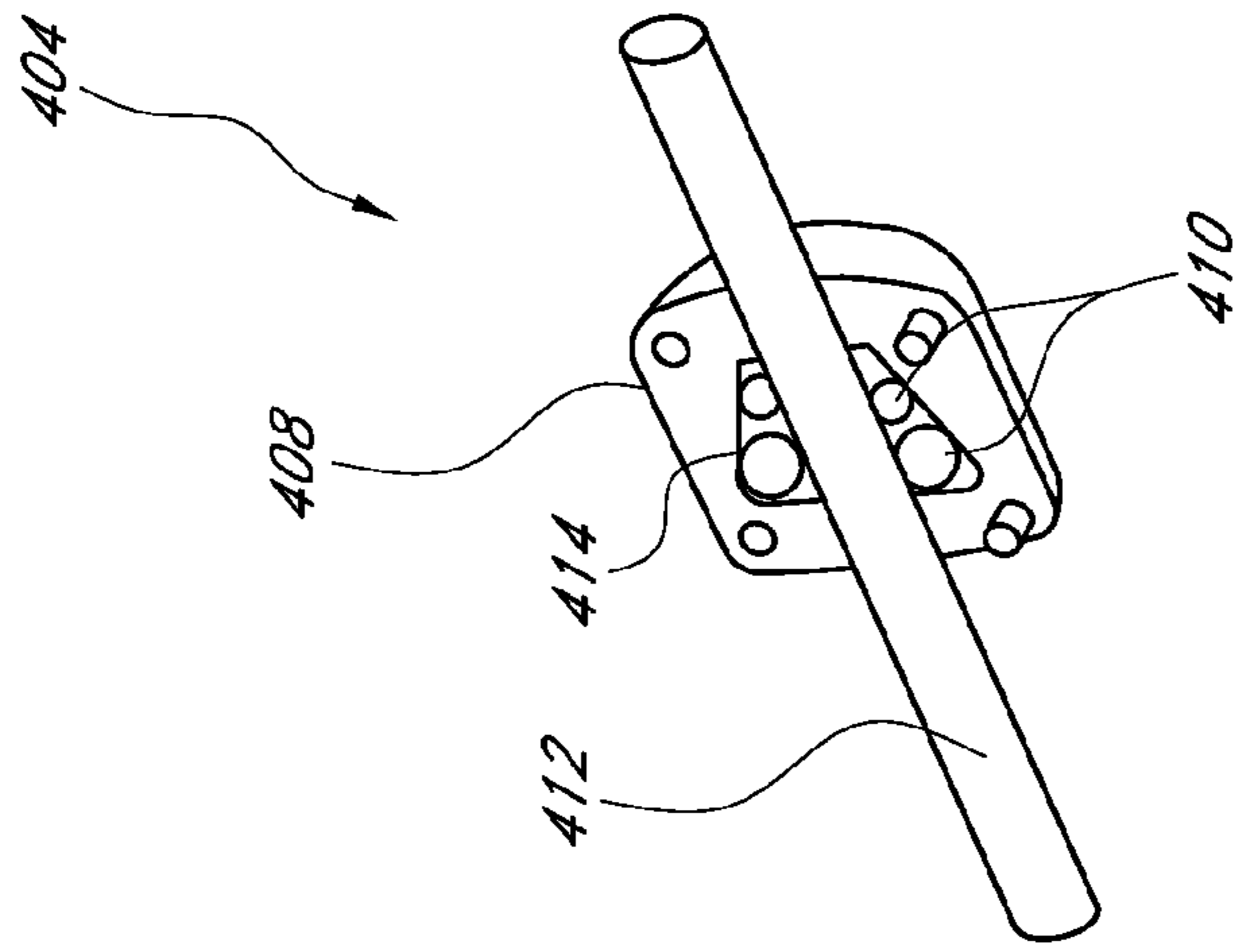
FIG. 28B
