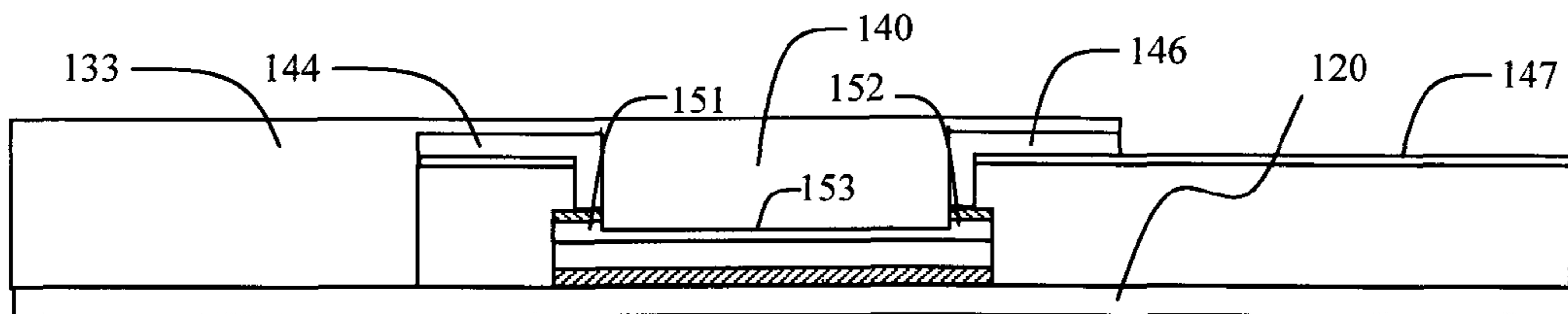
Fig. 6f
