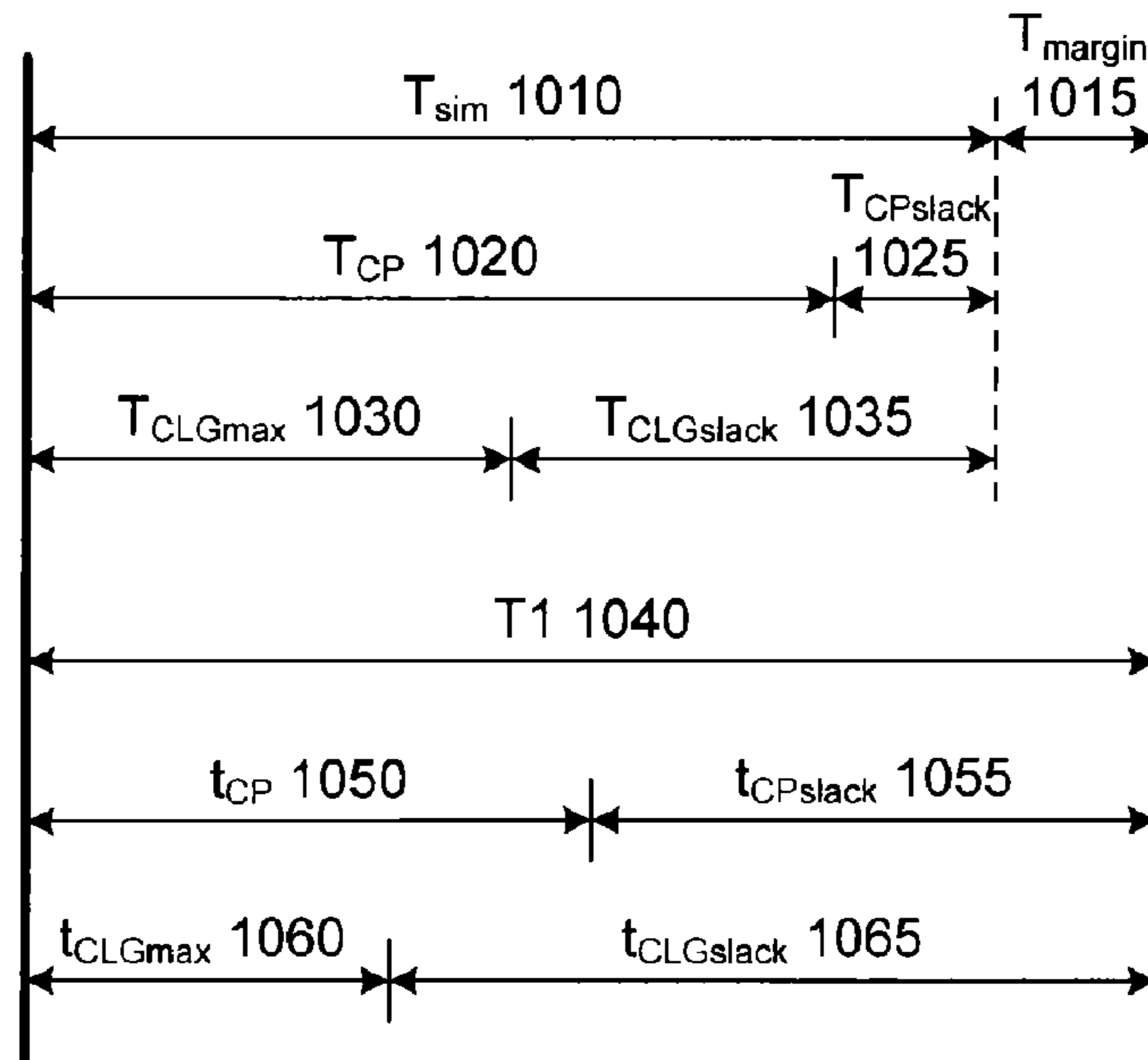
FIG. 10A
