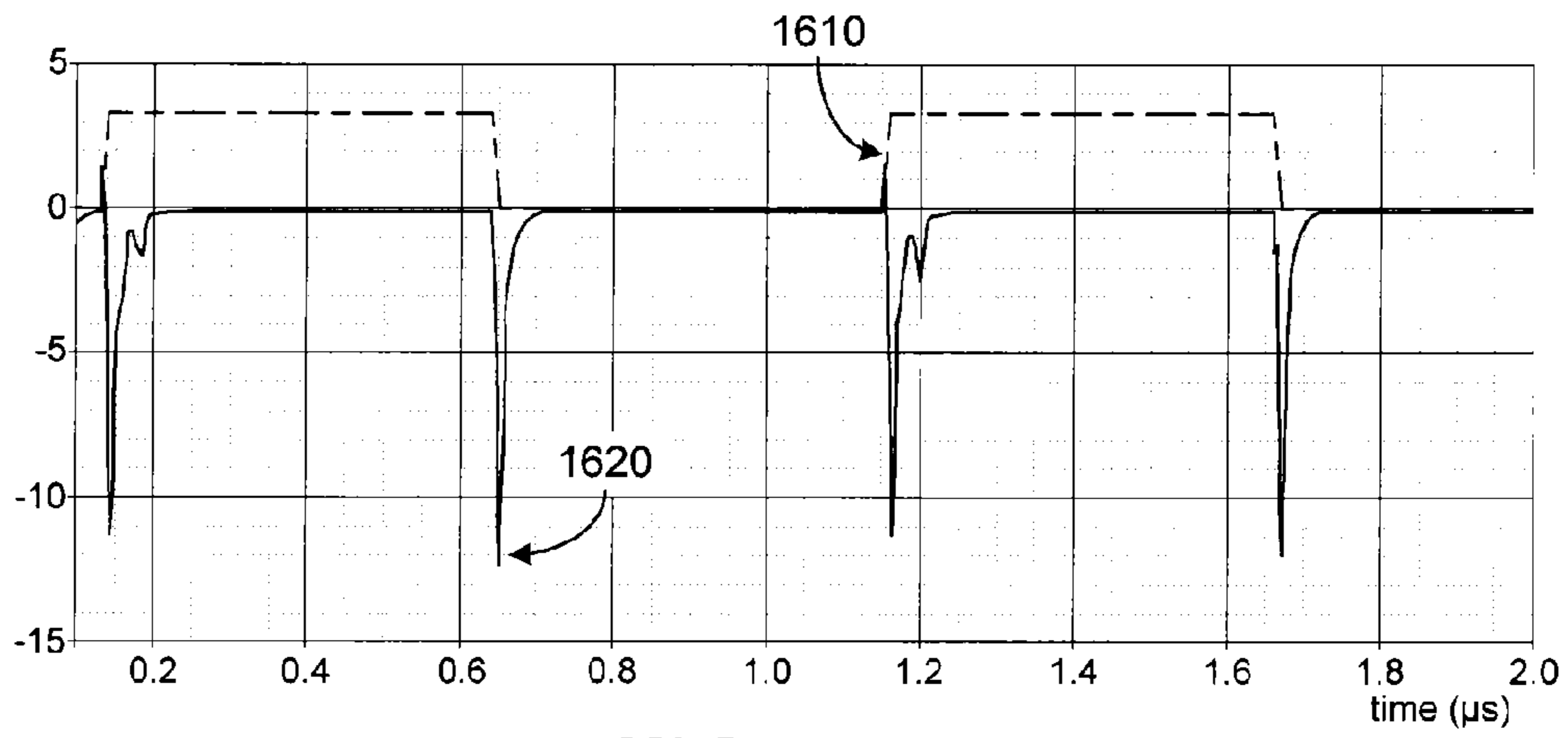
FIG. 16A
