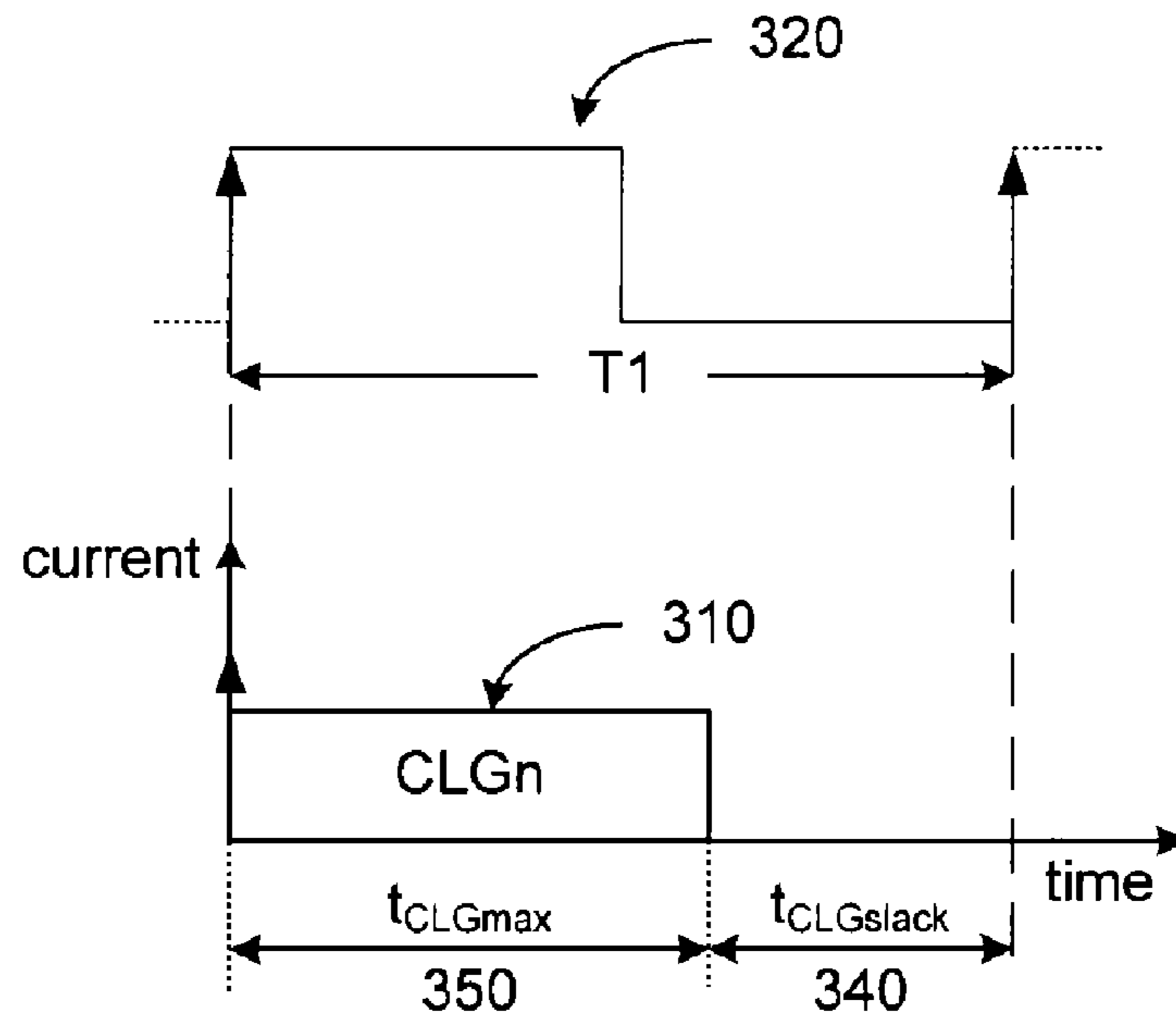
FIG. 3A
