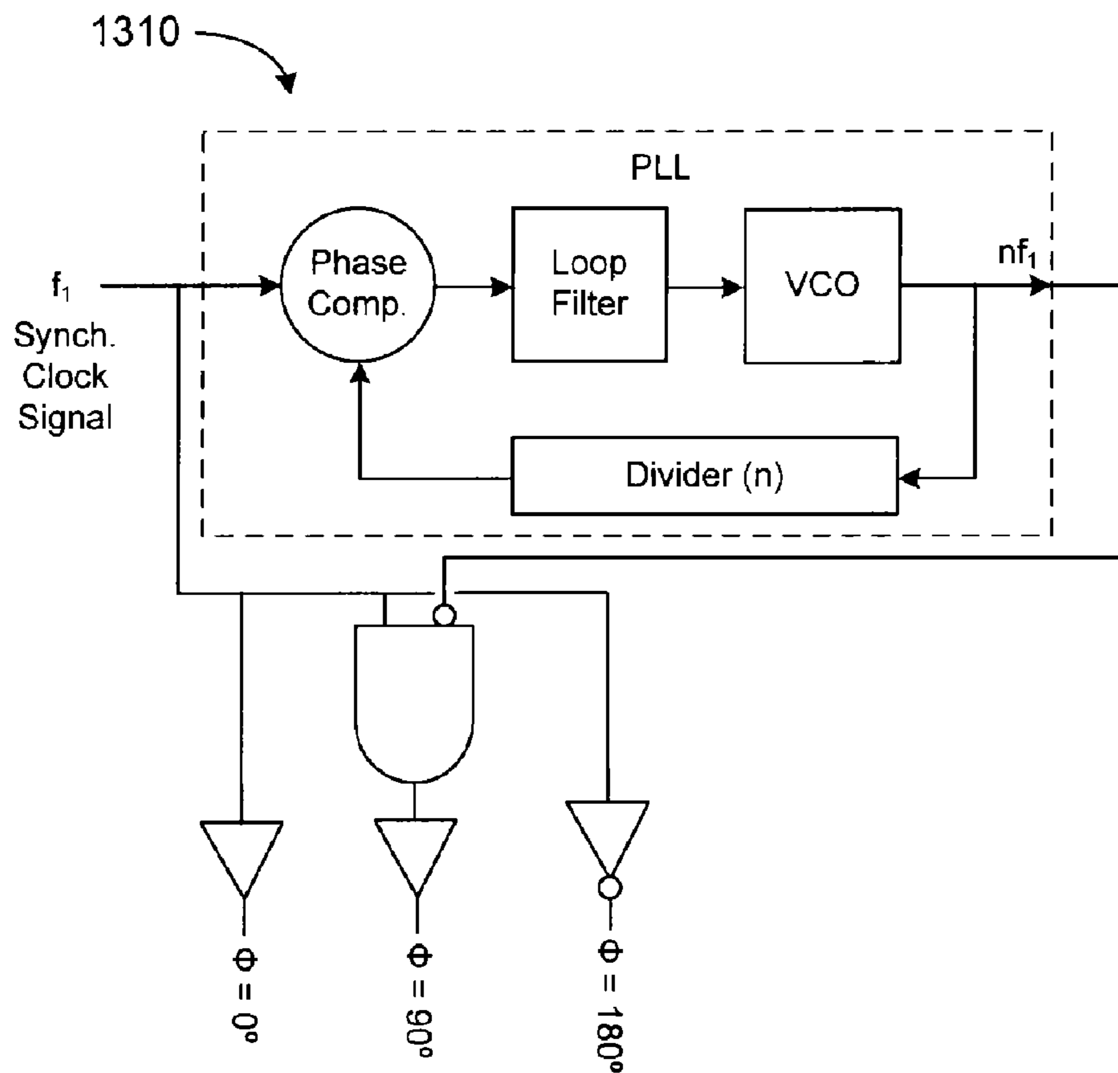
FIG. 13A
