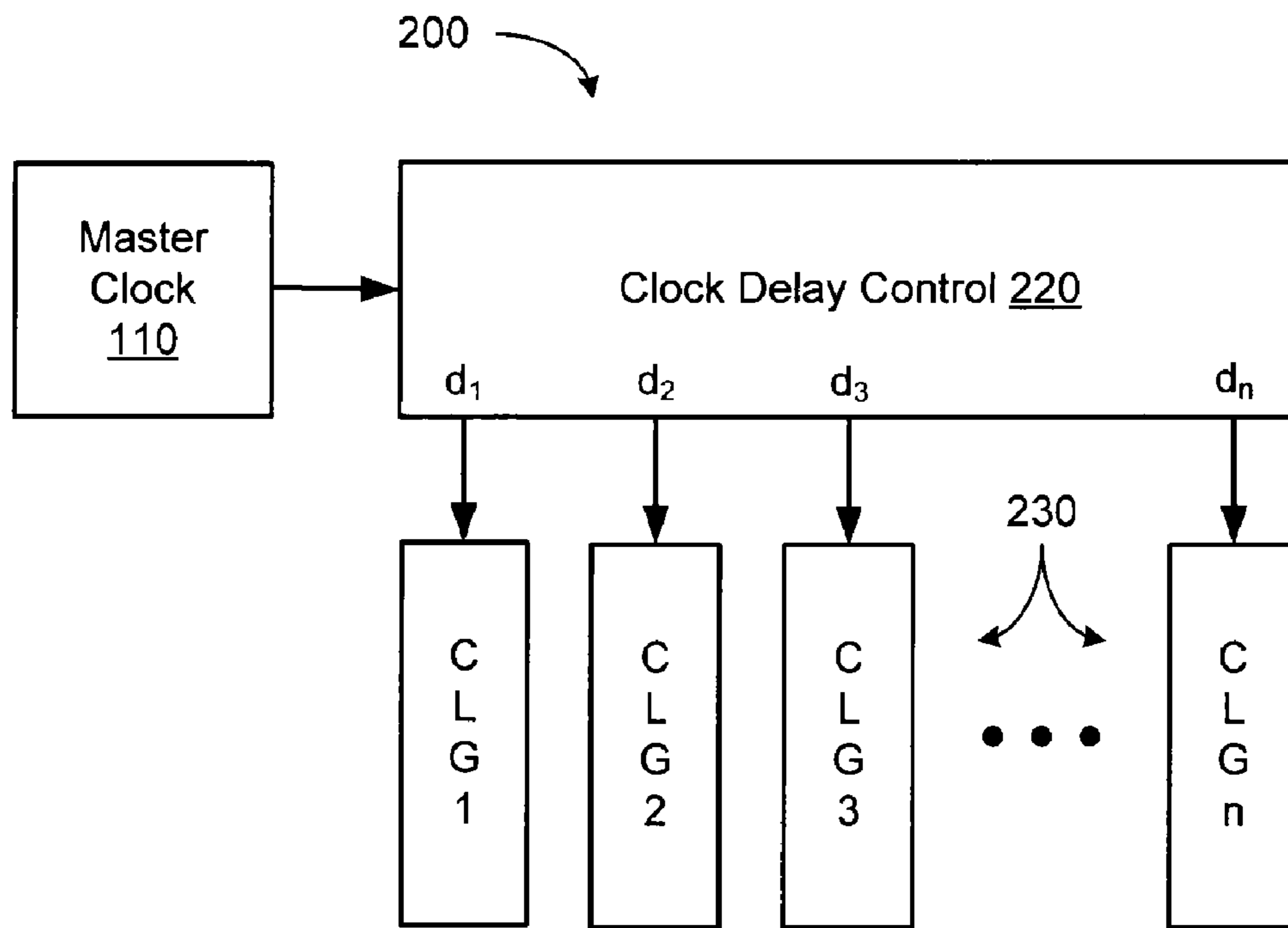
FIG. 2A
