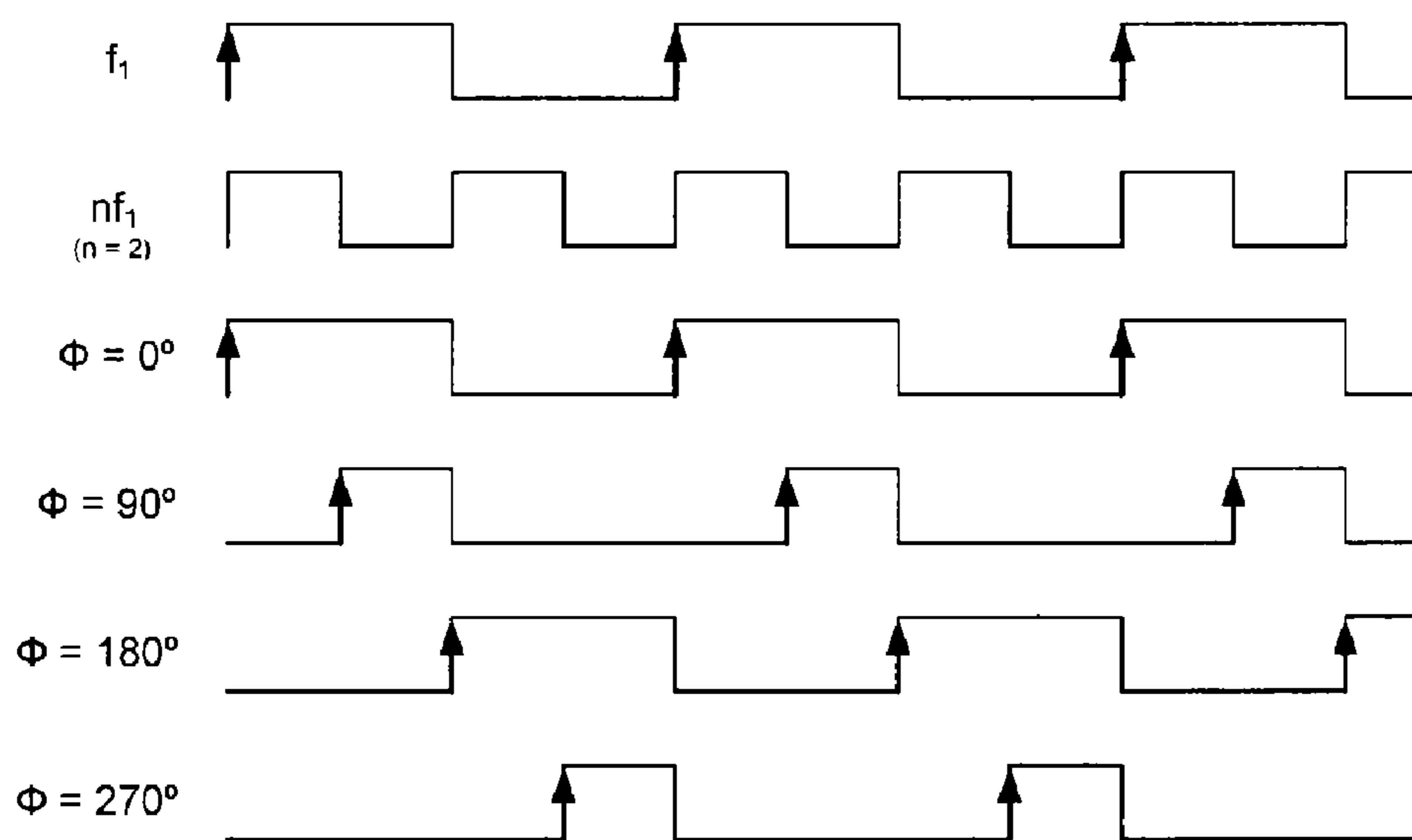
FIG. 14B
