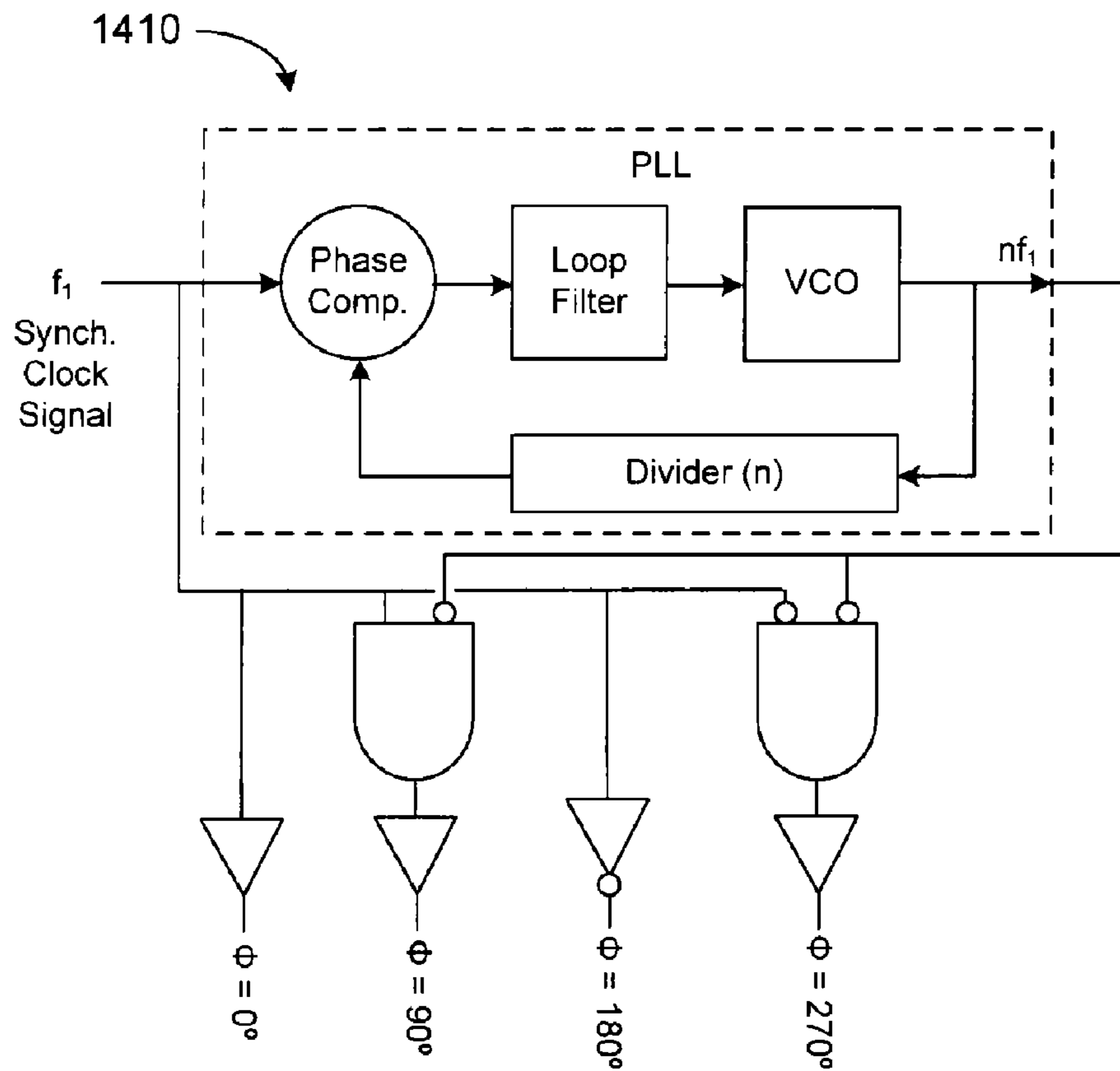
FIG. 14A
