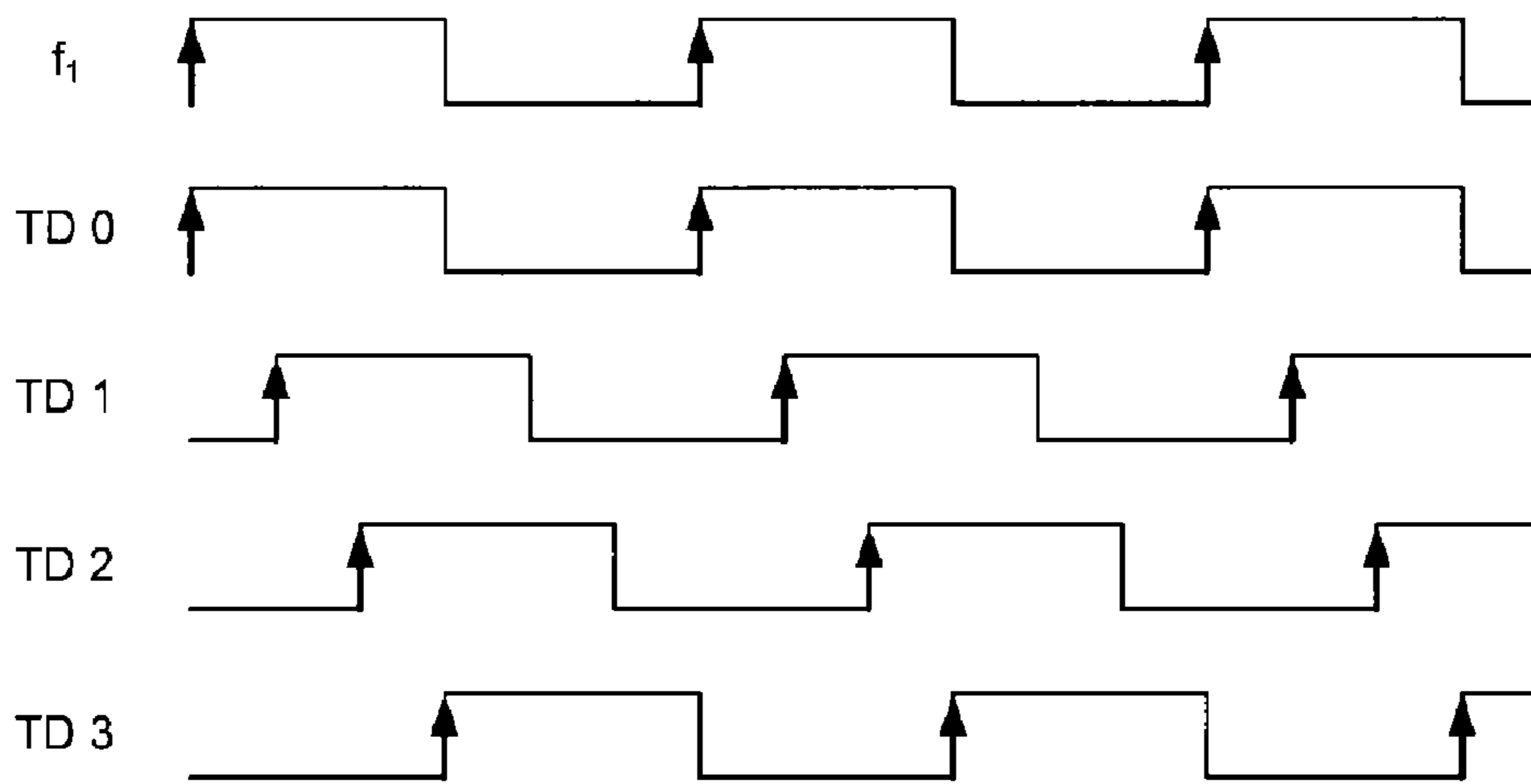
FIG. 15B
