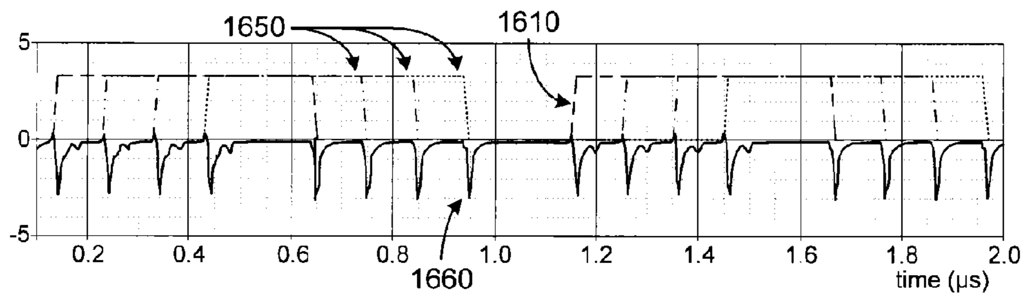
FIG. 16C
