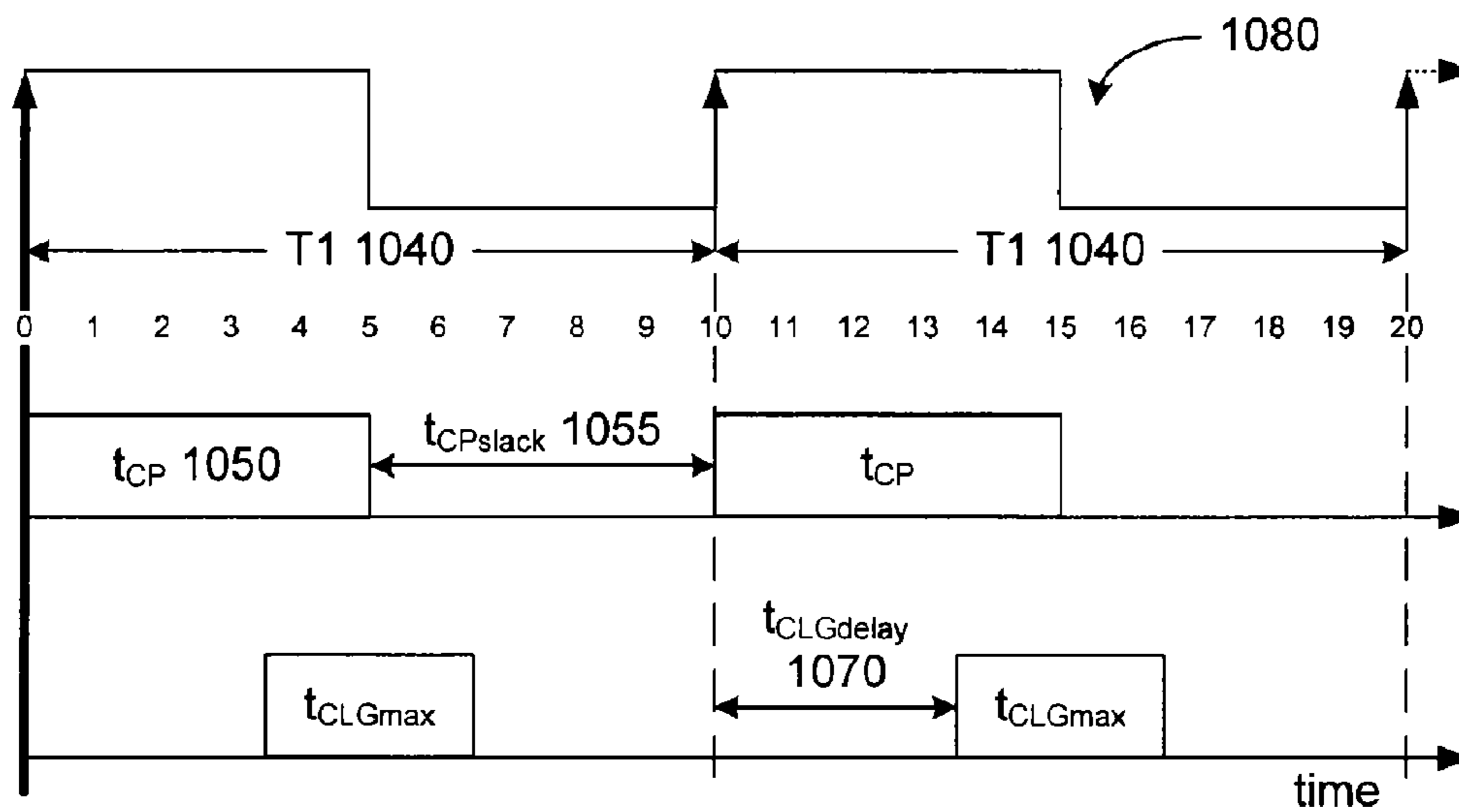
FIG. 10B
