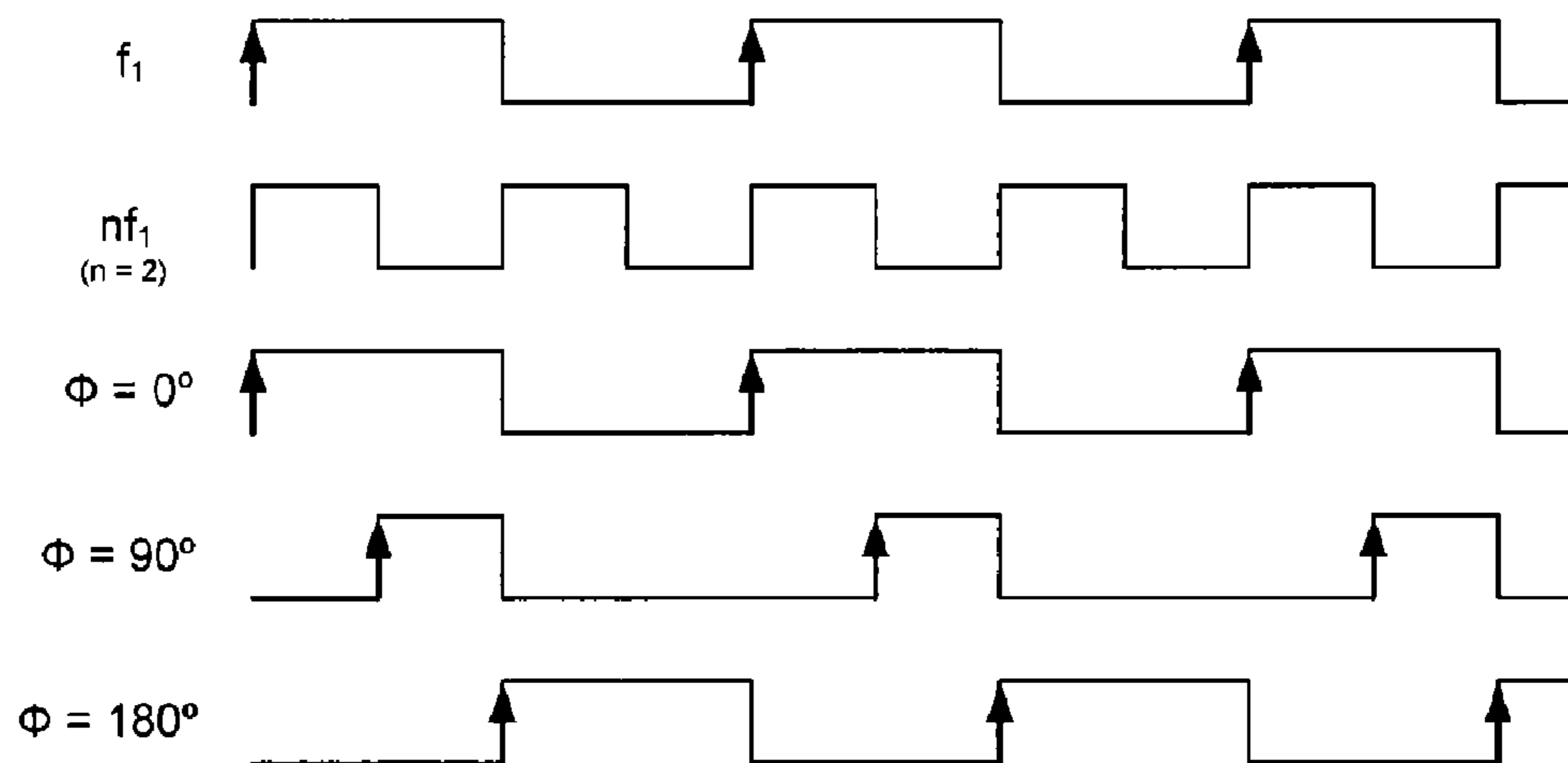
FIG. 13B
