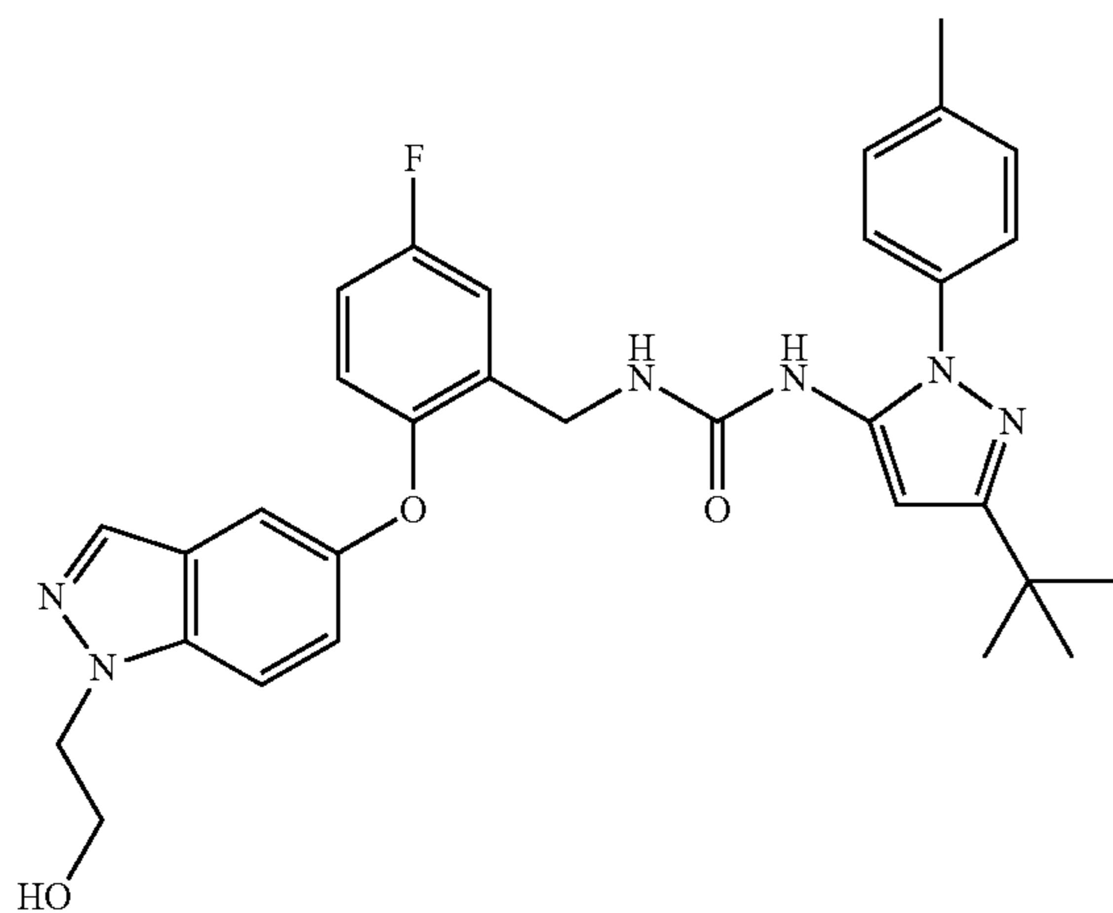
1-(3-tert-butyl-1-p-tolyl-1H-pyrazol-5-yl)-3-(5-fluoro-2-(1-(2-hydroxyethyl)-1H-indazol-5-yloxy)benzyl)urea (72)
