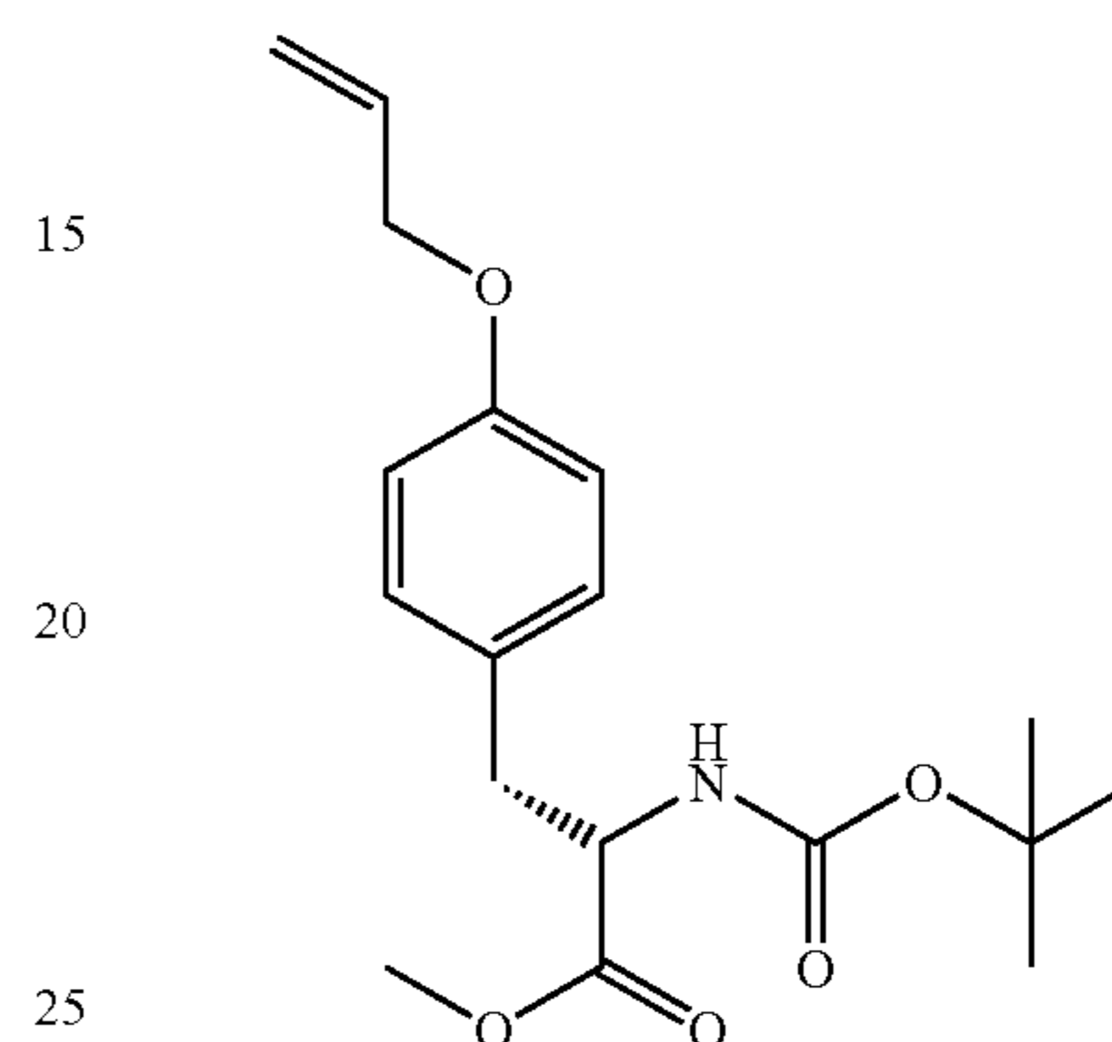
Methyl(2S)-3-(4-allyloxyphenyl)-2-tert-butoxycarboxamidopropanoate (59)
