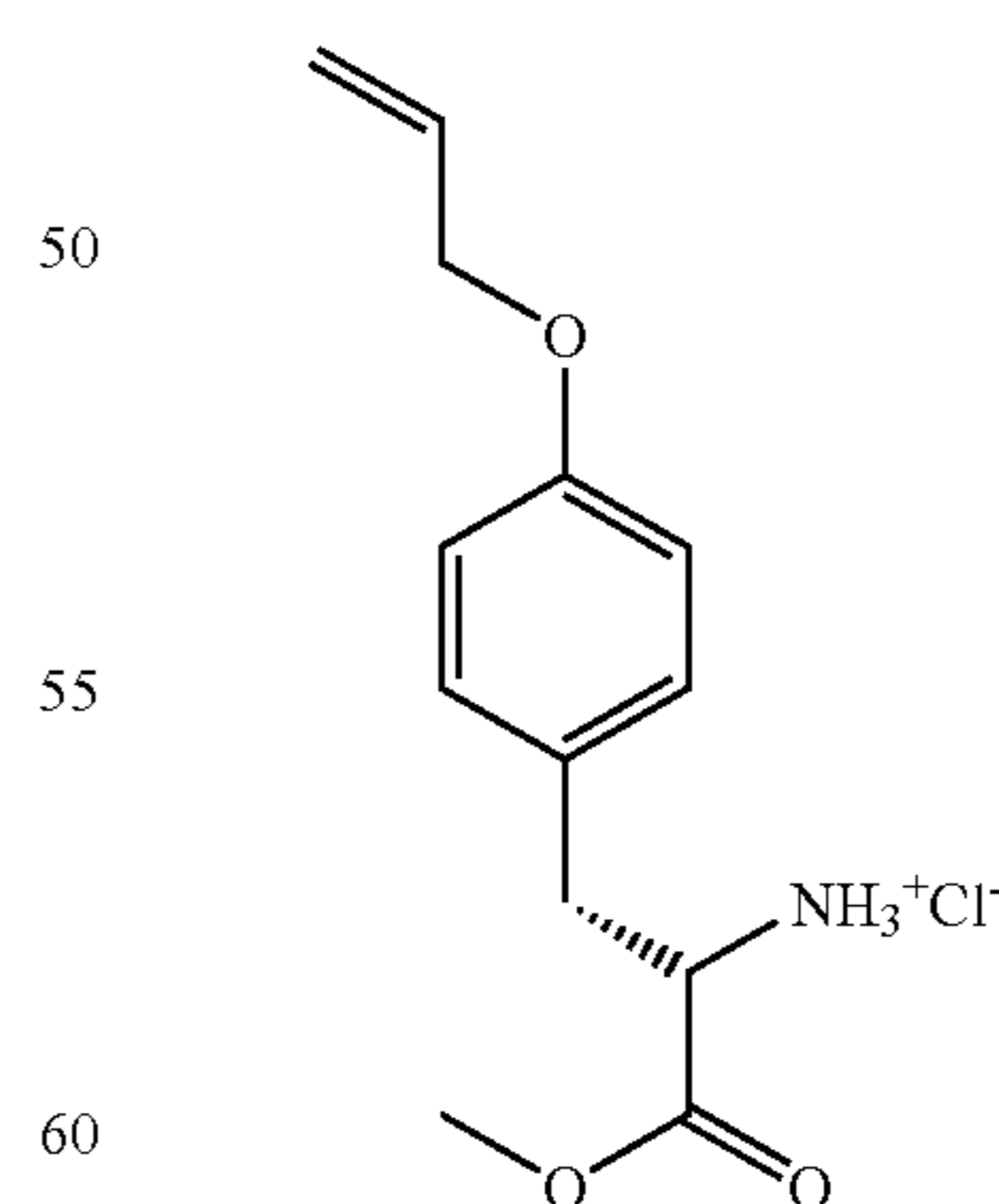
Methyl(2S)-2-(4-allyloxyphenyl)-2-aminopropanoate hydrochloride (60)
