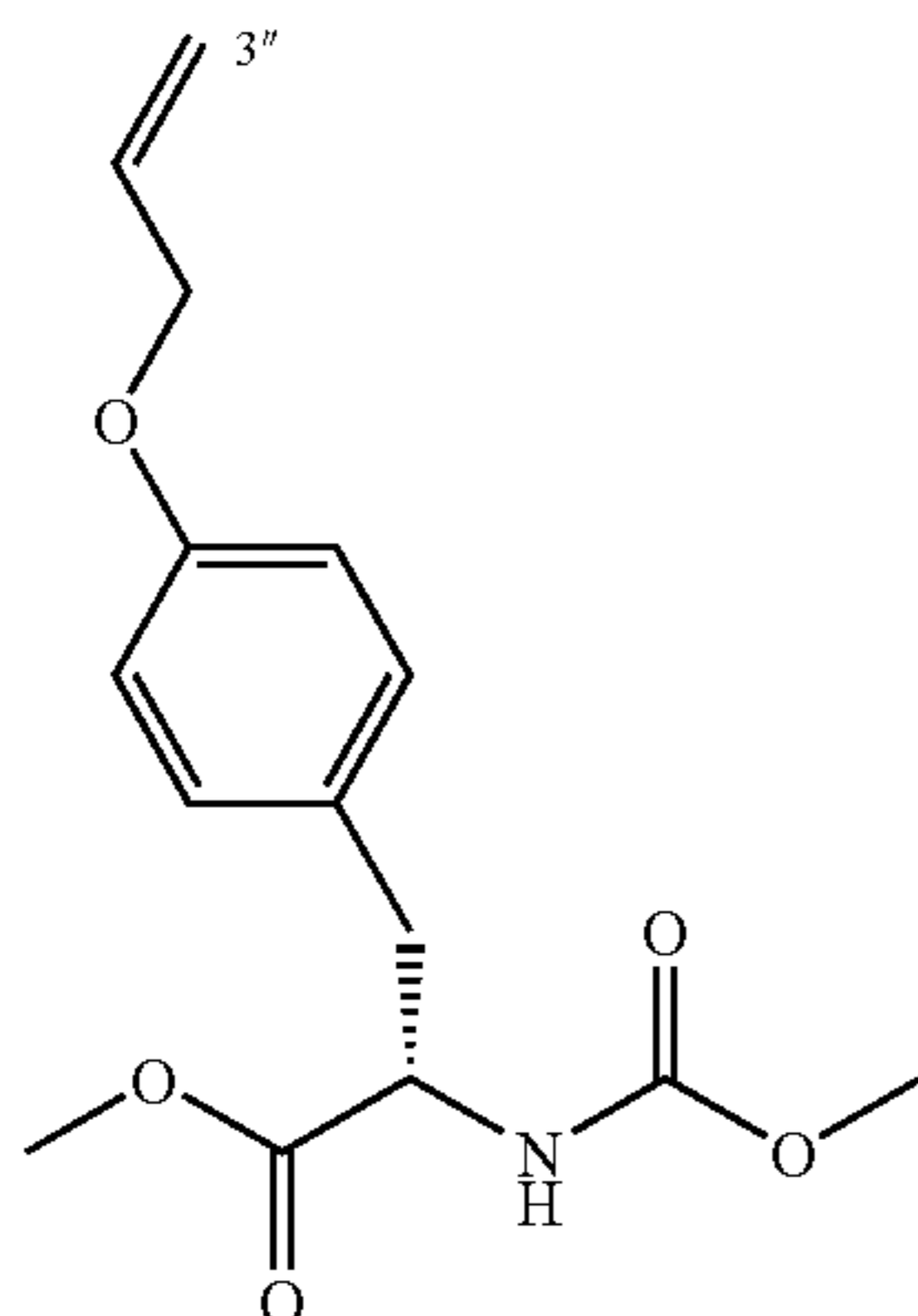
Methyl(2S)-3-(4-allyloxyphenyl)-2-methoxycarboxamidopropanoate (171)
