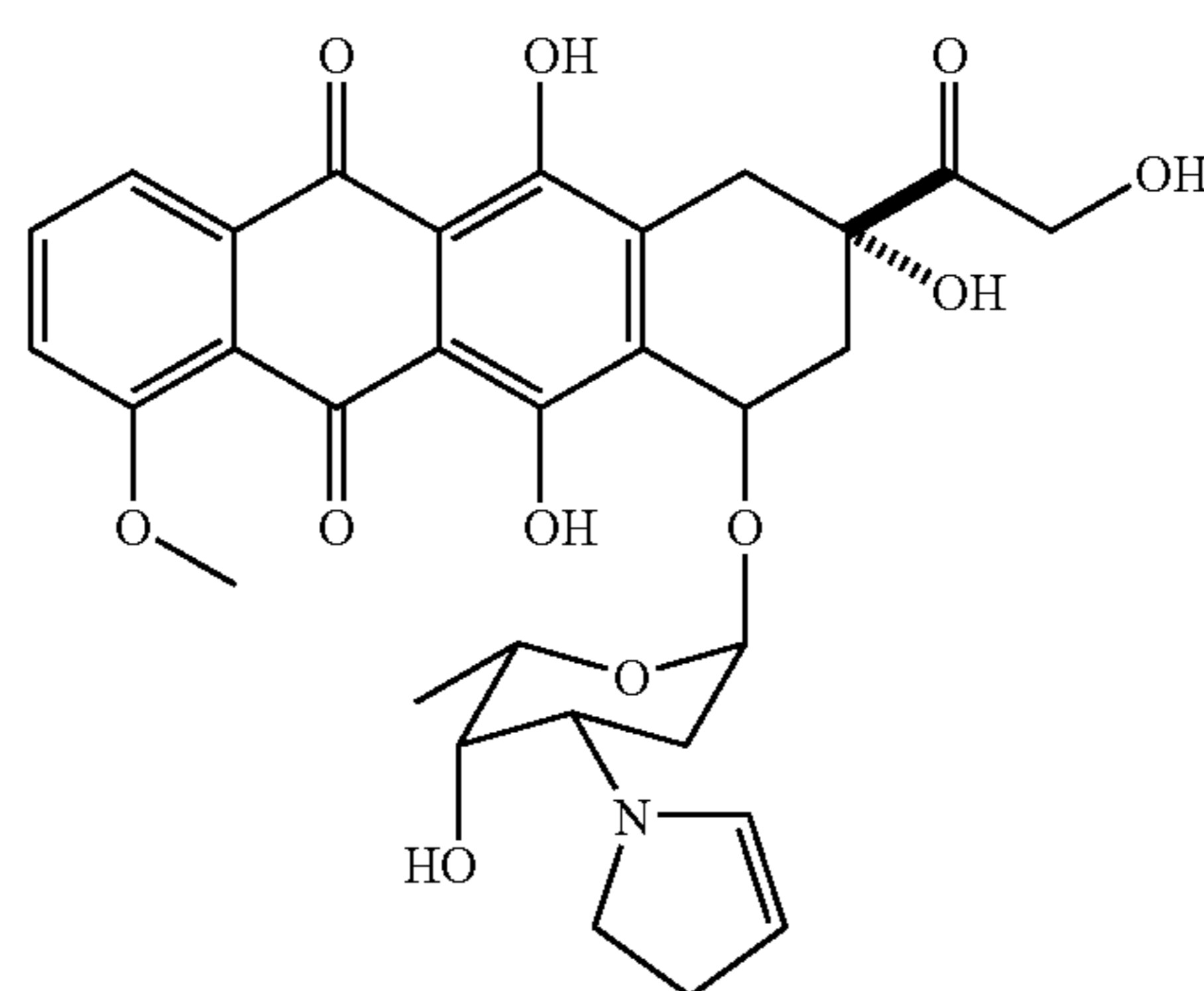
2-Pyrrolinodoxorubicin (4)
