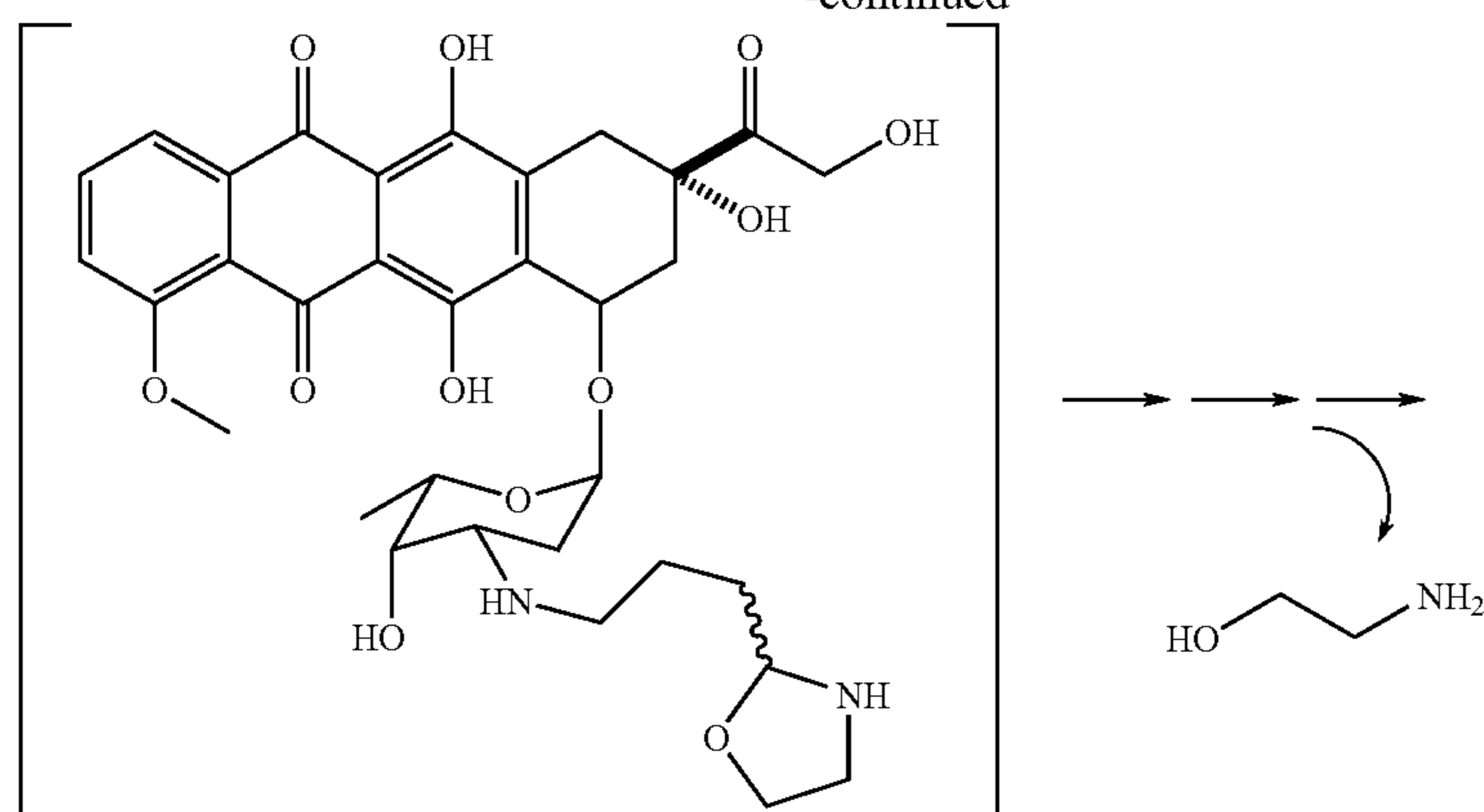
Doxorubicin propyl oxazolidine (DPO;2)
