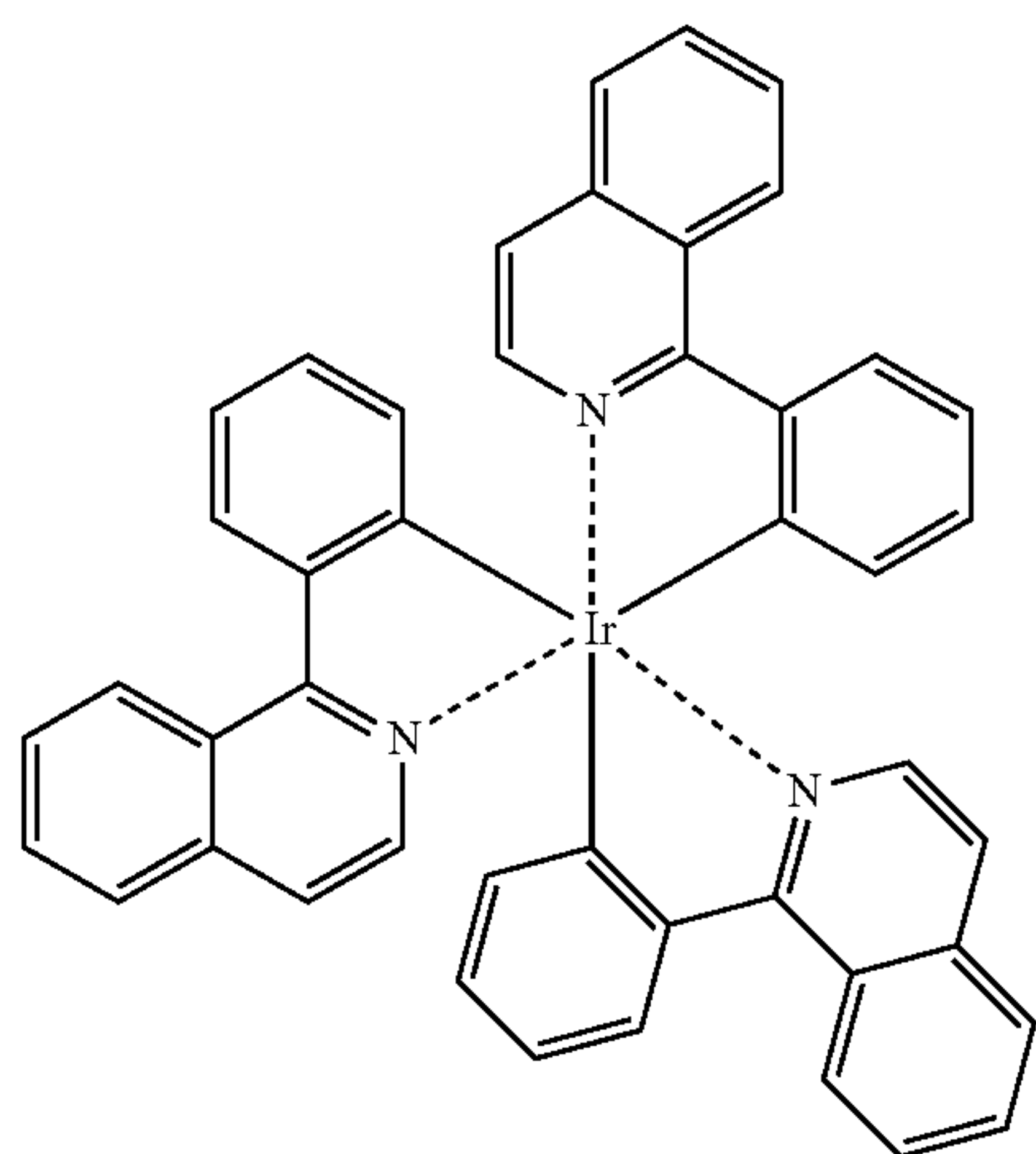
Ir(piq) 3
