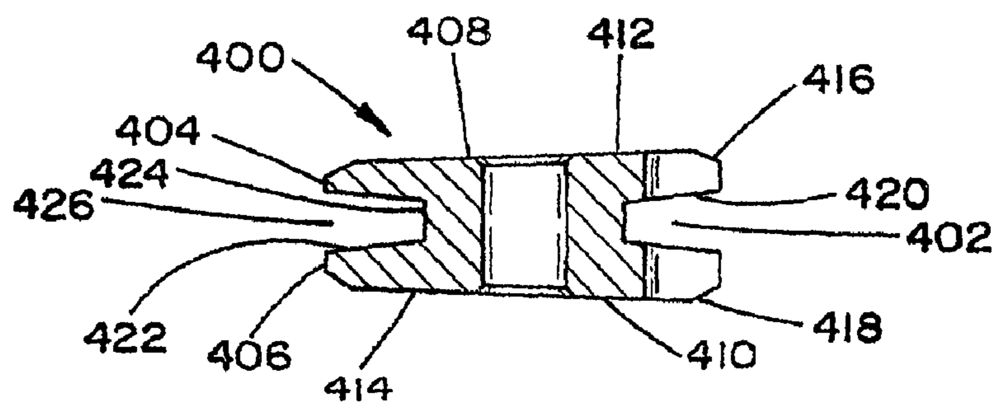
Section A-A
