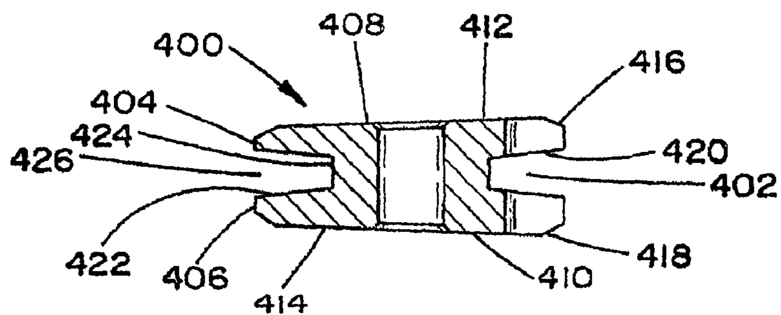
Section A-A
