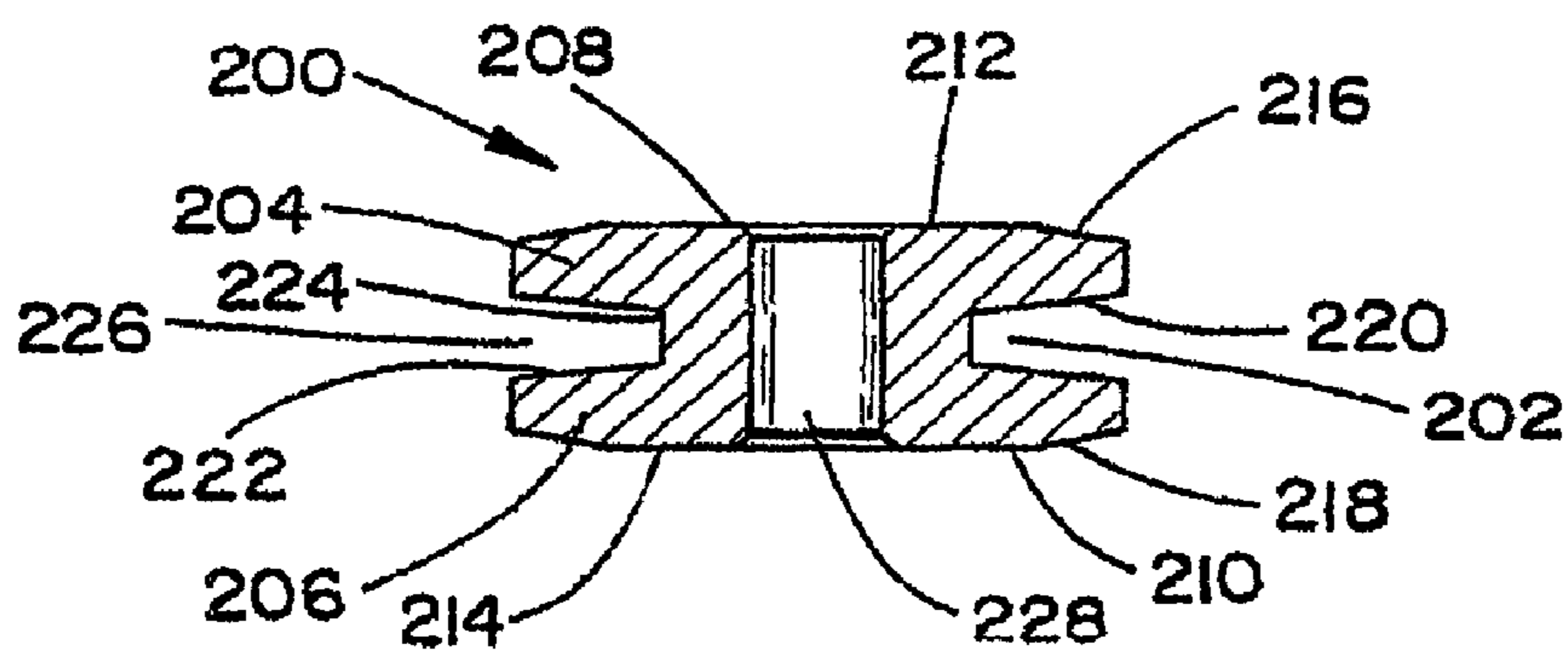
Section A-A
