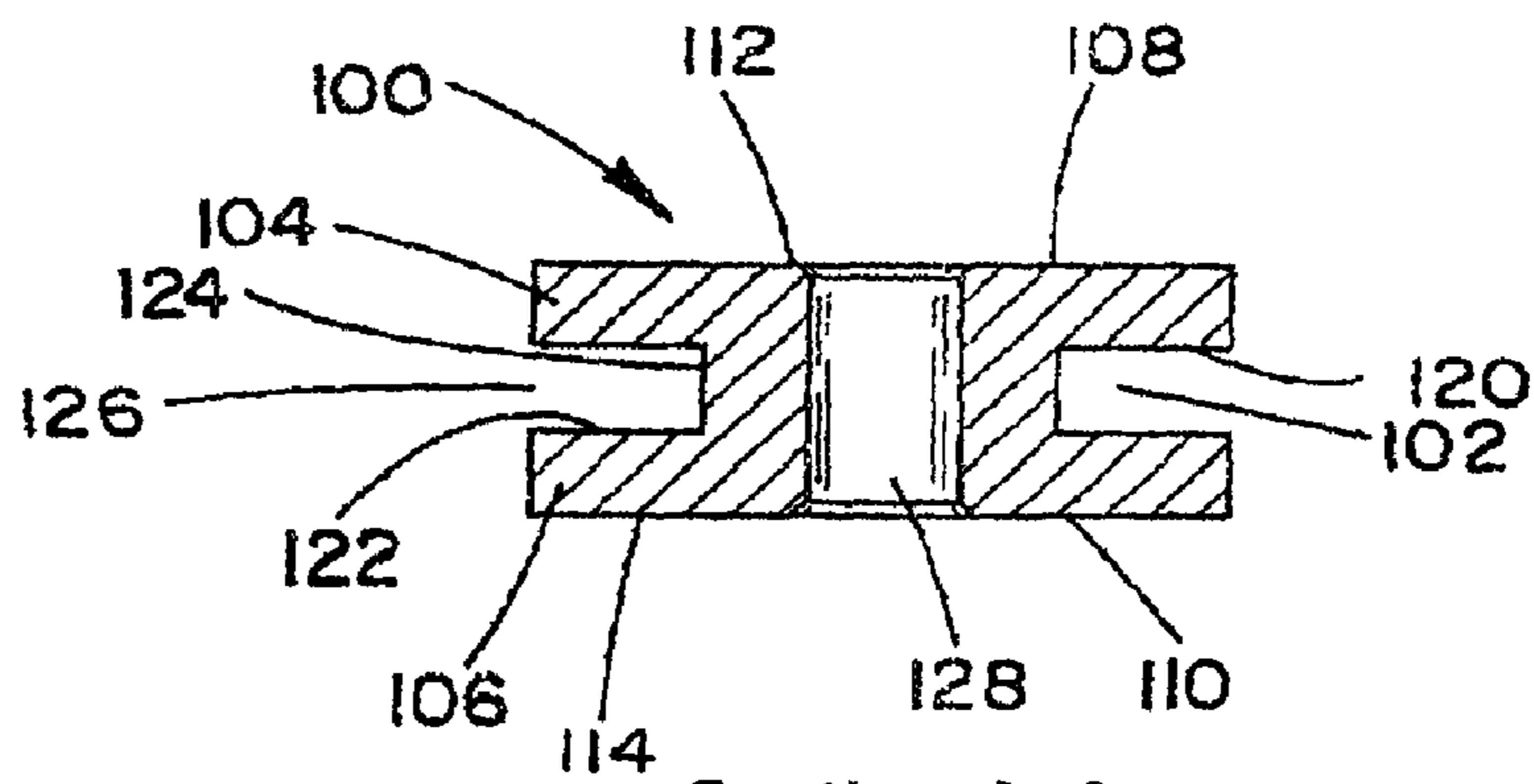
Section A-A FIG. 1c
