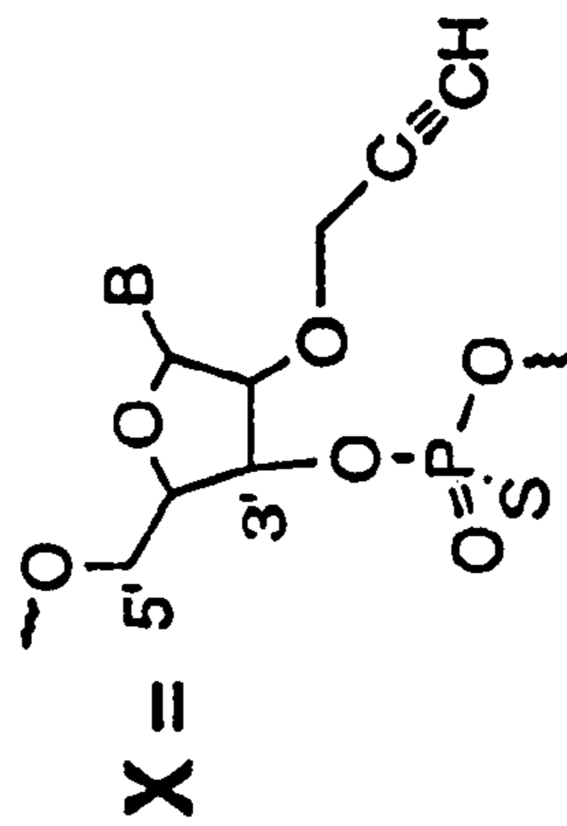
2'-O-Propargyl-ribonucleoside
