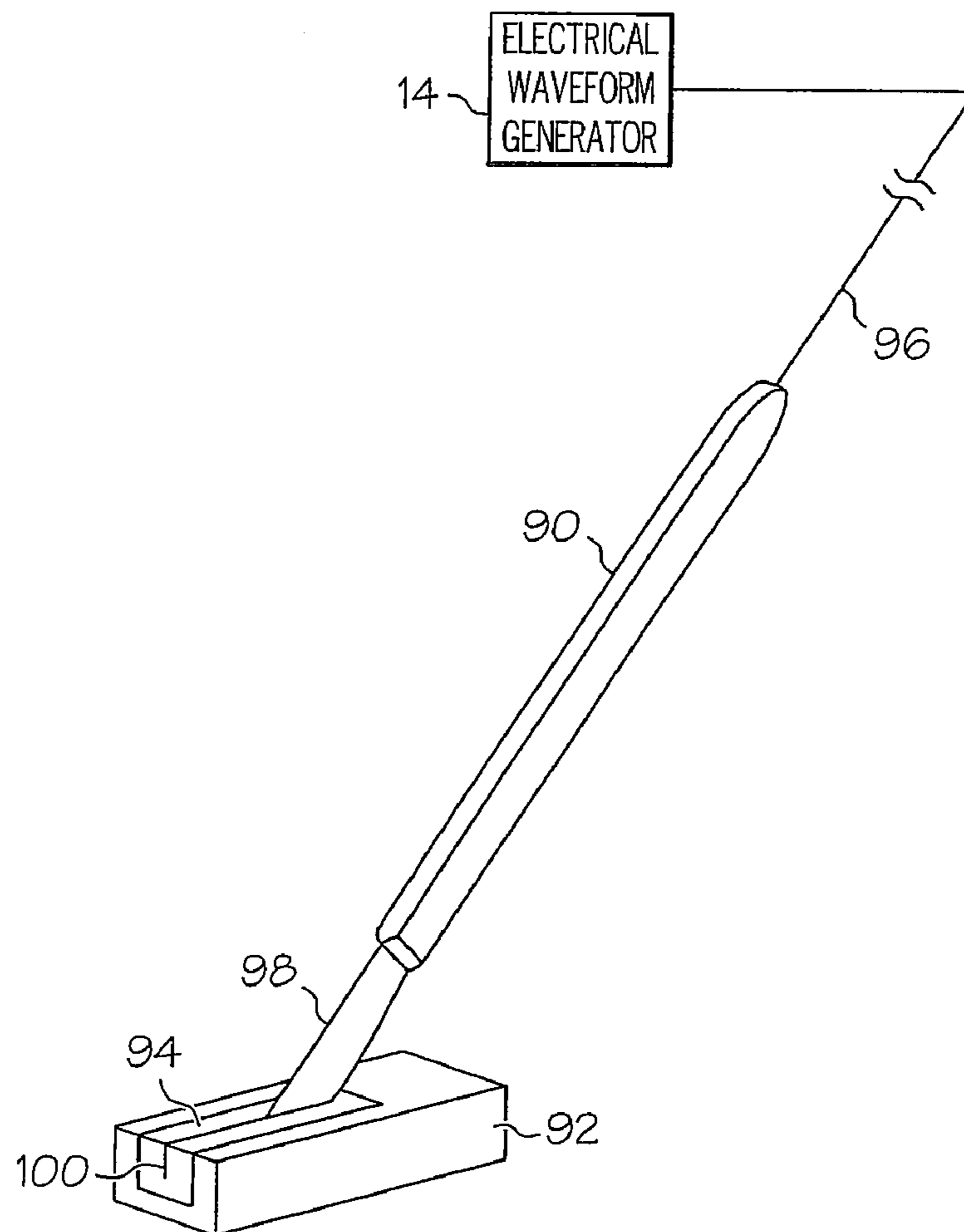
FIG. 13
