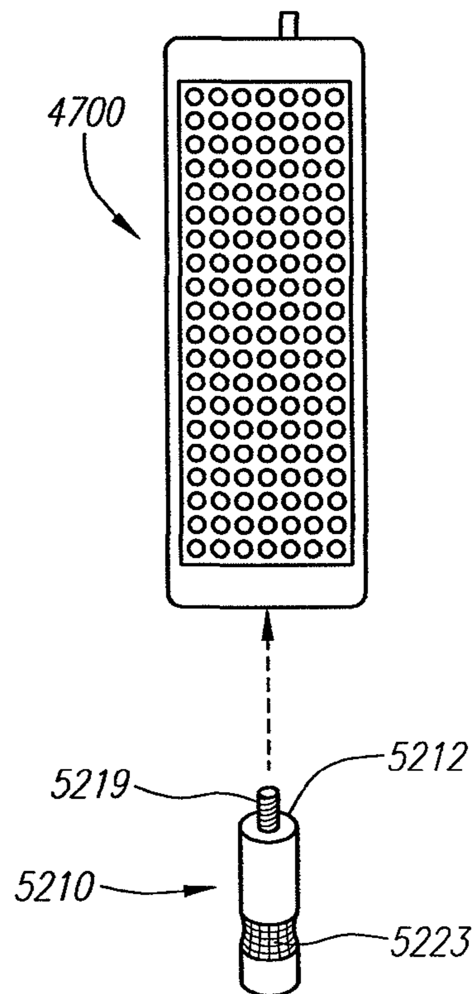
FIG. 52C
