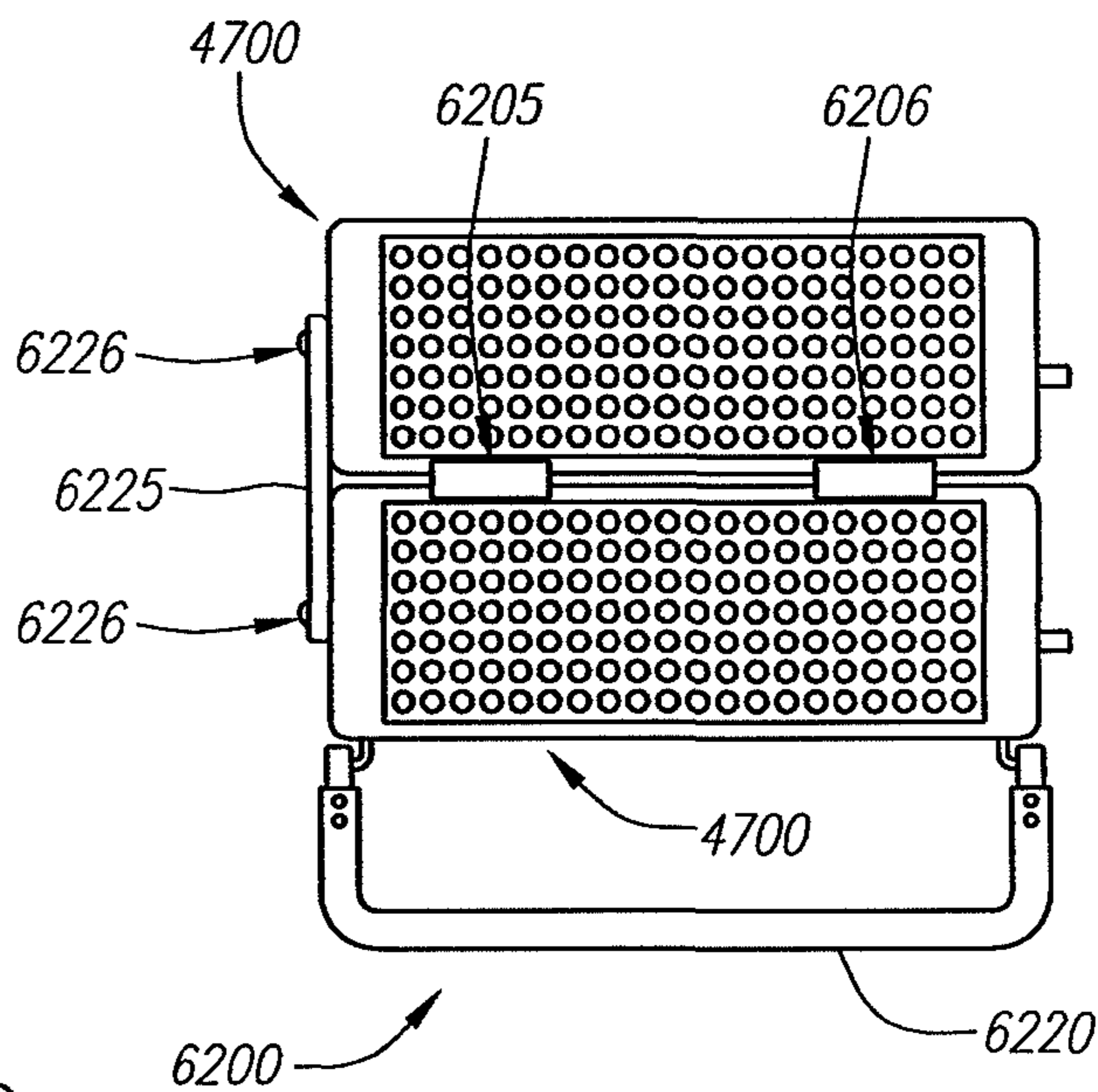
FIG. 62
