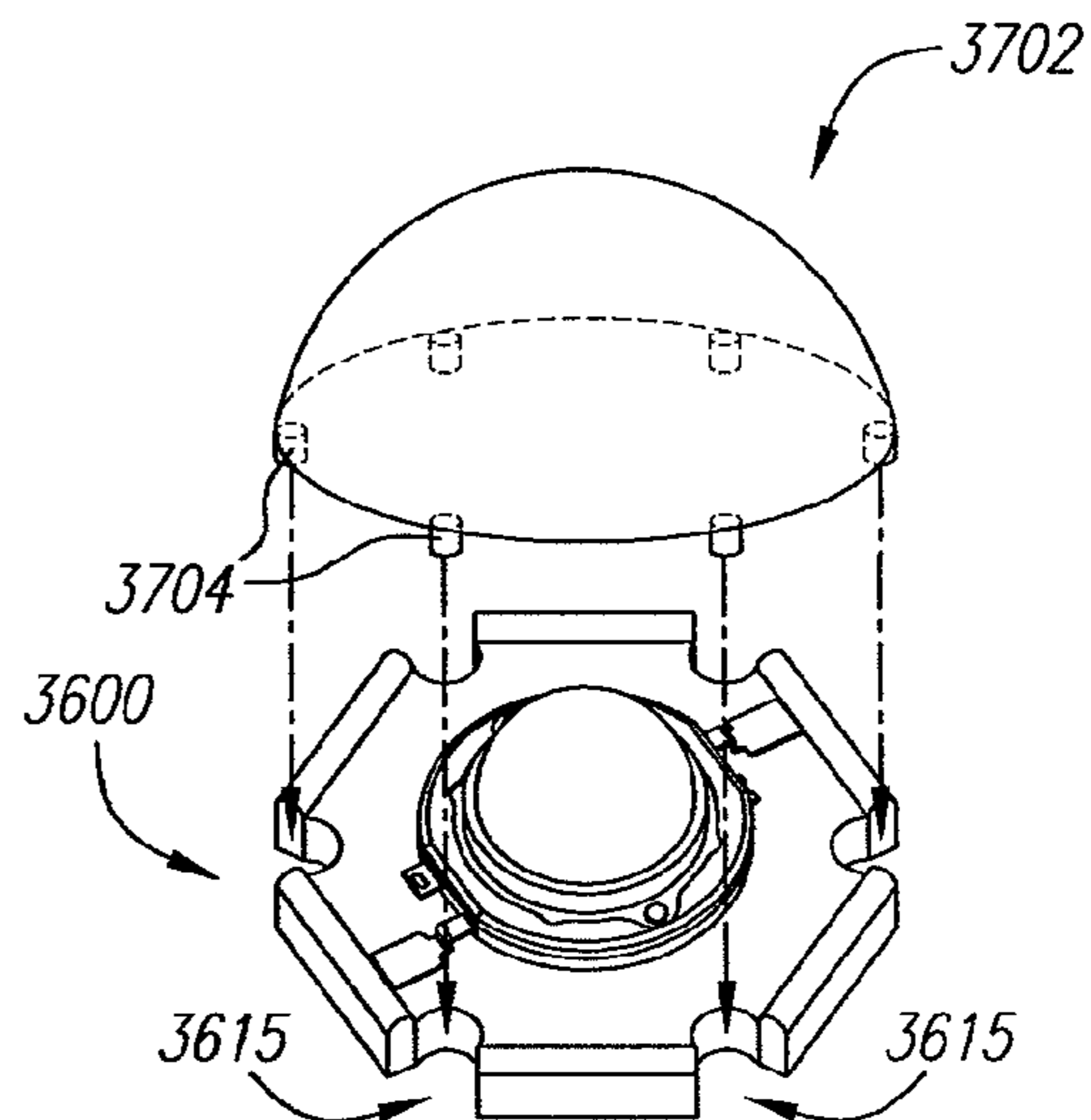
FIG. 37B
