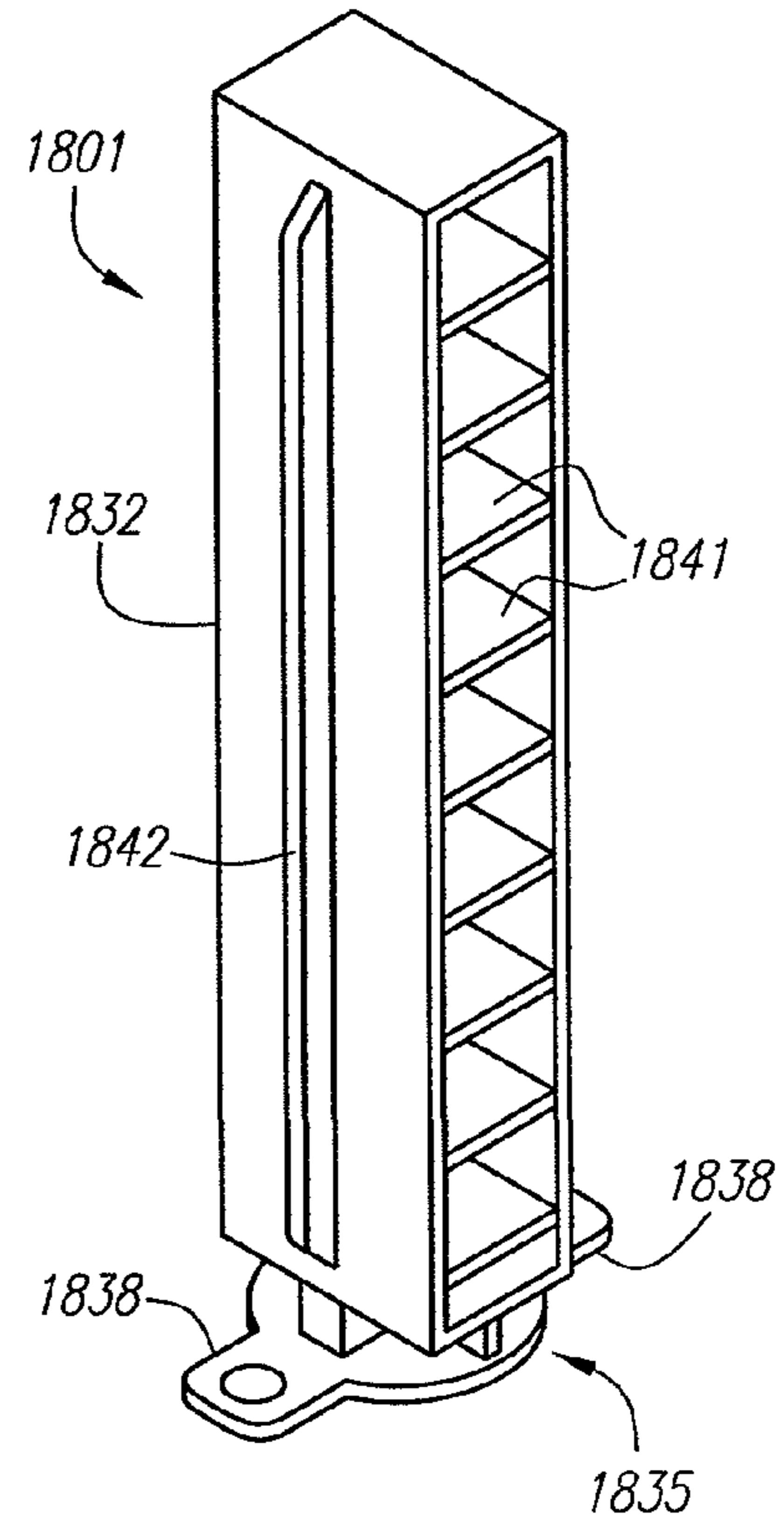
FIG. 18
