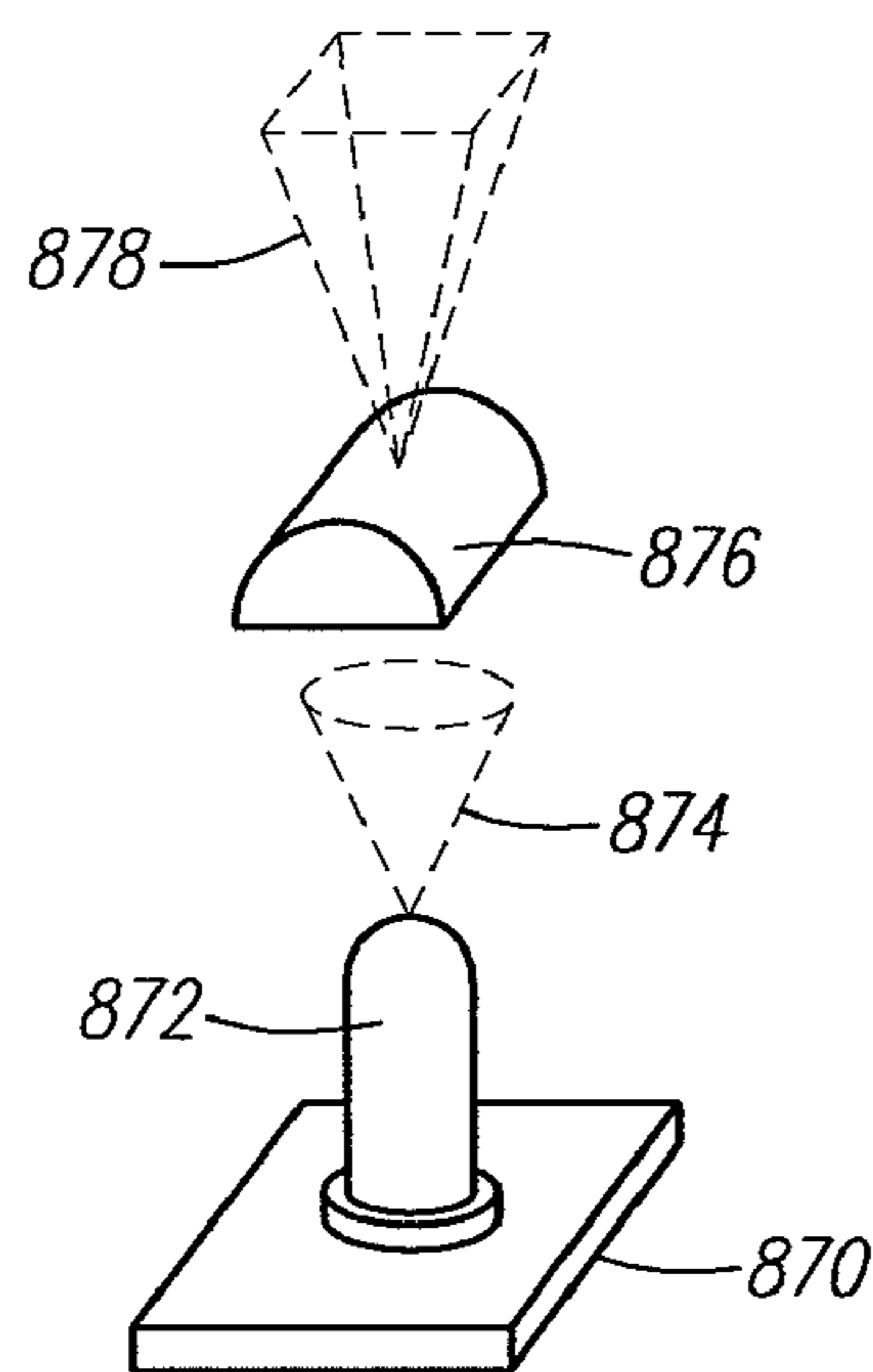
FIG. 8
