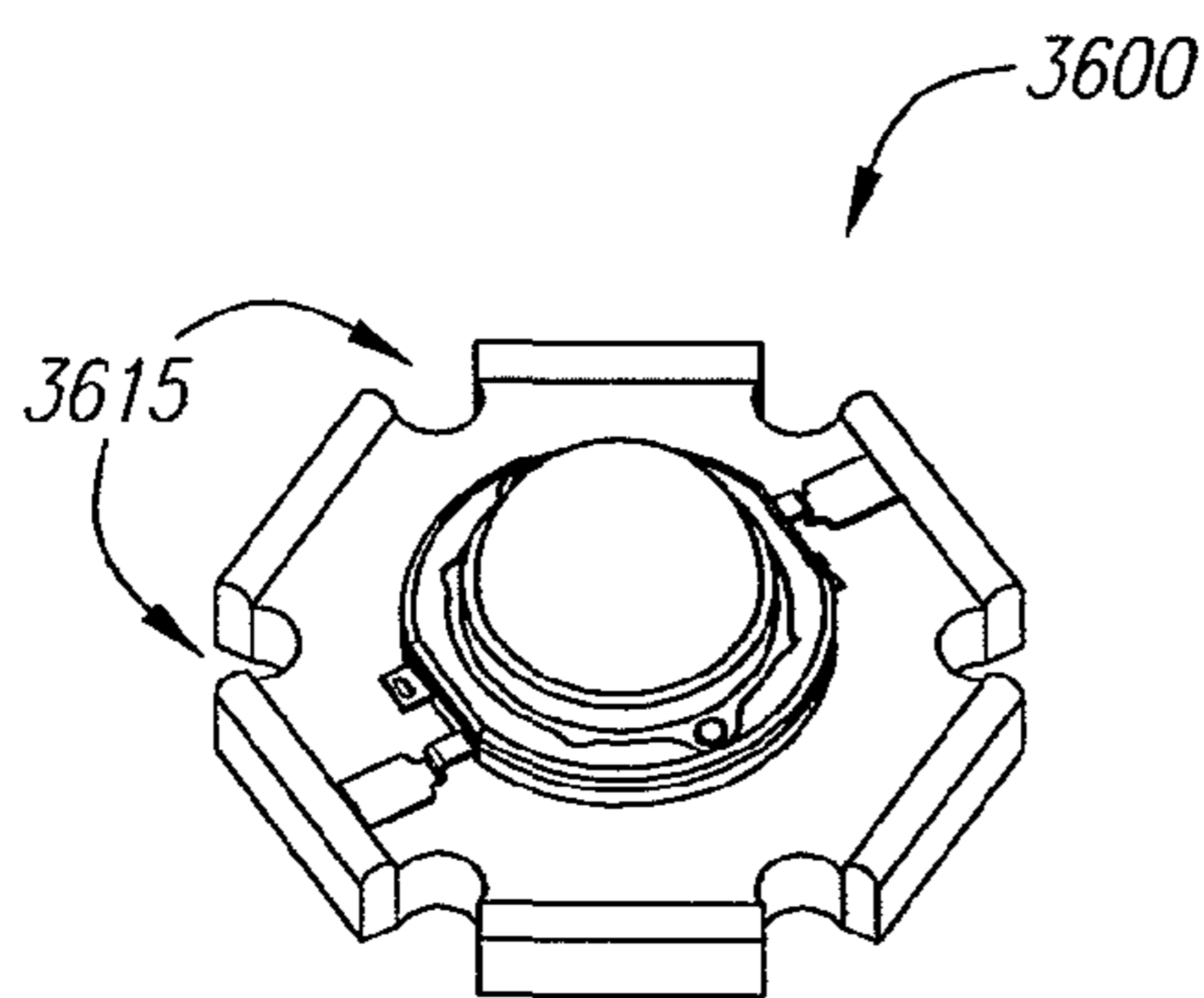
FIG. 36C
