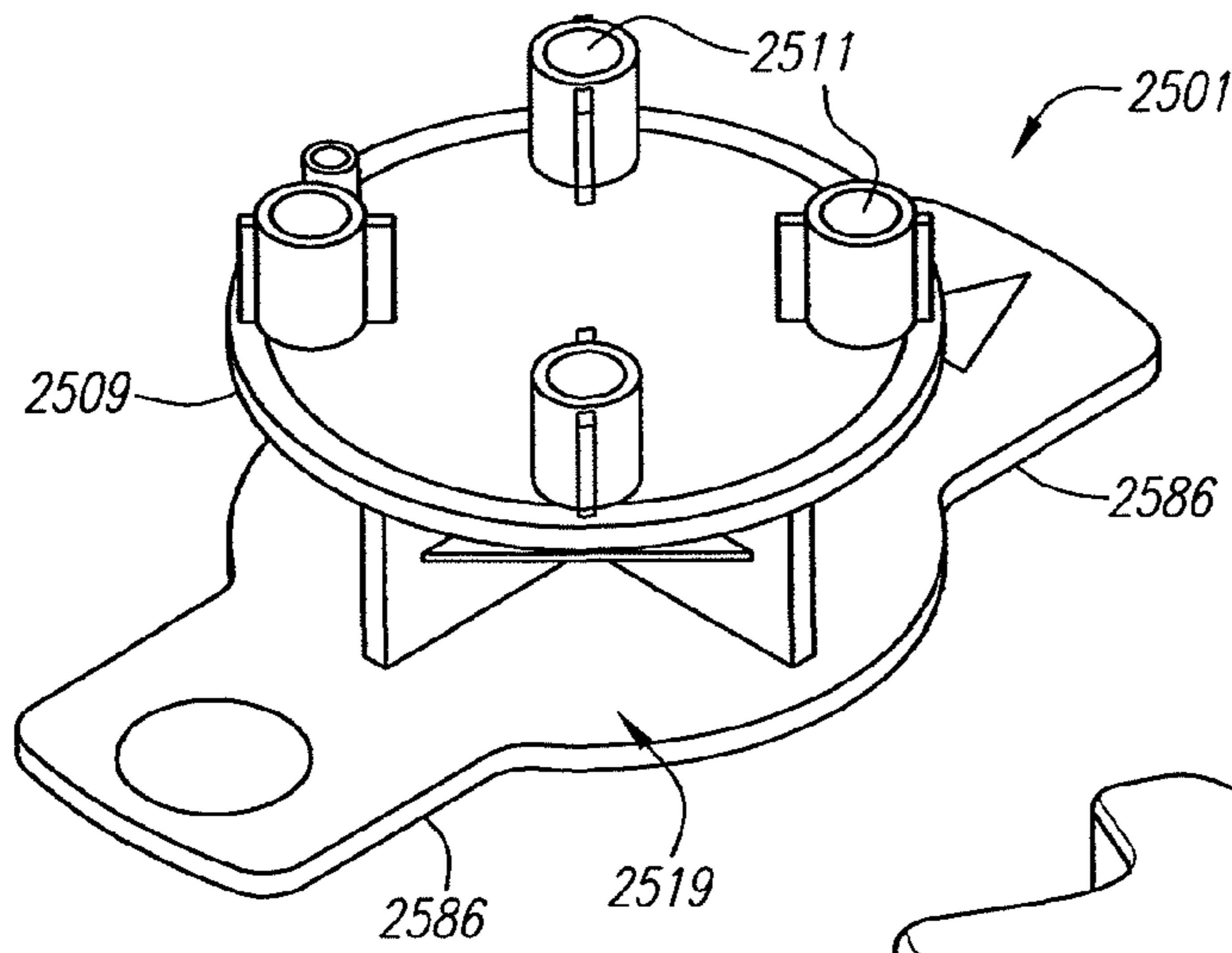
FIG. 25
