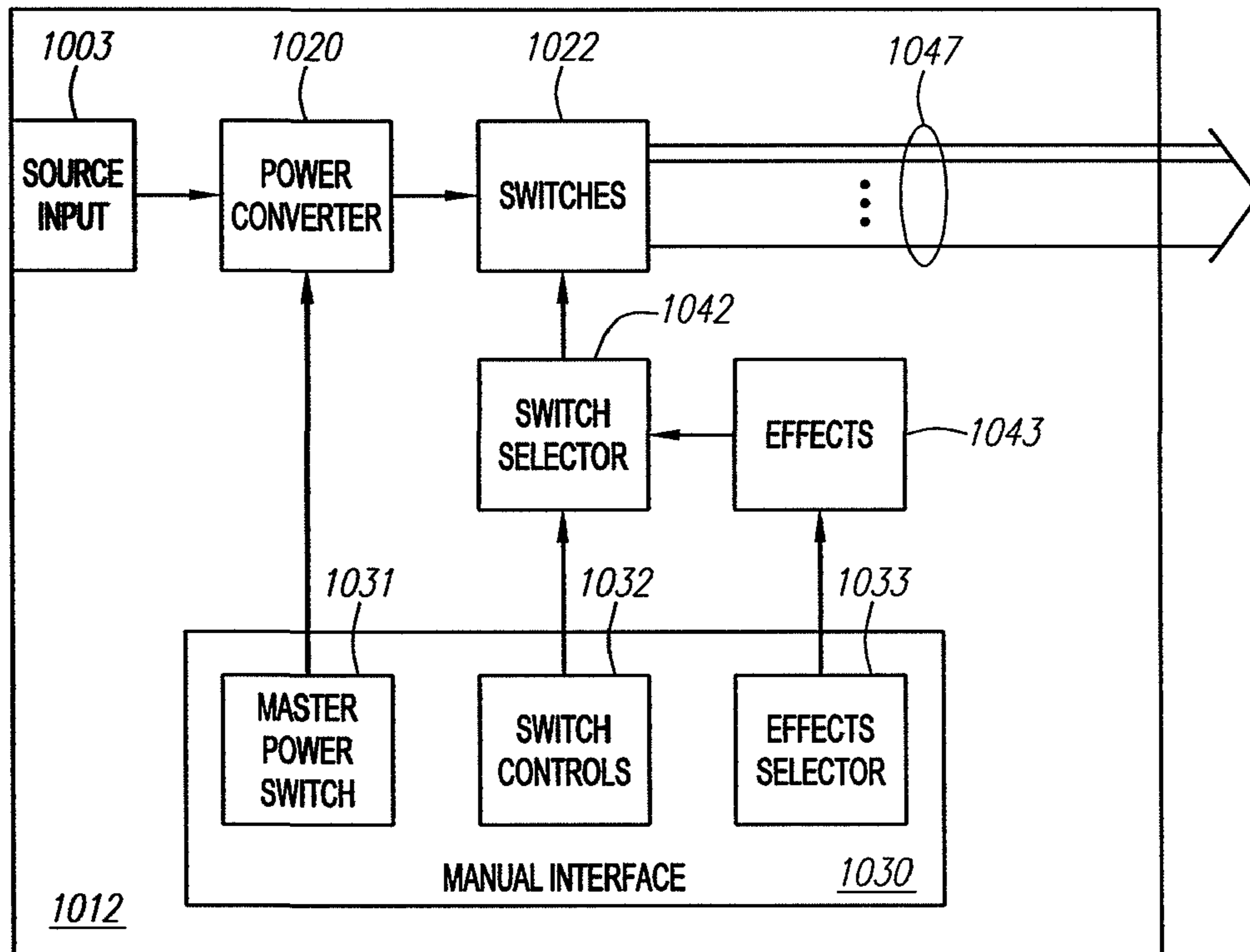
FIG. 10A
