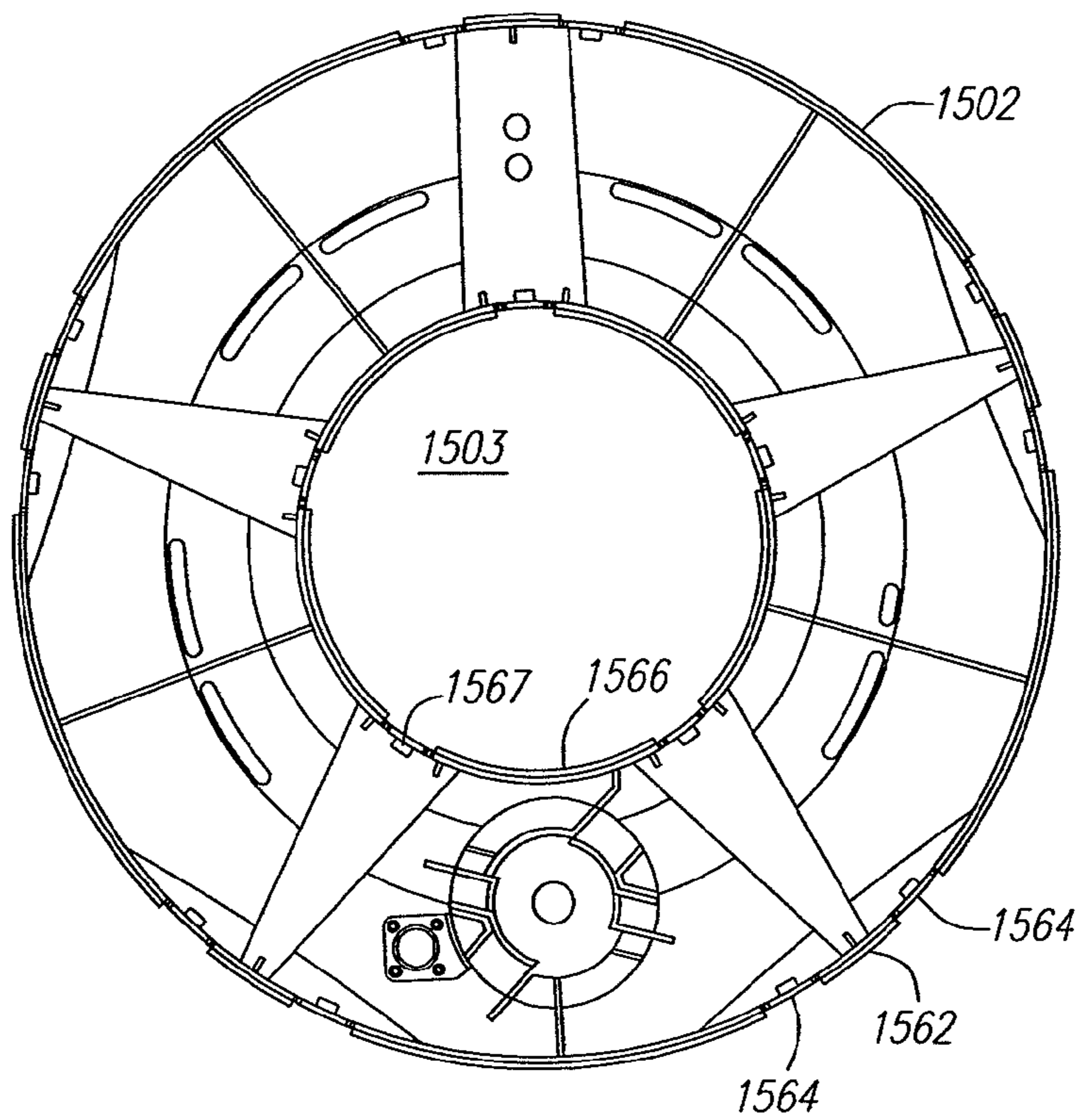
FIG. 16B
