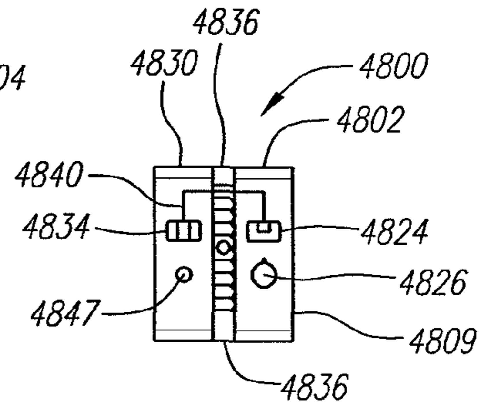
FIG. 48B
