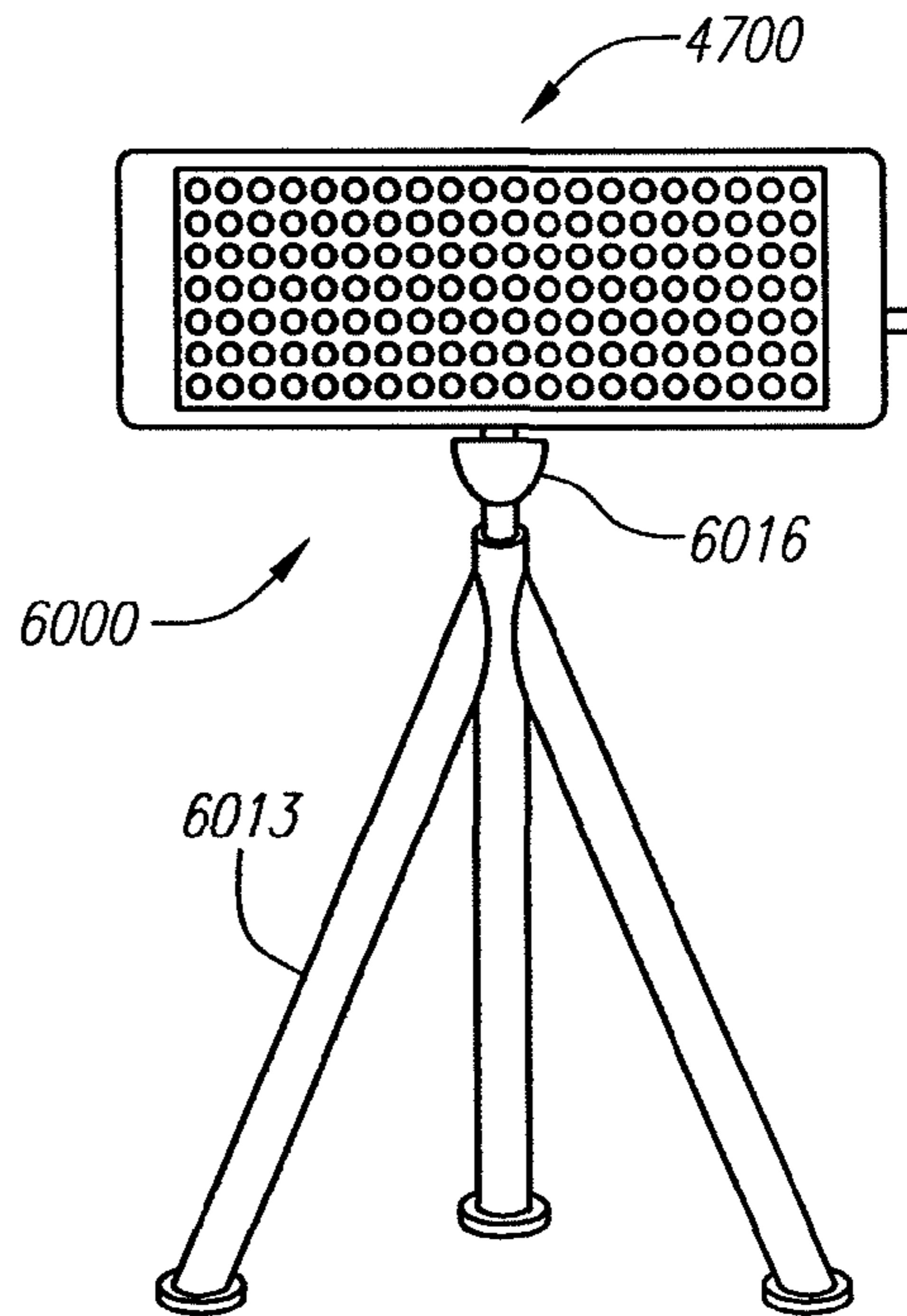
FIG. 60
