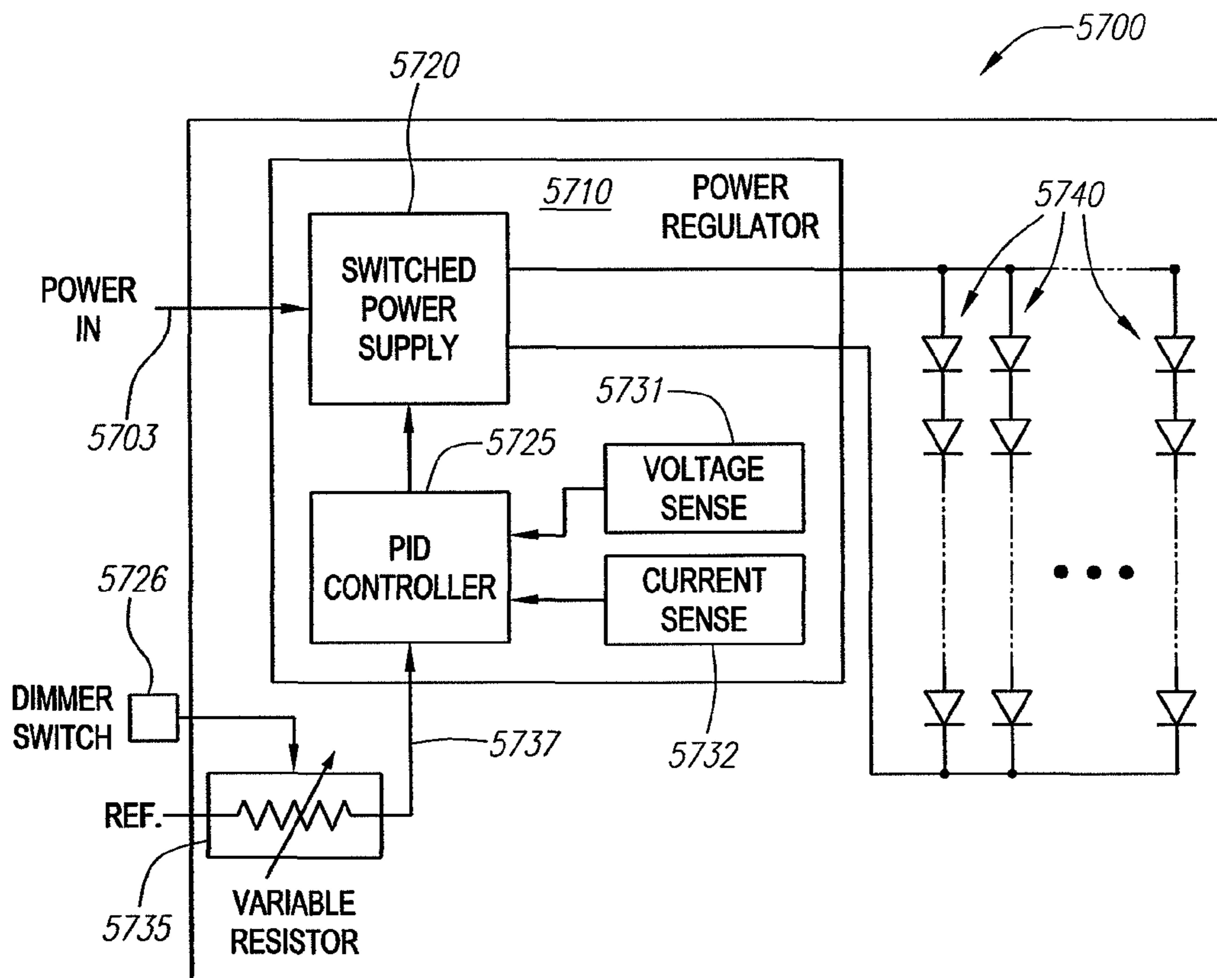
FIG. 57
