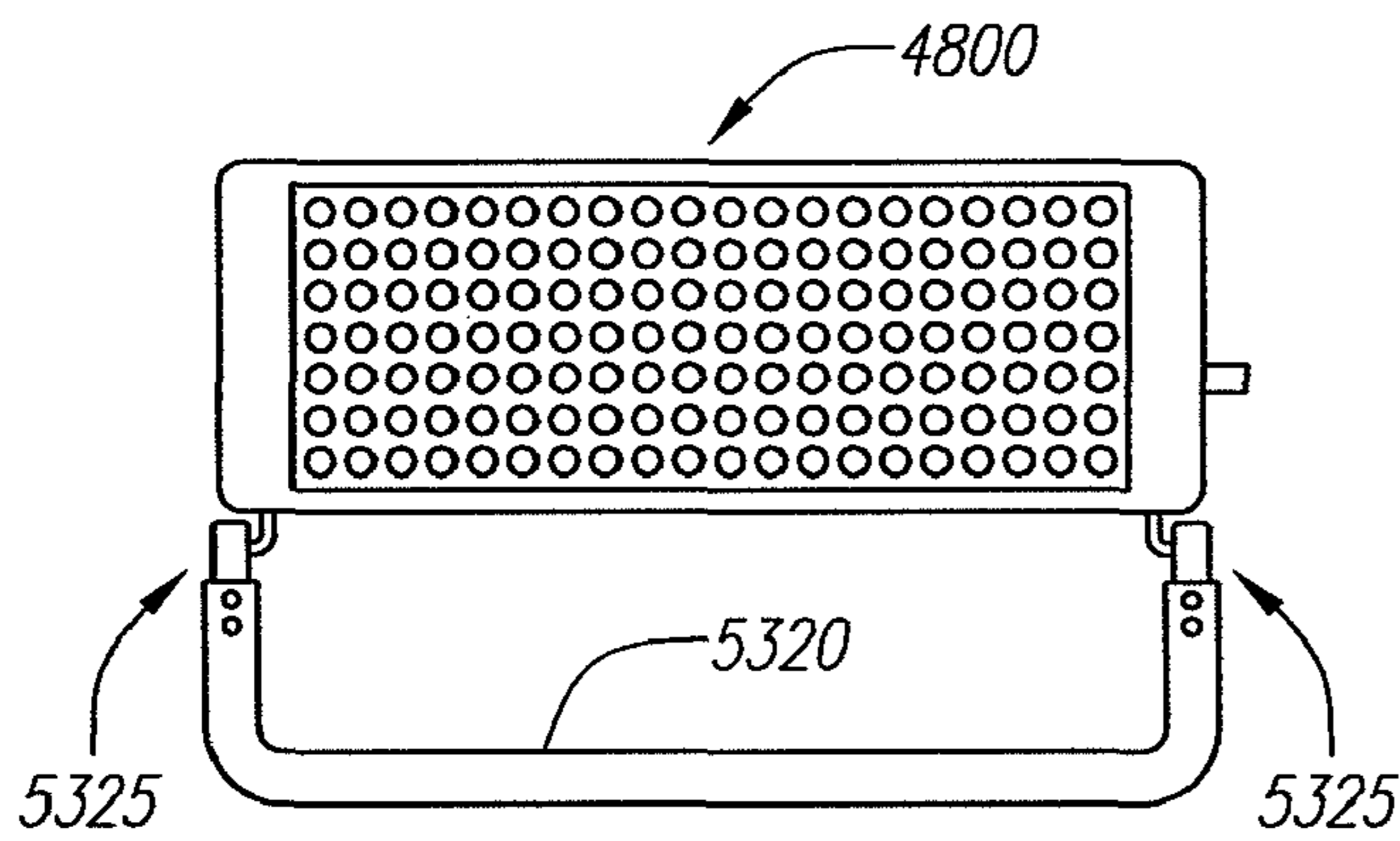
FIG. 53C
