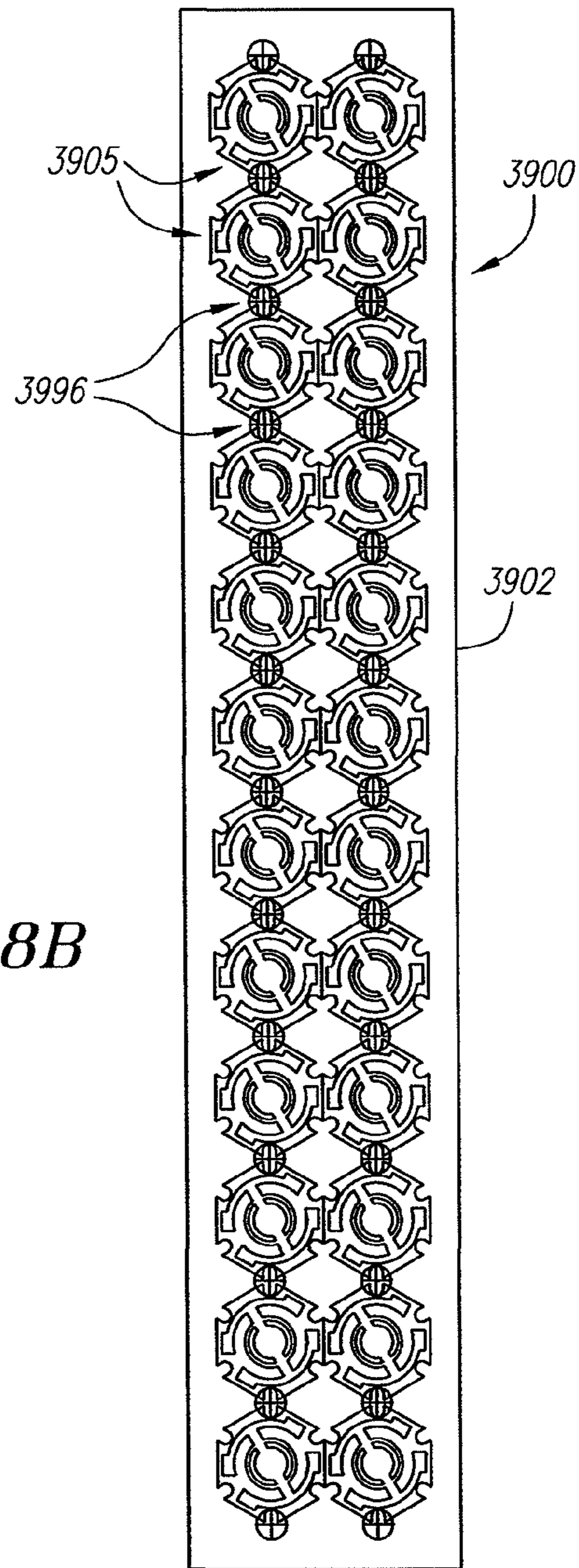
FIG. 39
