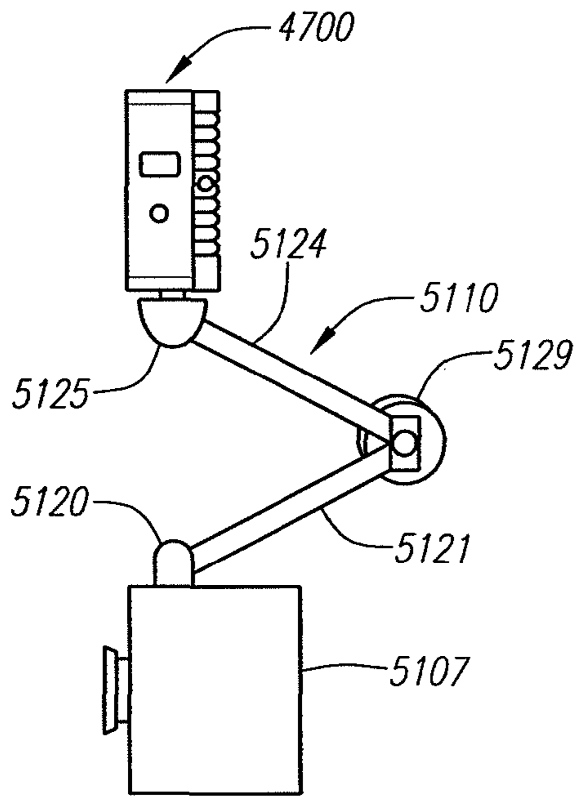
FIG. 51
