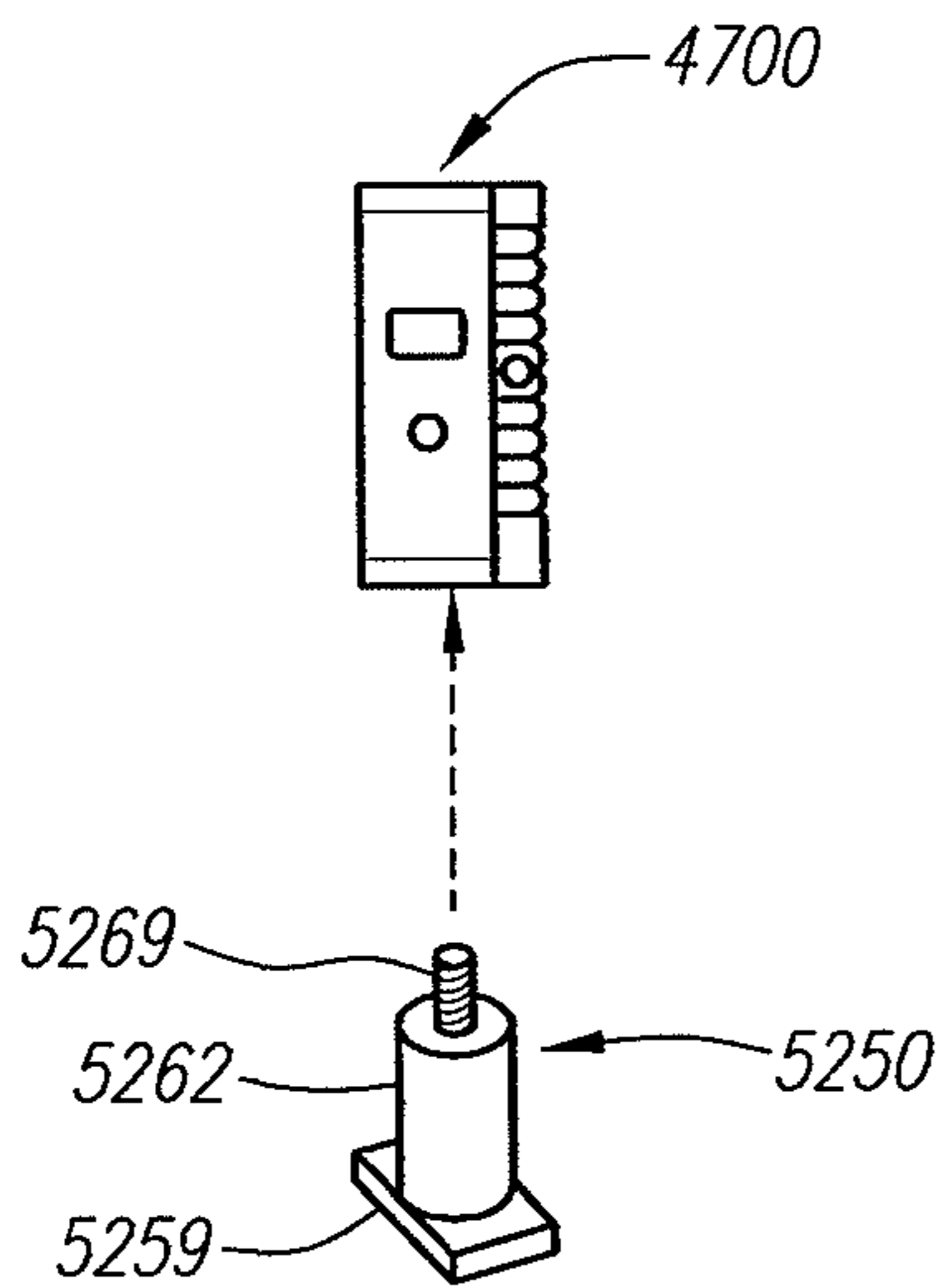
FIG. 52B
