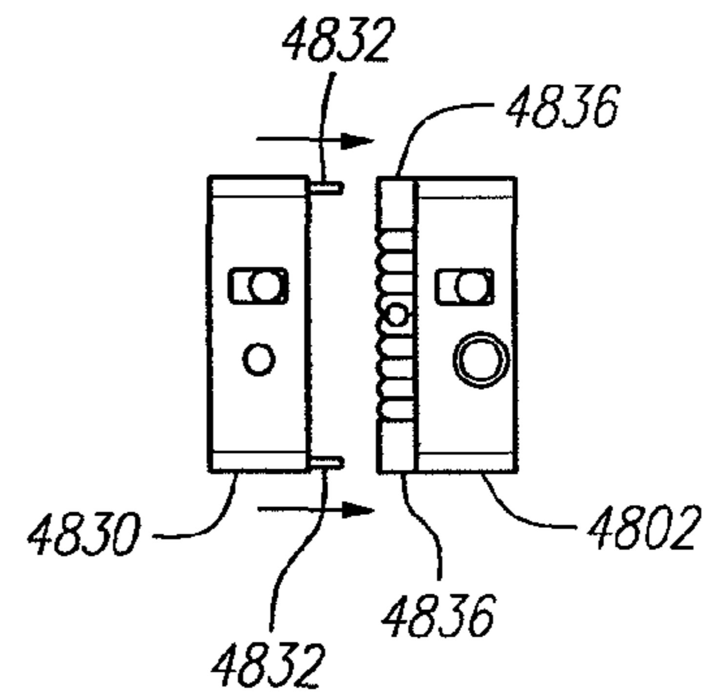
FIG. 49B
