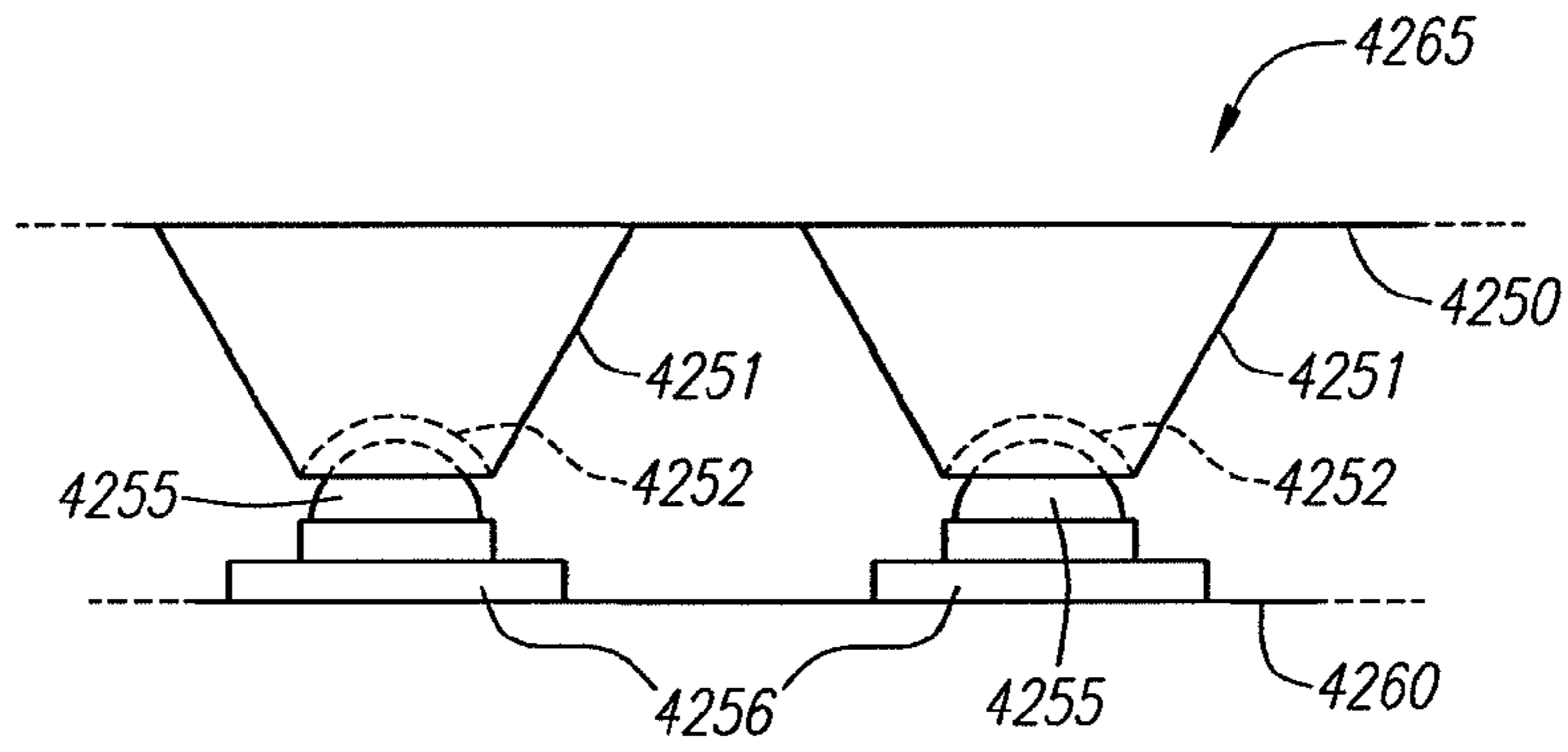
FIG. 42C
