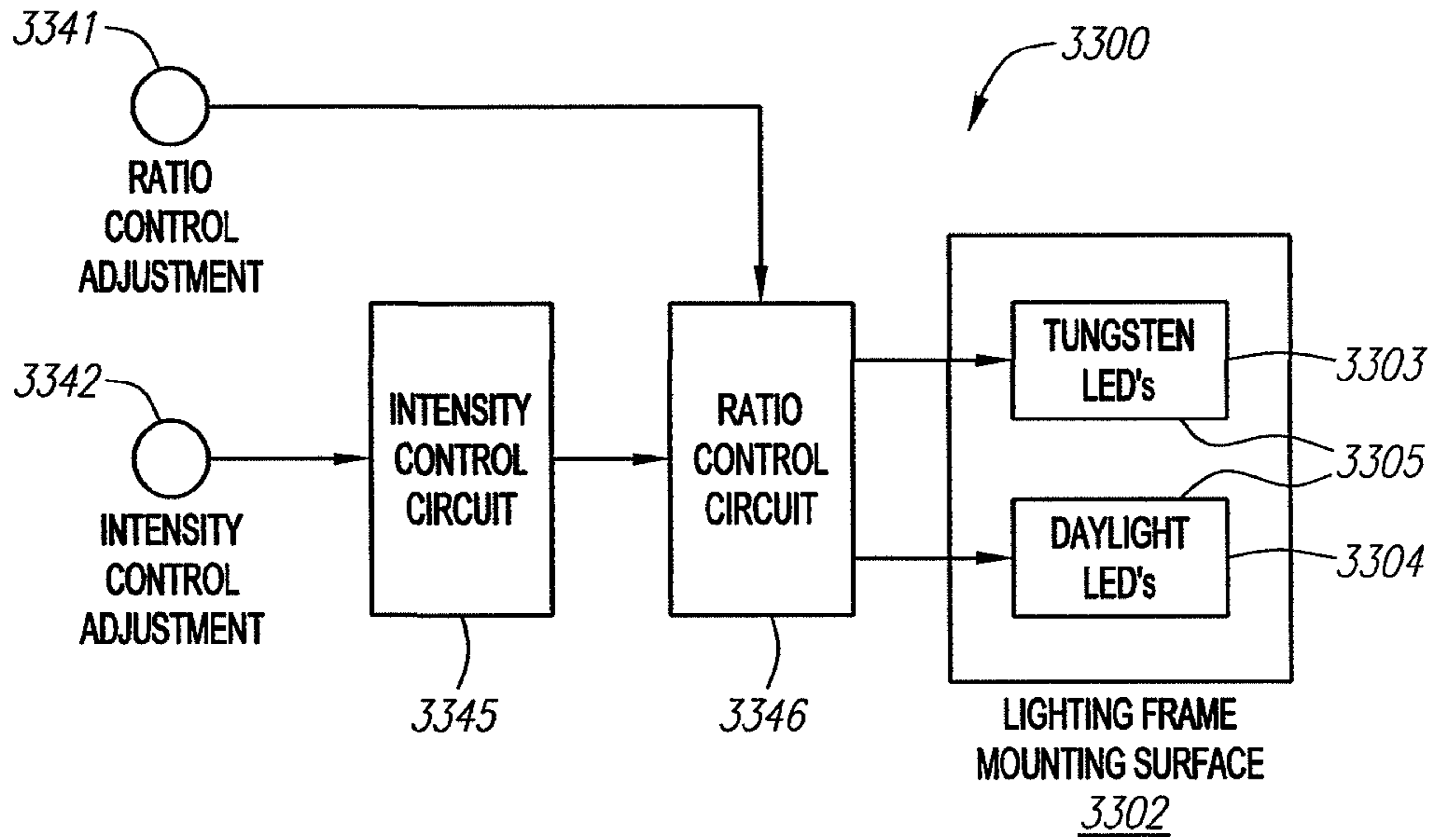
FIG. 33
