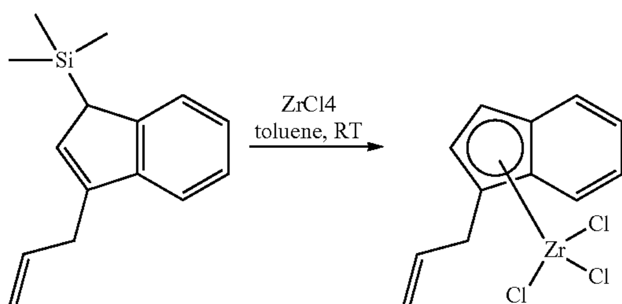
EQN. 11
