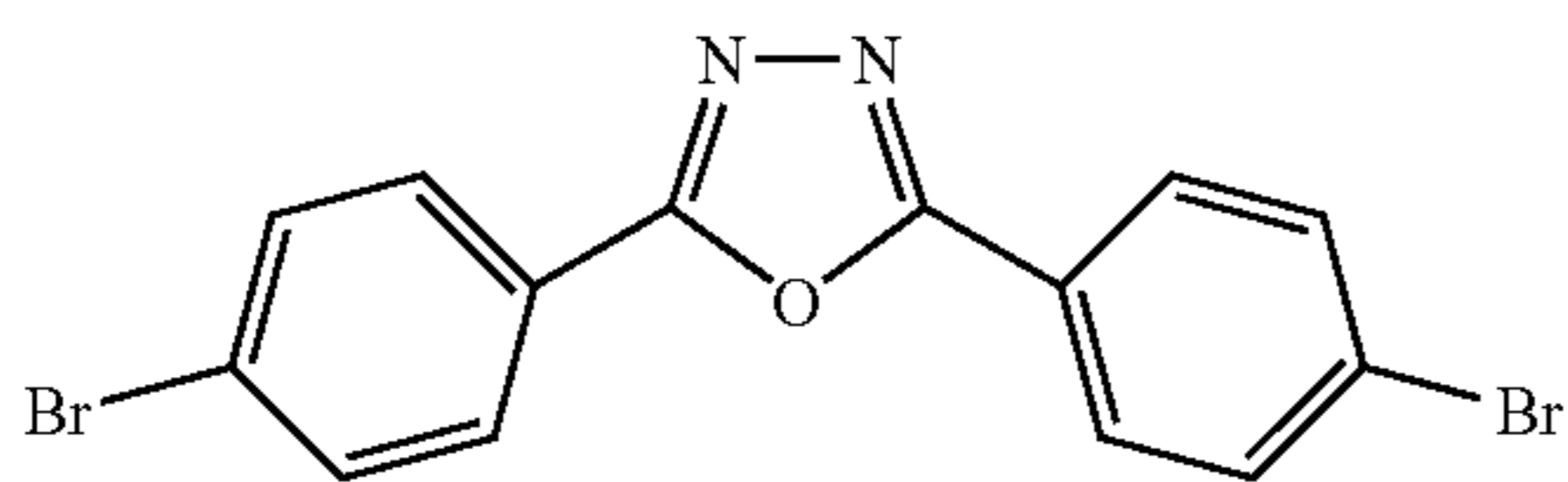
2,5-Bis-(4-bromo-phenyl)-[1,3,4]oxadiazole
