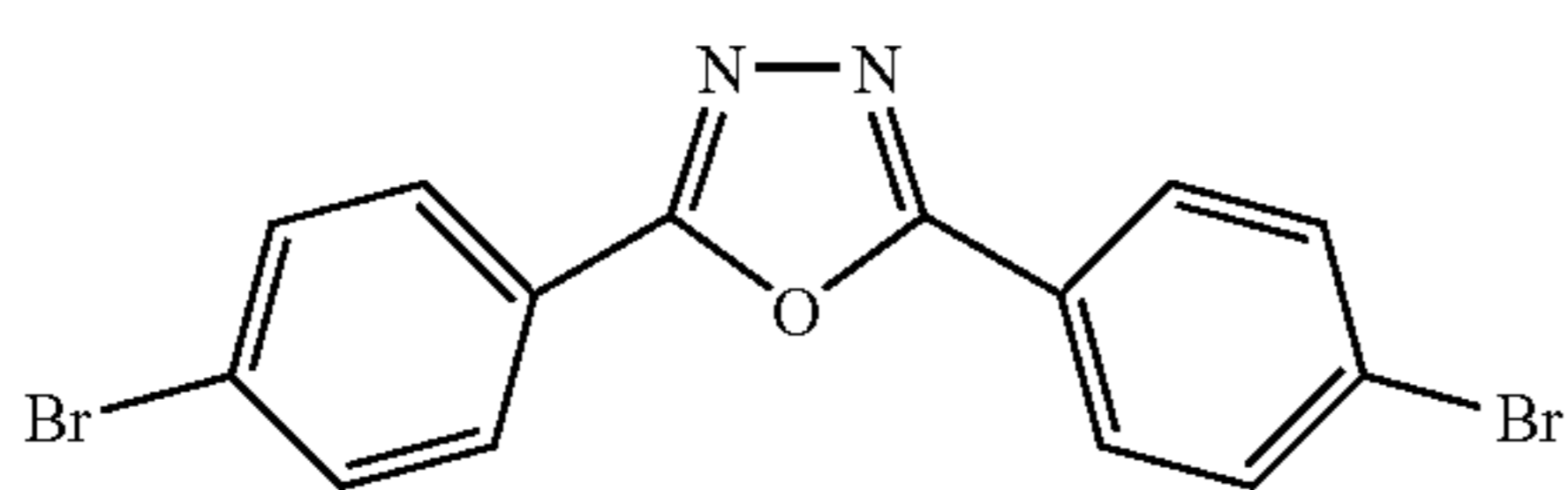
2,5-Bis-(4-bromo-phenyl)-[1,3,4]oxadiazole
