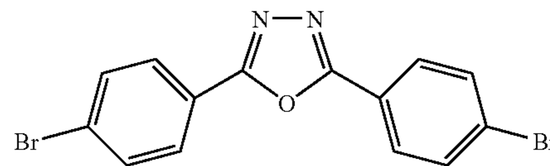
2,5-Bis-(4-bromo-phenyl)-[1,3,4]oxadiazole
