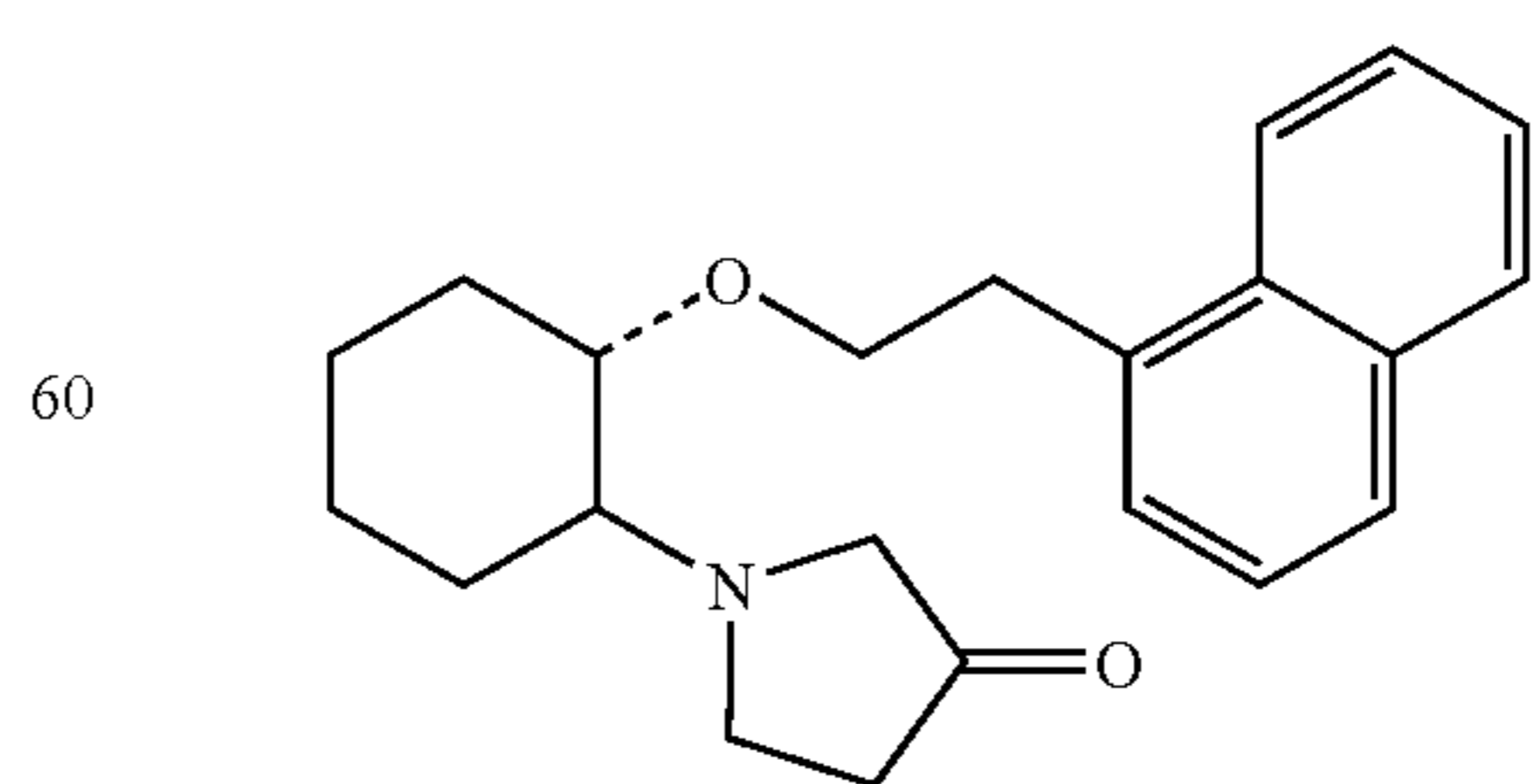
(1R,2R)/(1S,2S)-2-(3-ketopyrrolidinyl)-1-(1-naphthenethoxy)cyclohexane
