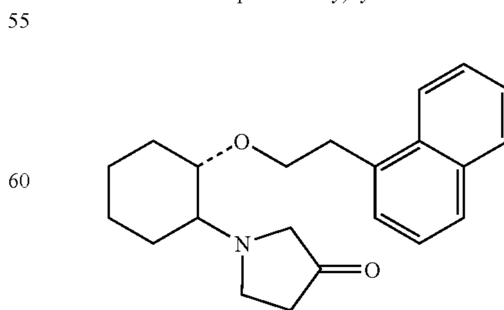
(1R,2R)/(1S,2S)-2-(3-ketopyrrolidinyl)-1-(1-naphthenethoxy)cyclohexane
