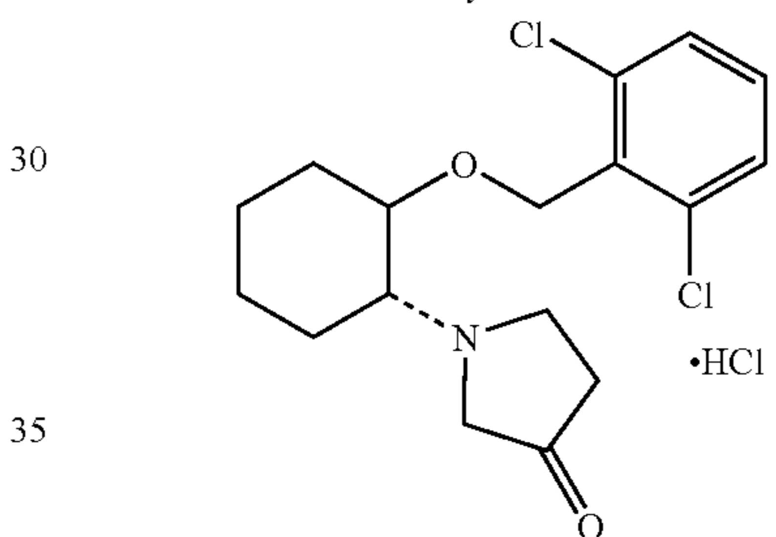
(1R,2R)/(1S,2S)-2-(3-ketopyrrolidinyl)-1-[2,6-dichlorophenyl)methoxy]cyclohexane monohydrochloride
