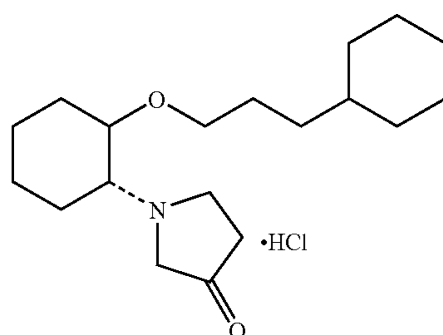
(1R,2R)/(1S,2S)-2-(3-ketopyrrolidinyl)-1-[3-(cyclohexy)propoxy]cyclohexane monohydrochloride
