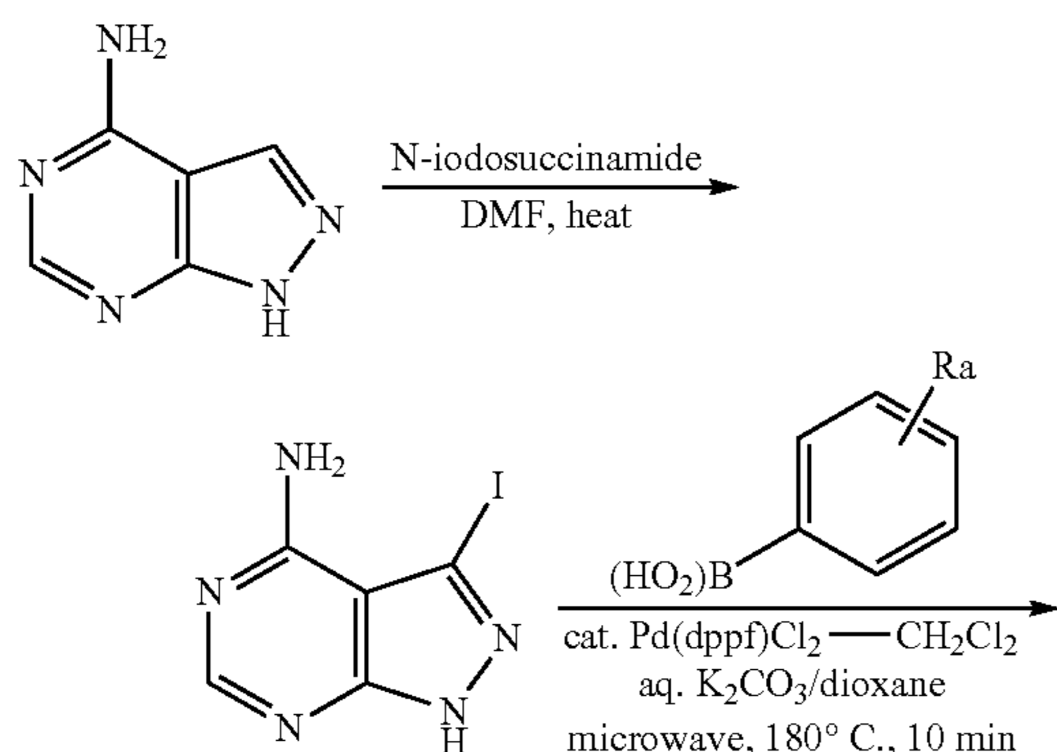
Scheme I.
