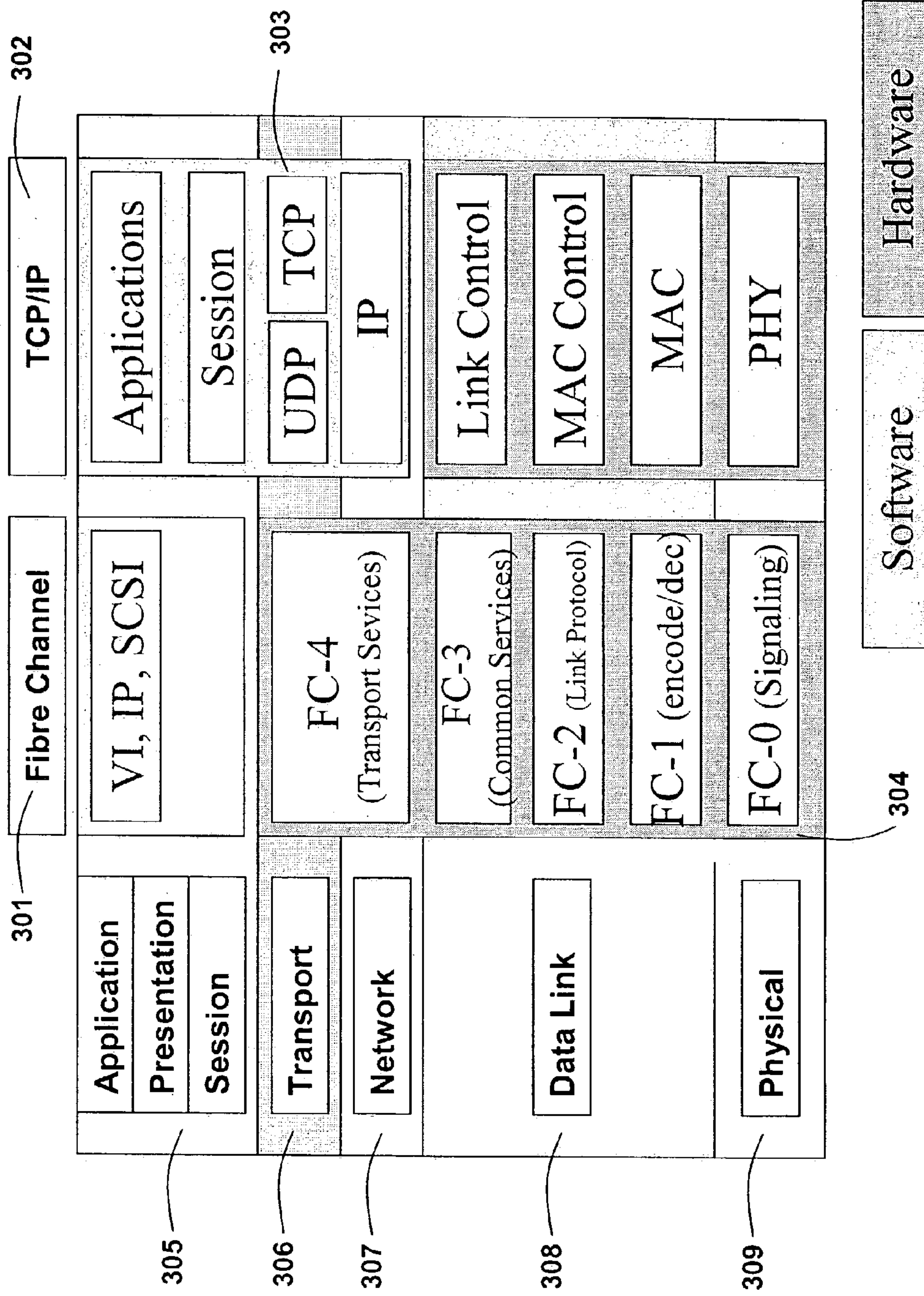
Fig. 3 OSI Stack
