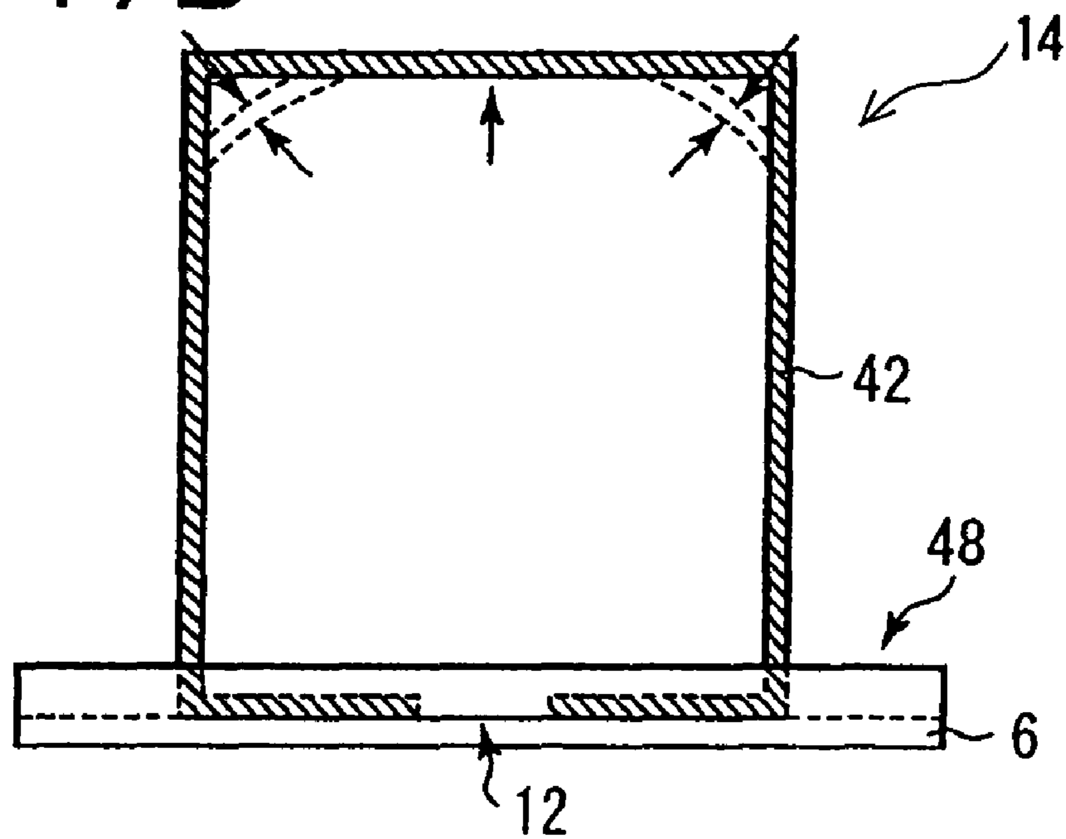
FIG. 17B
