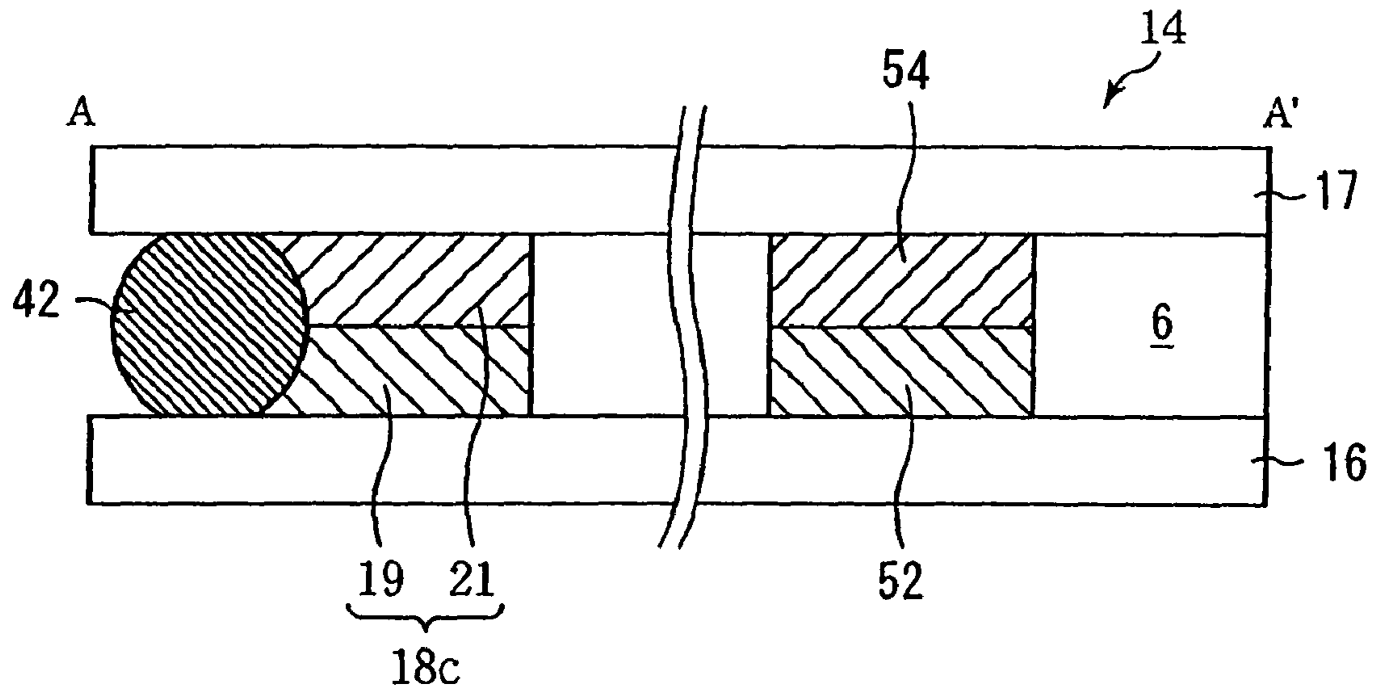
FIG. 26
