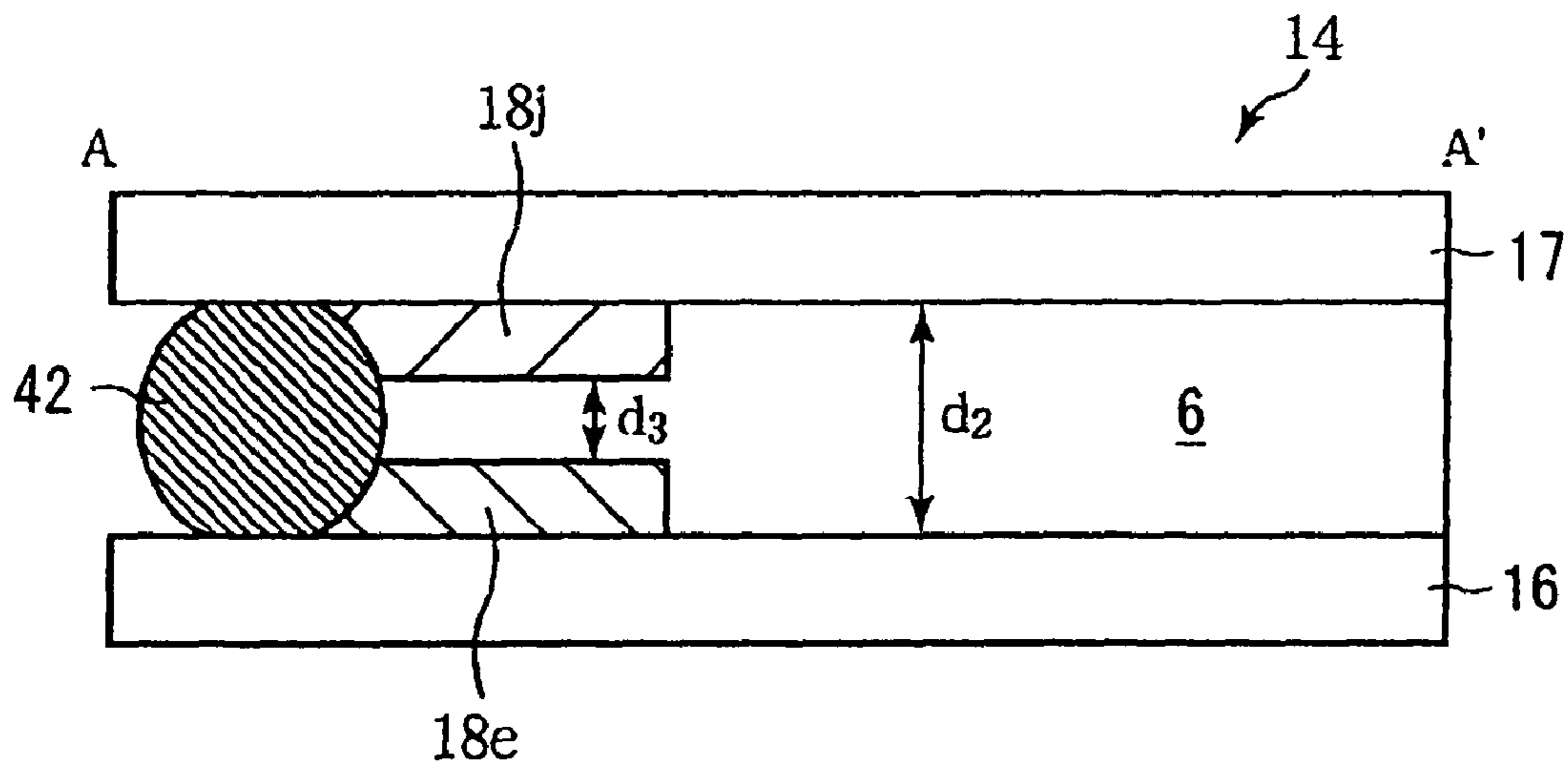
FIG. 33A
