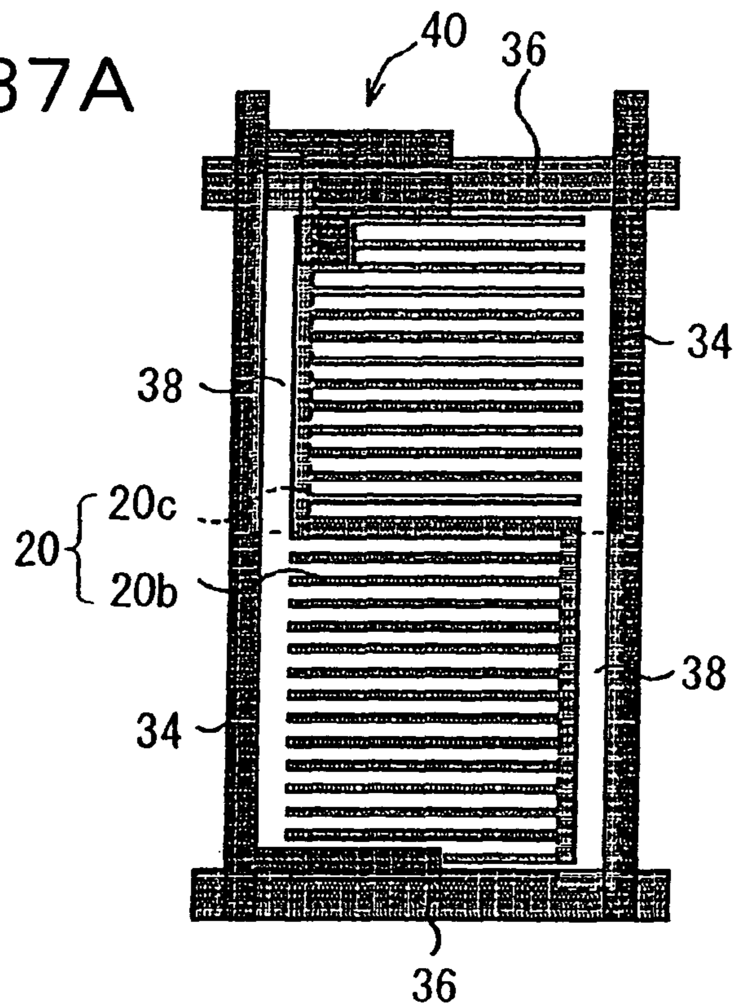
FIG. 37B
