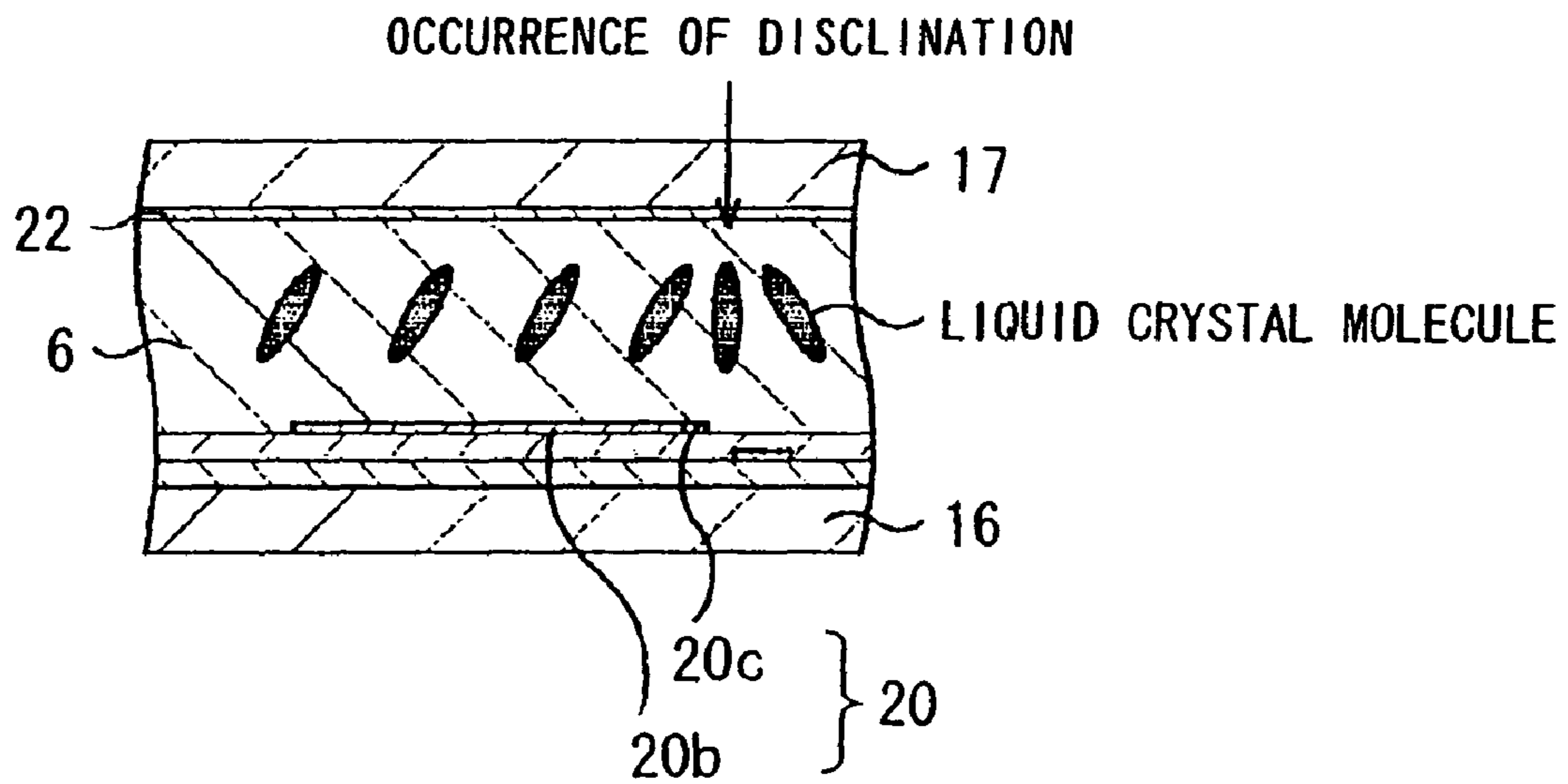
FIG. 36B
