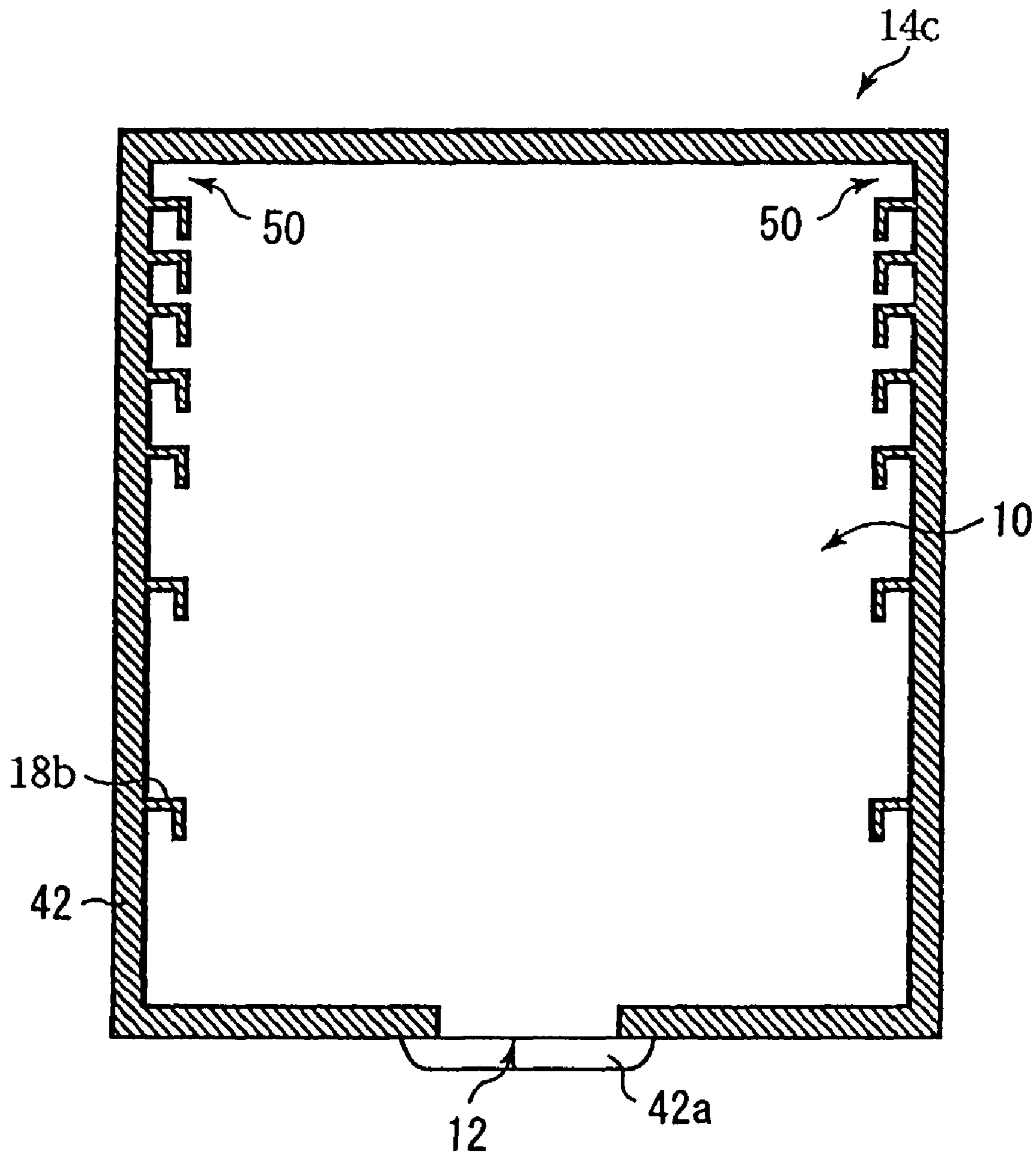
FIG. 24
