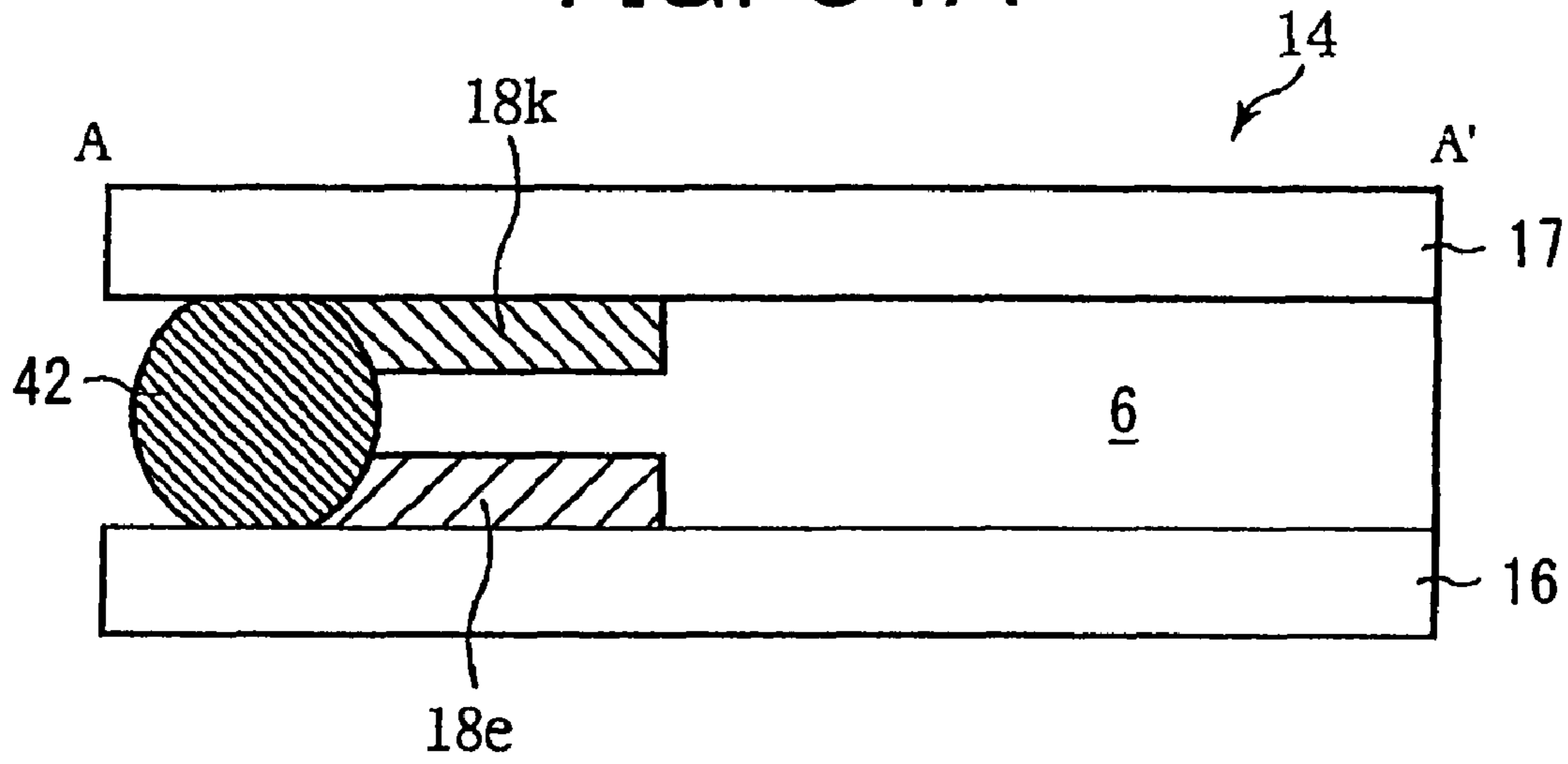
FIG. 34A
