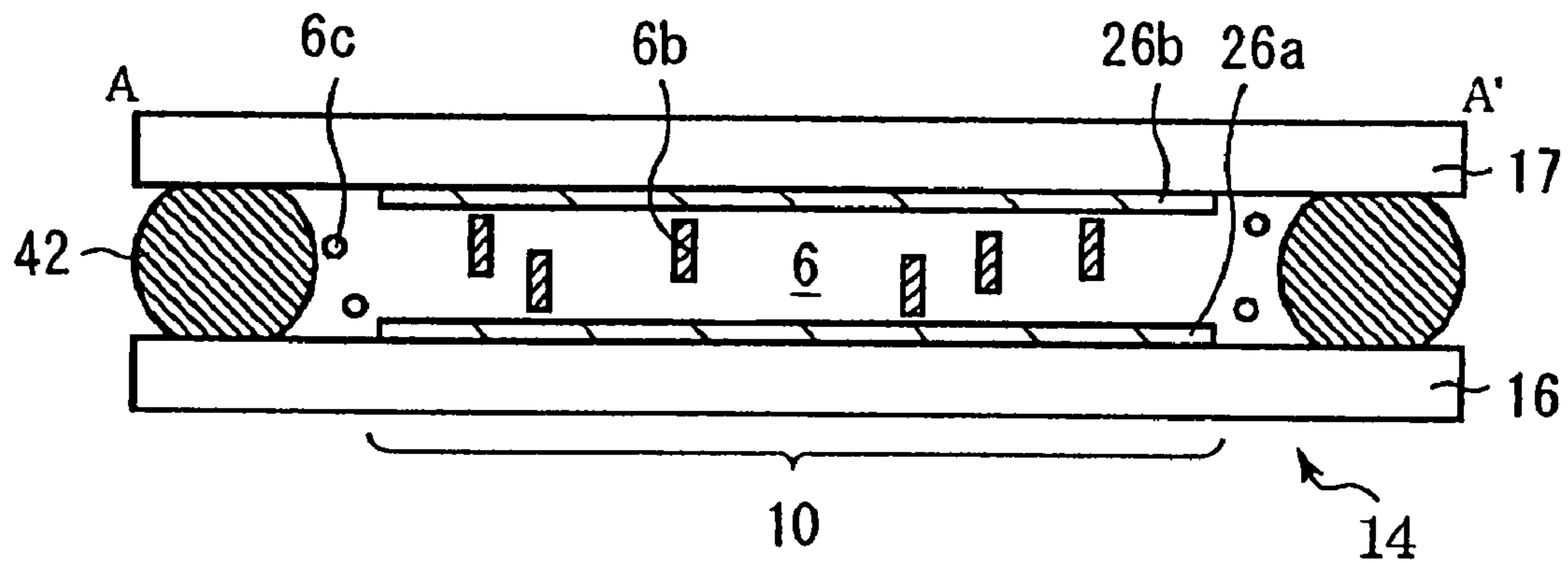
FIG. 15A
