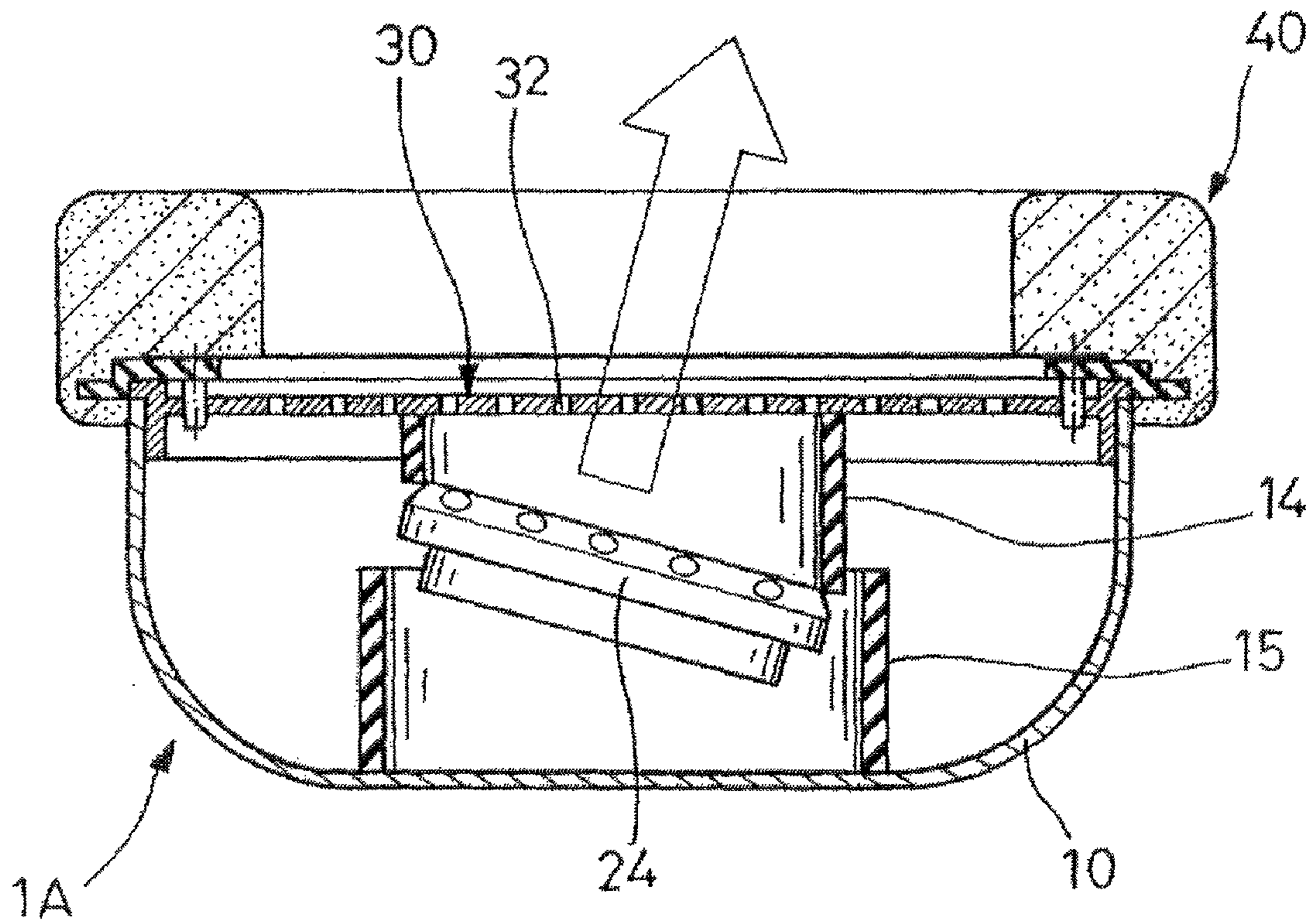
FIG. 2E (PRIOR ART)
