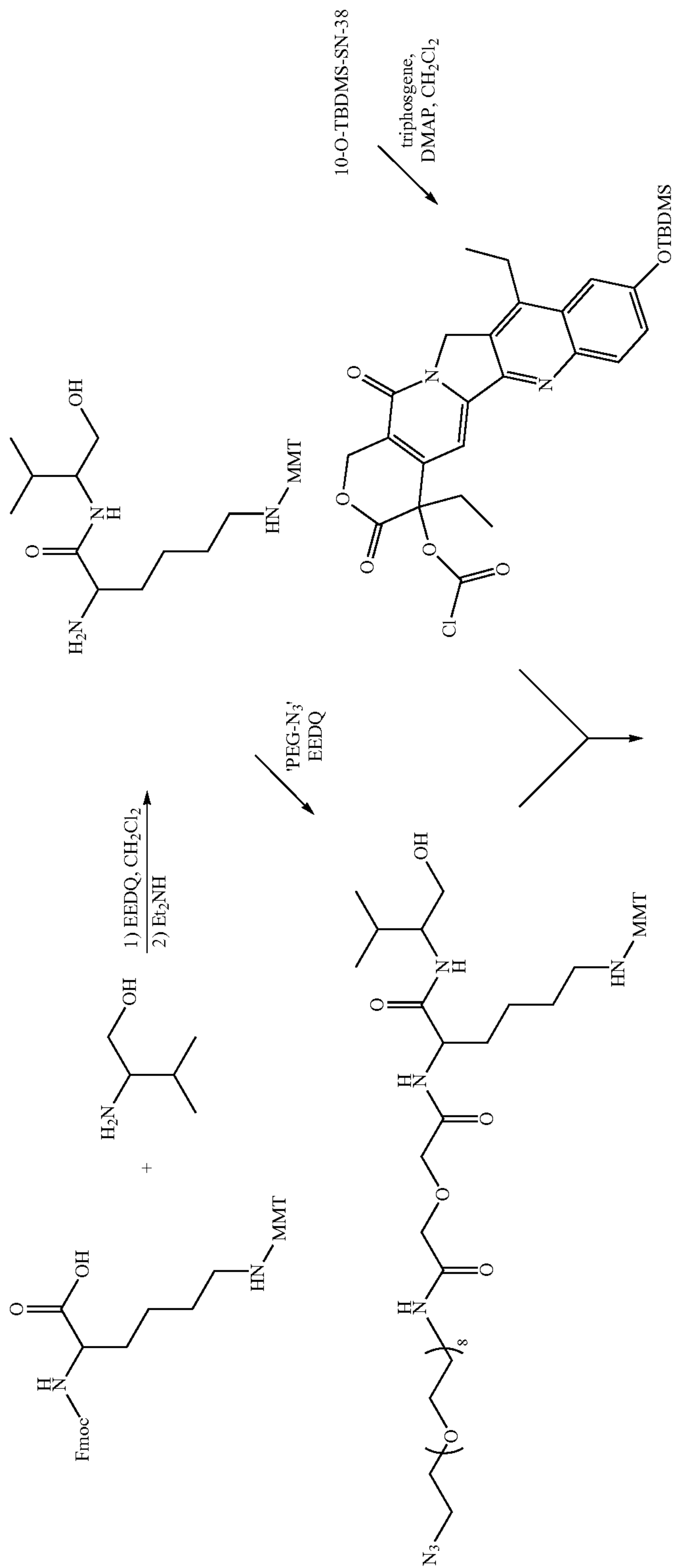
Scheme-2
