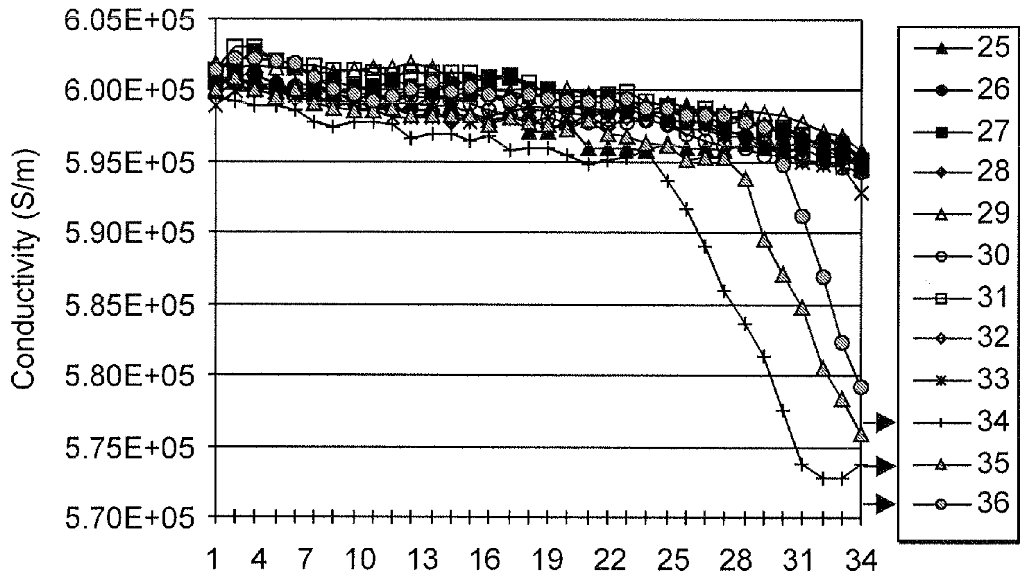
FIG. 43c Position (1/16" increments)
