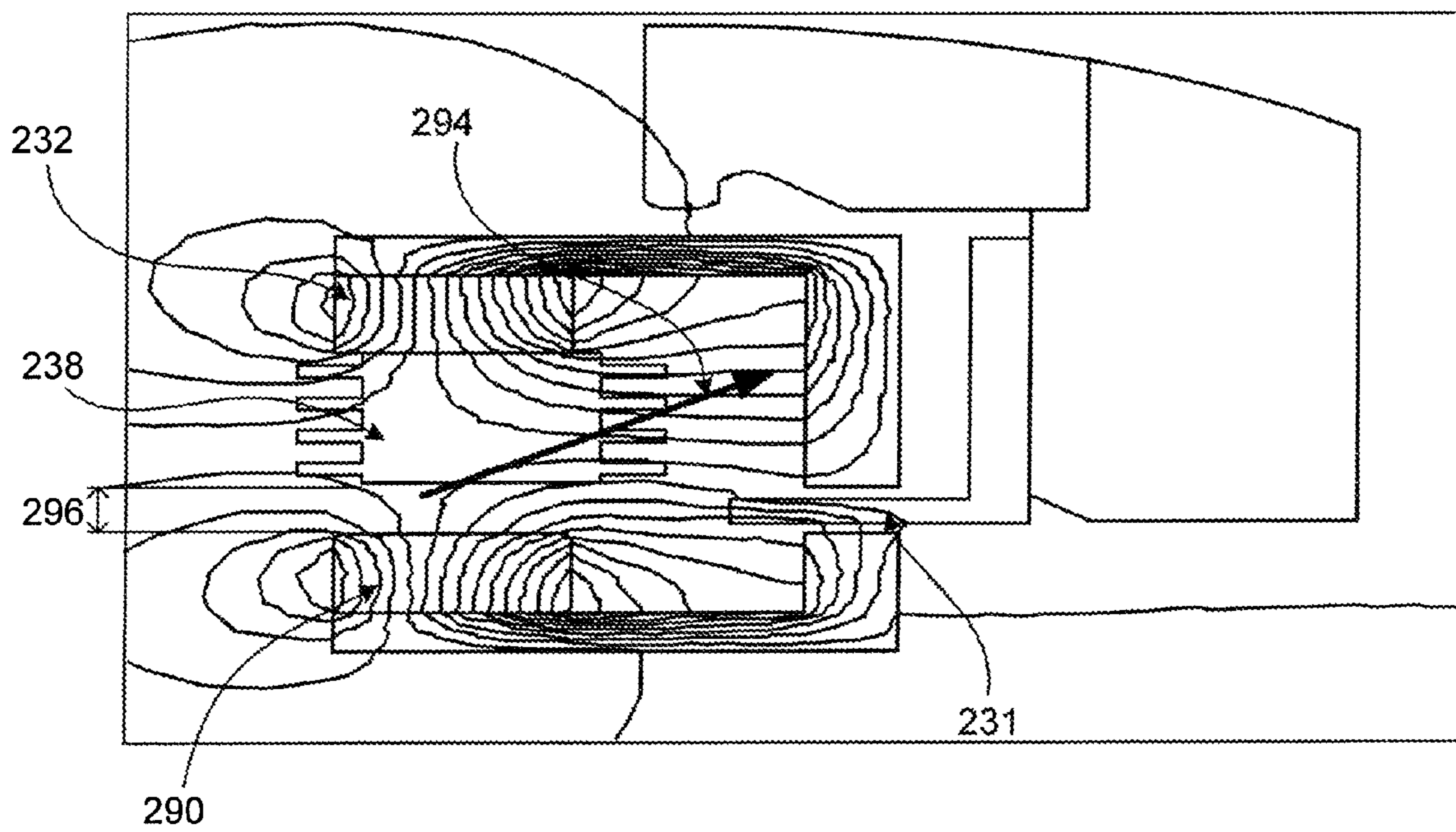
FIG. 13B
