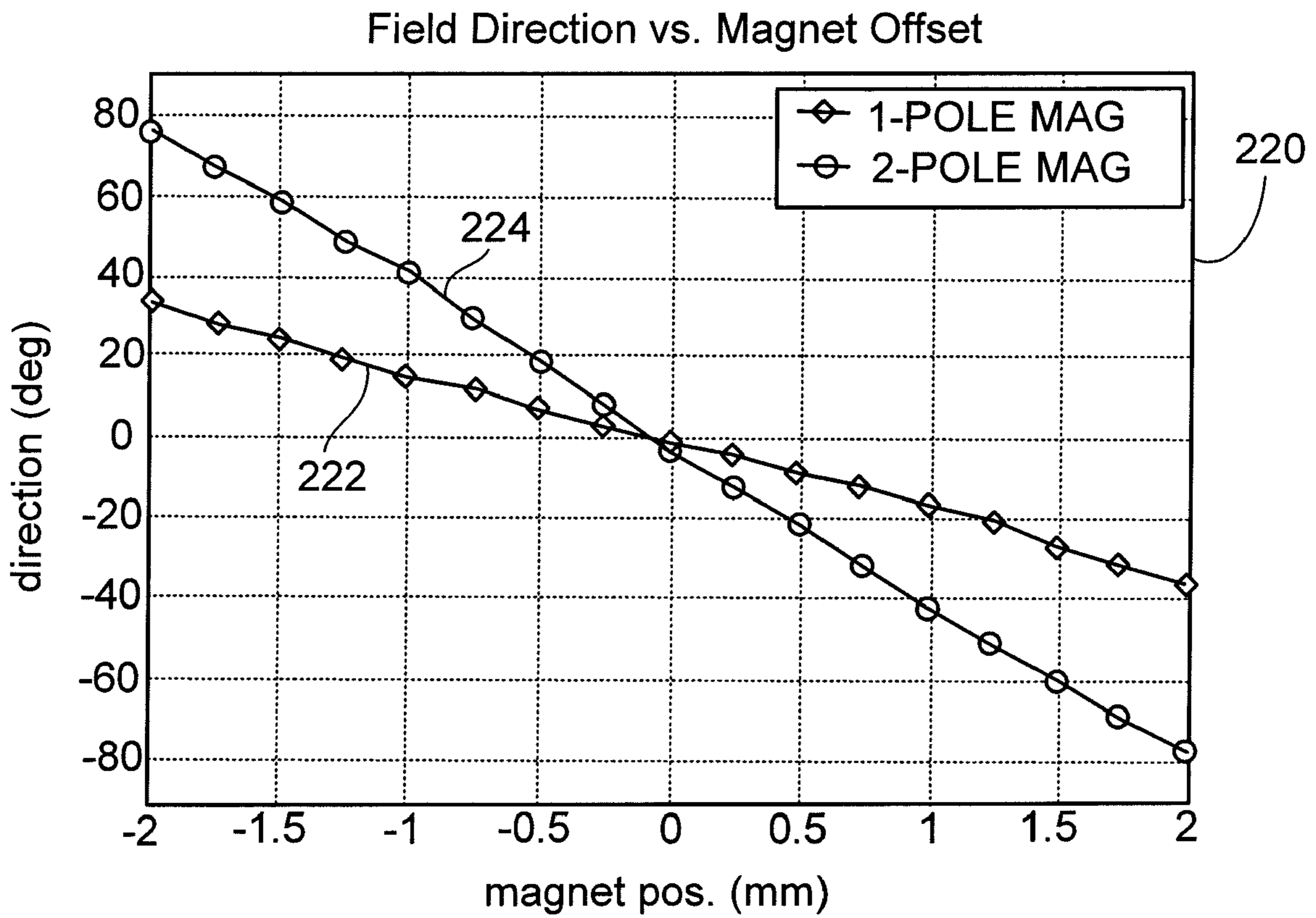
FIG. 11B
