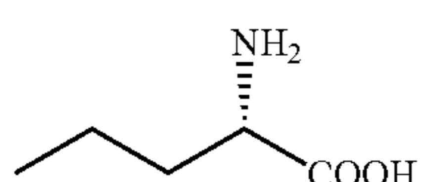
L-norvaline
