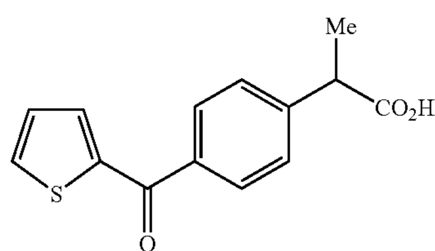
Suprofen
