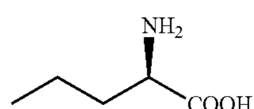
D-norvaline
