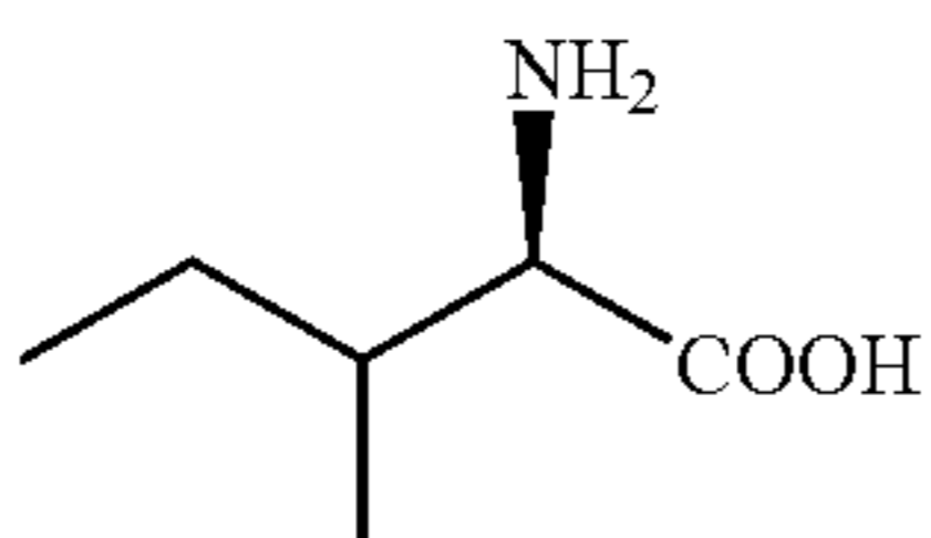
D-isoleucine
