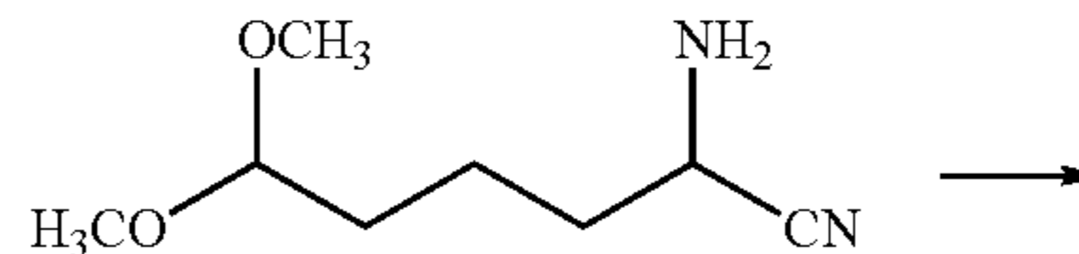
2-amino-6,6-dimethoxy hexanenitrile
