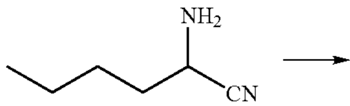
2-amino hexanenitrile
