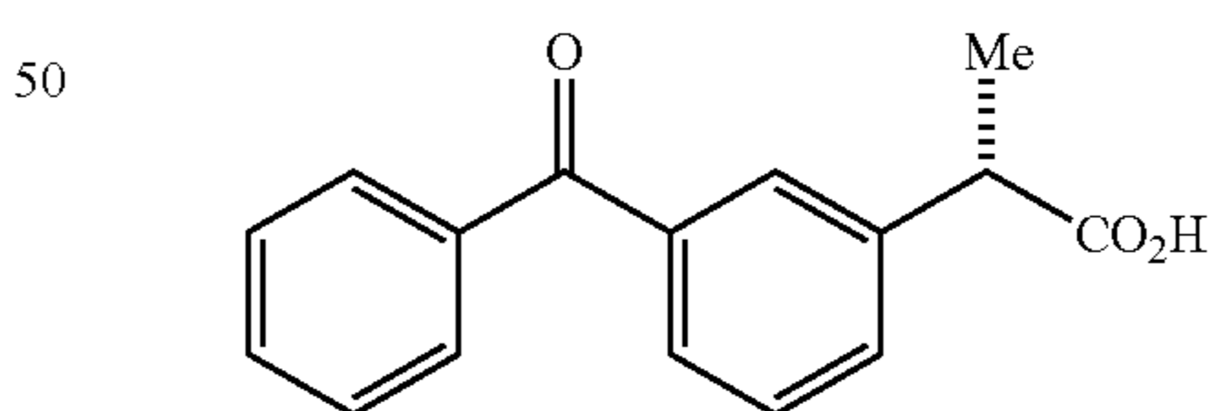
Dexketoprofen
