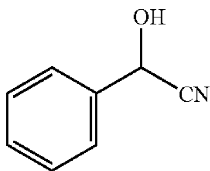
mandelonitrile
