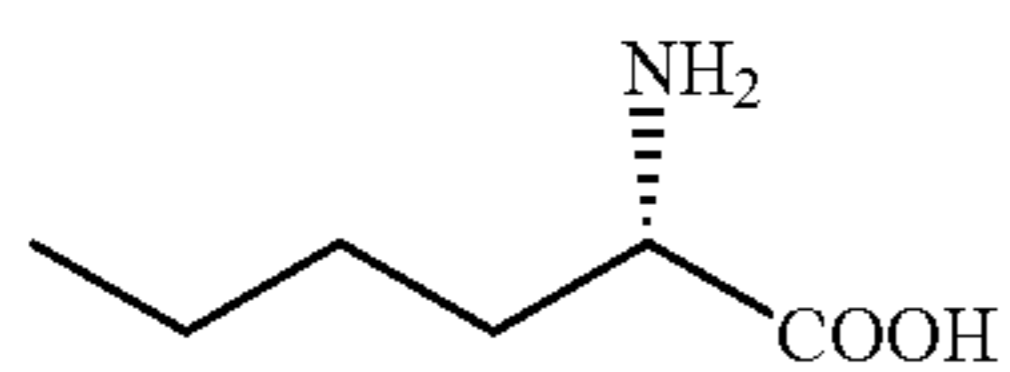
L-norleucine
