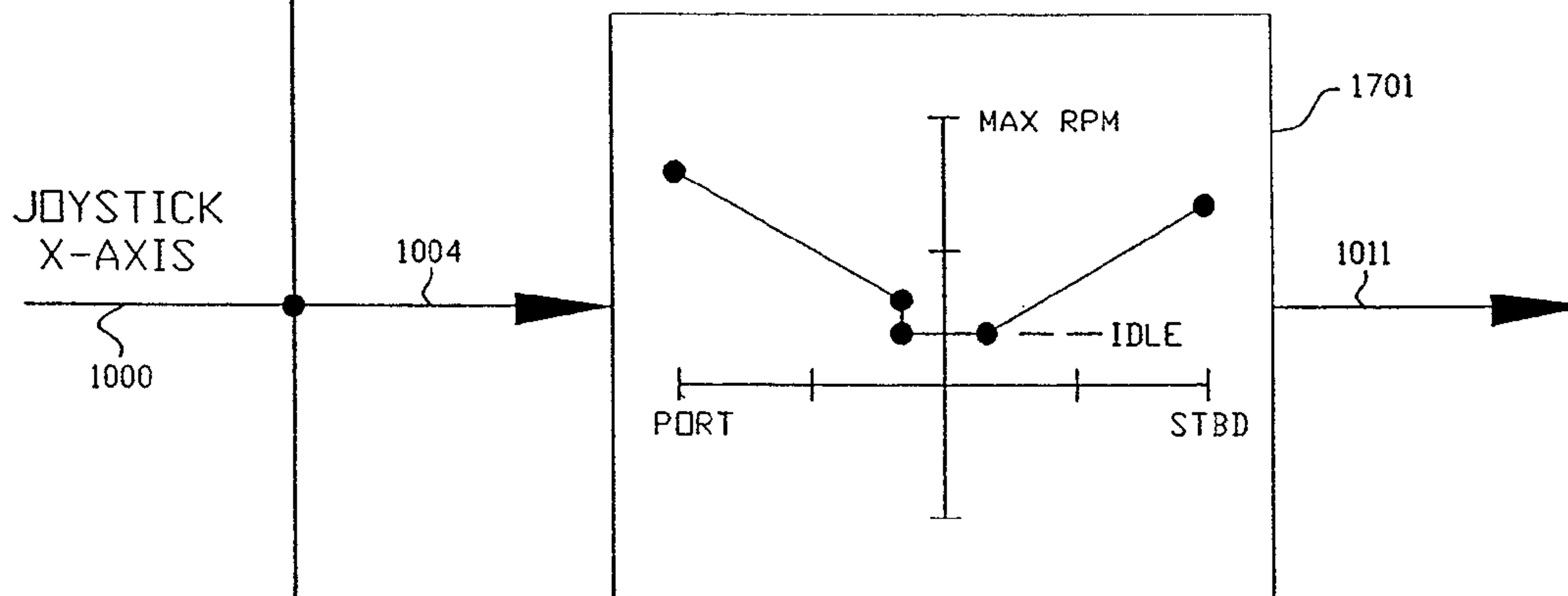
FIG. 14E PORT ENGINE RPM
