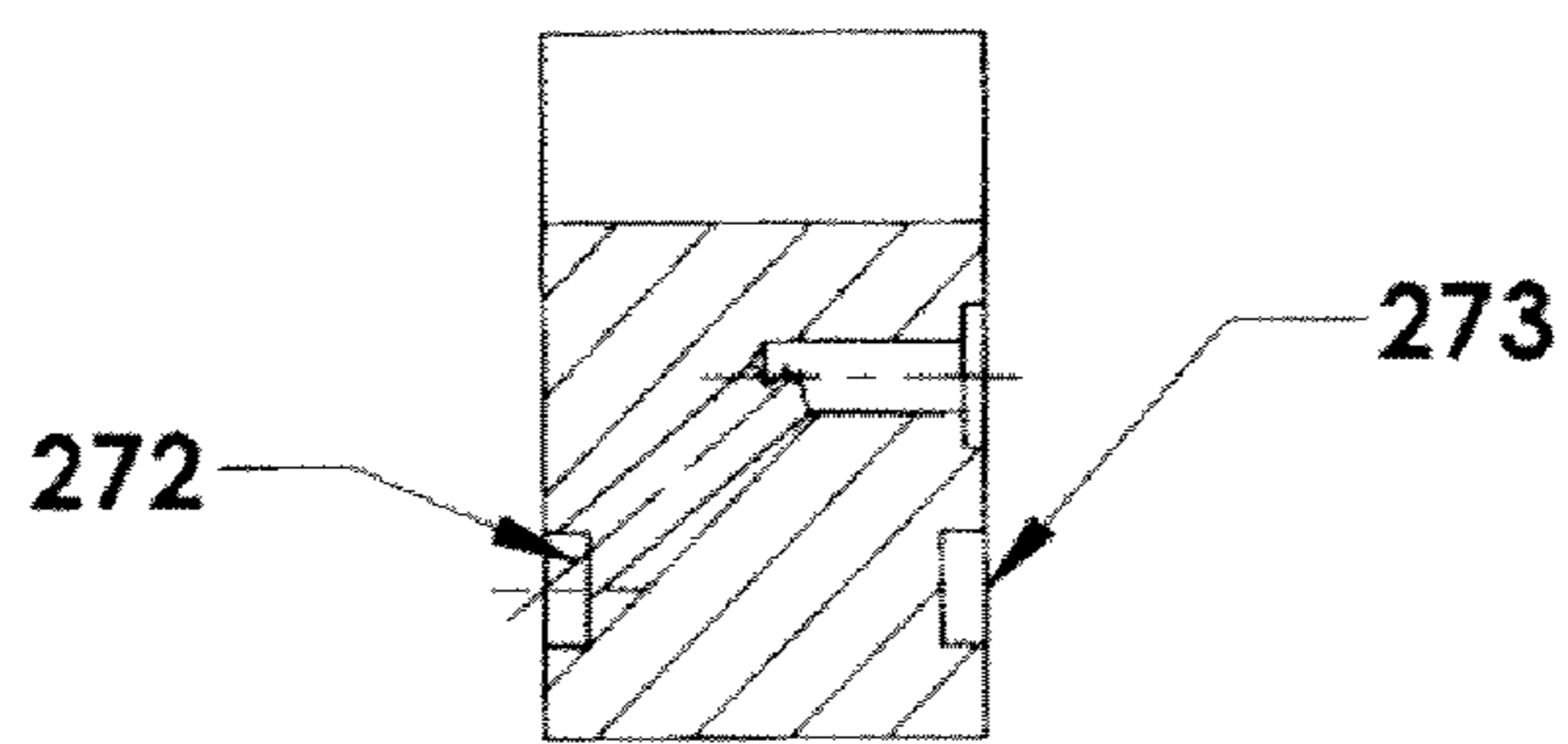
SECTION B-B FIG. 20
