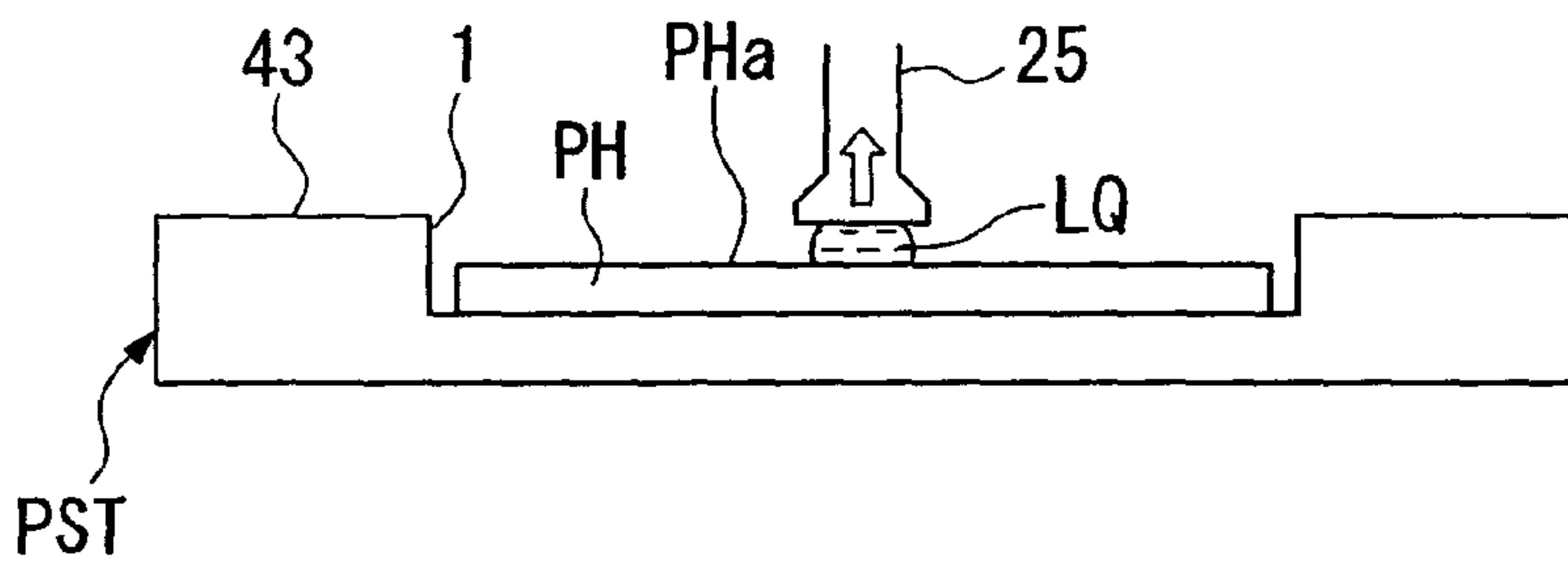
FIG. 13B
