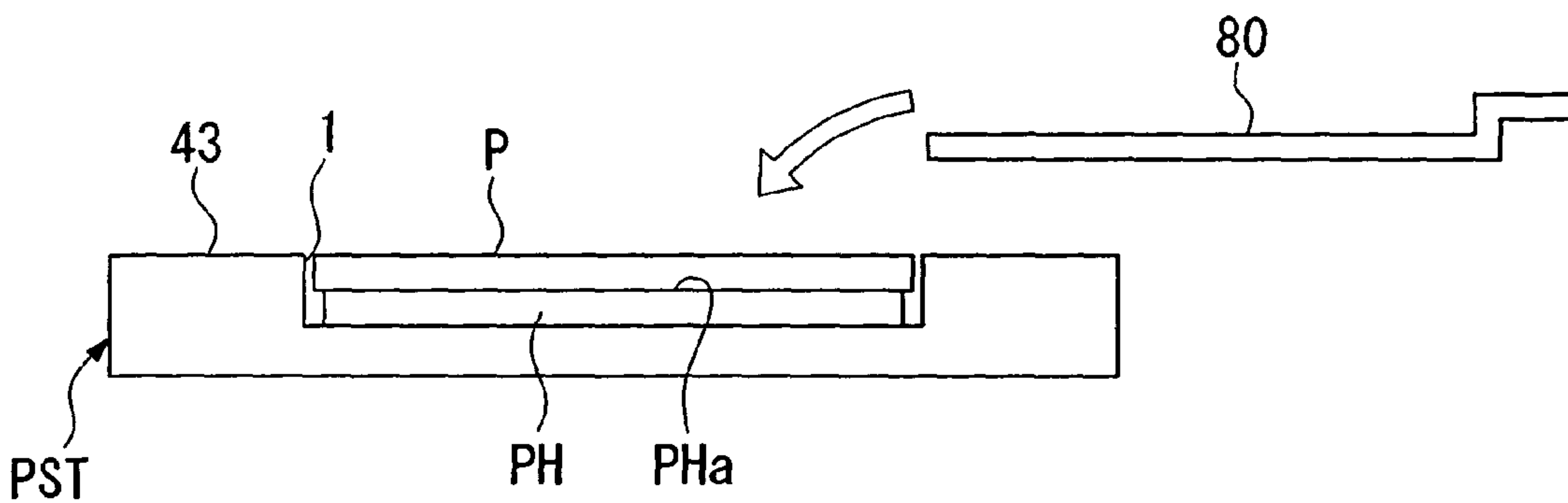
FIG. 13B
