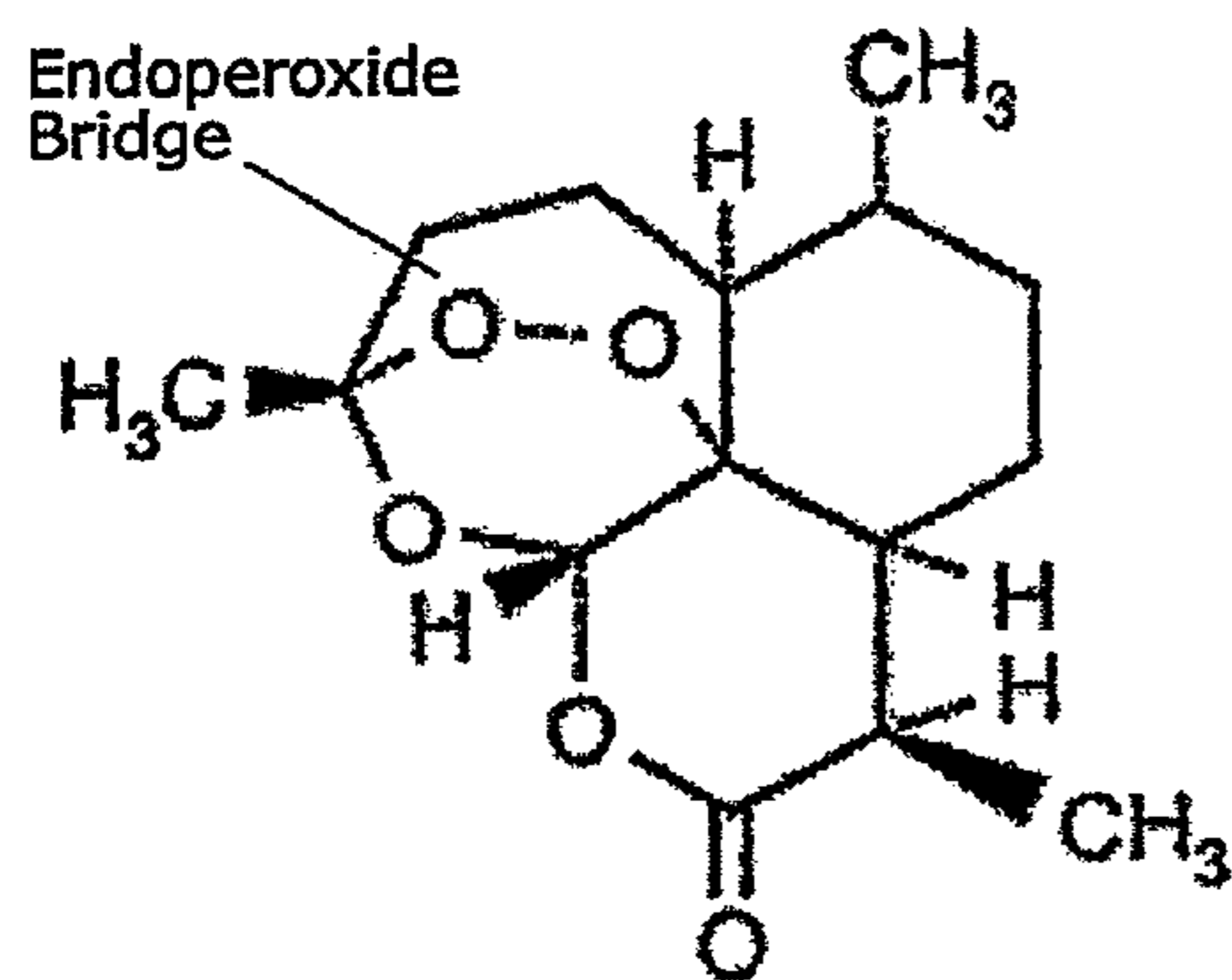
Artemisinin
