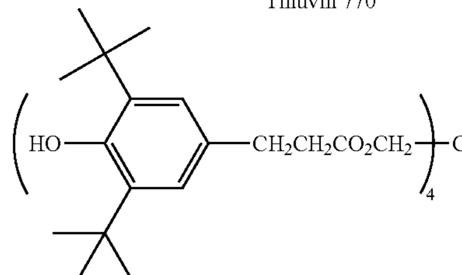
Irganox 1010
