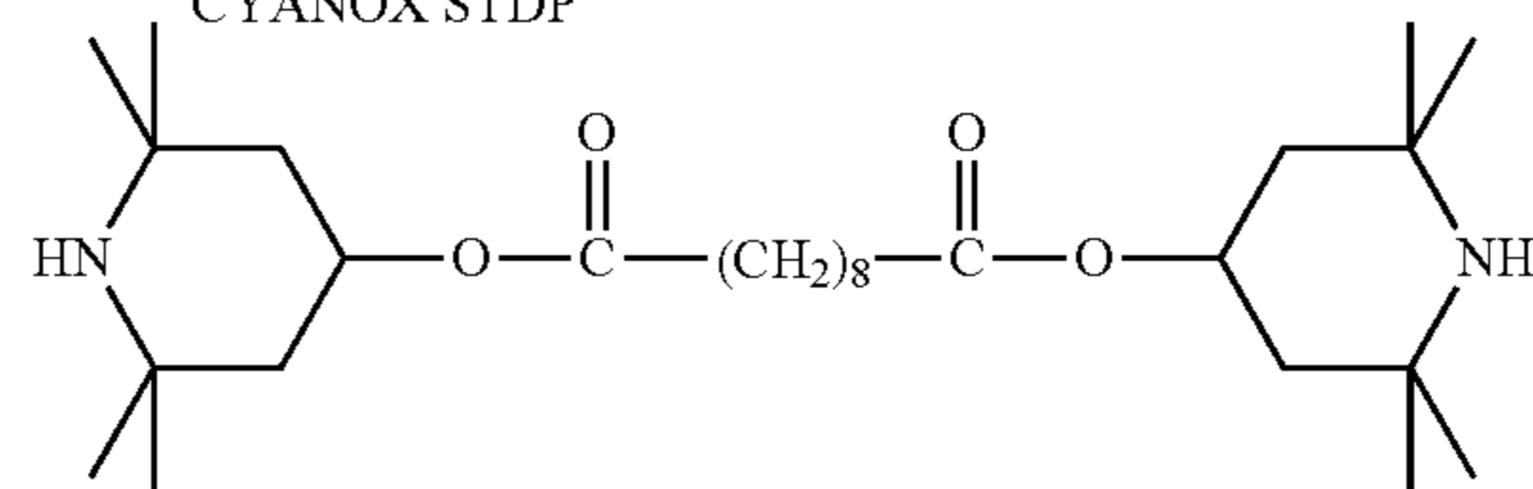
Tinuvin 770
