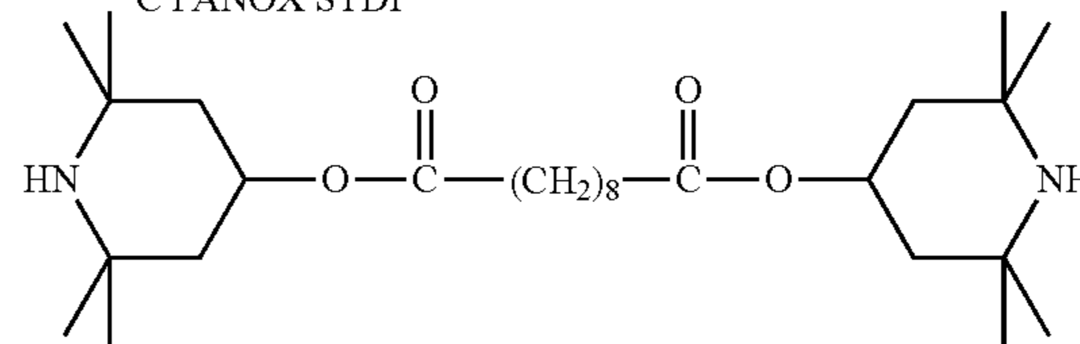
Tinuvin 770
