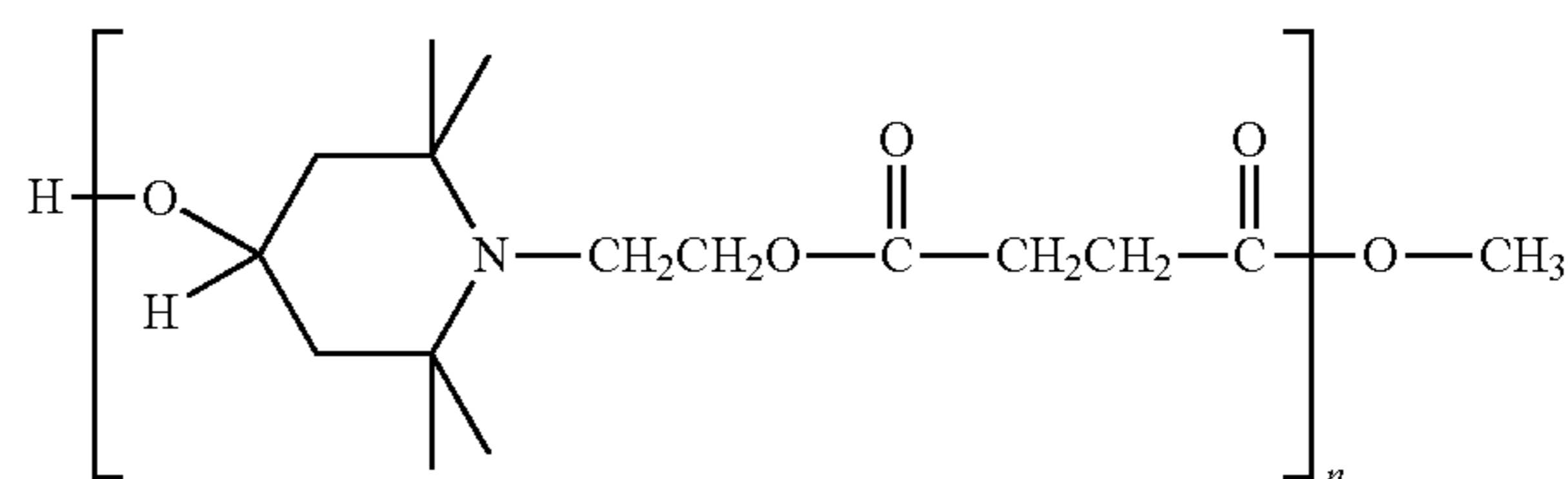
Tinuvin 622
