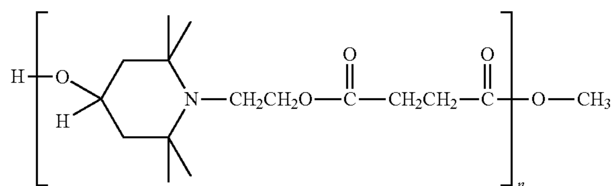
Tinuvin 622
