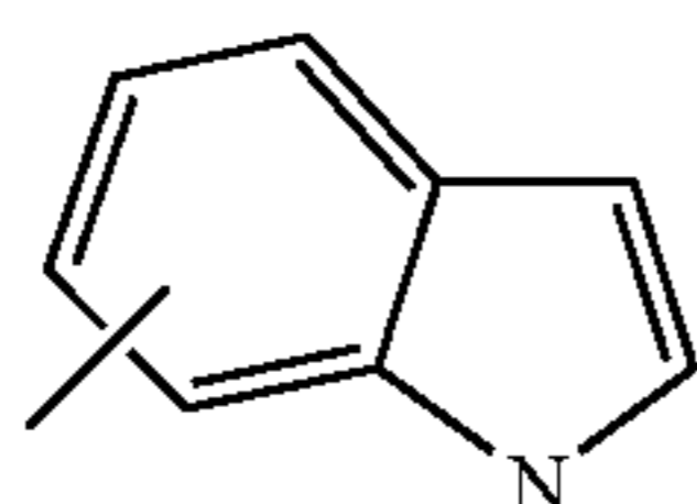
indyl
