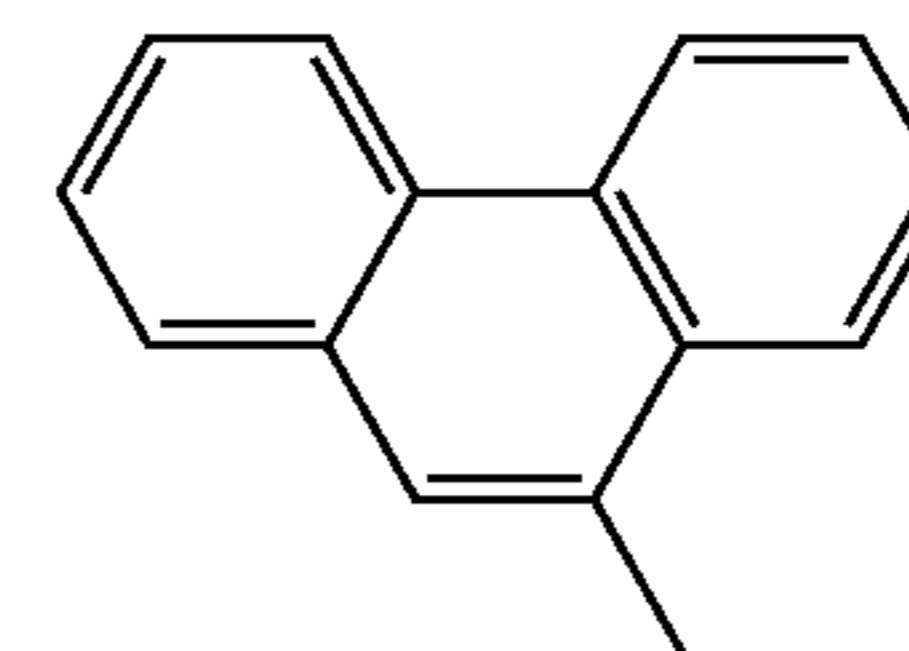
9-phenanthryl
