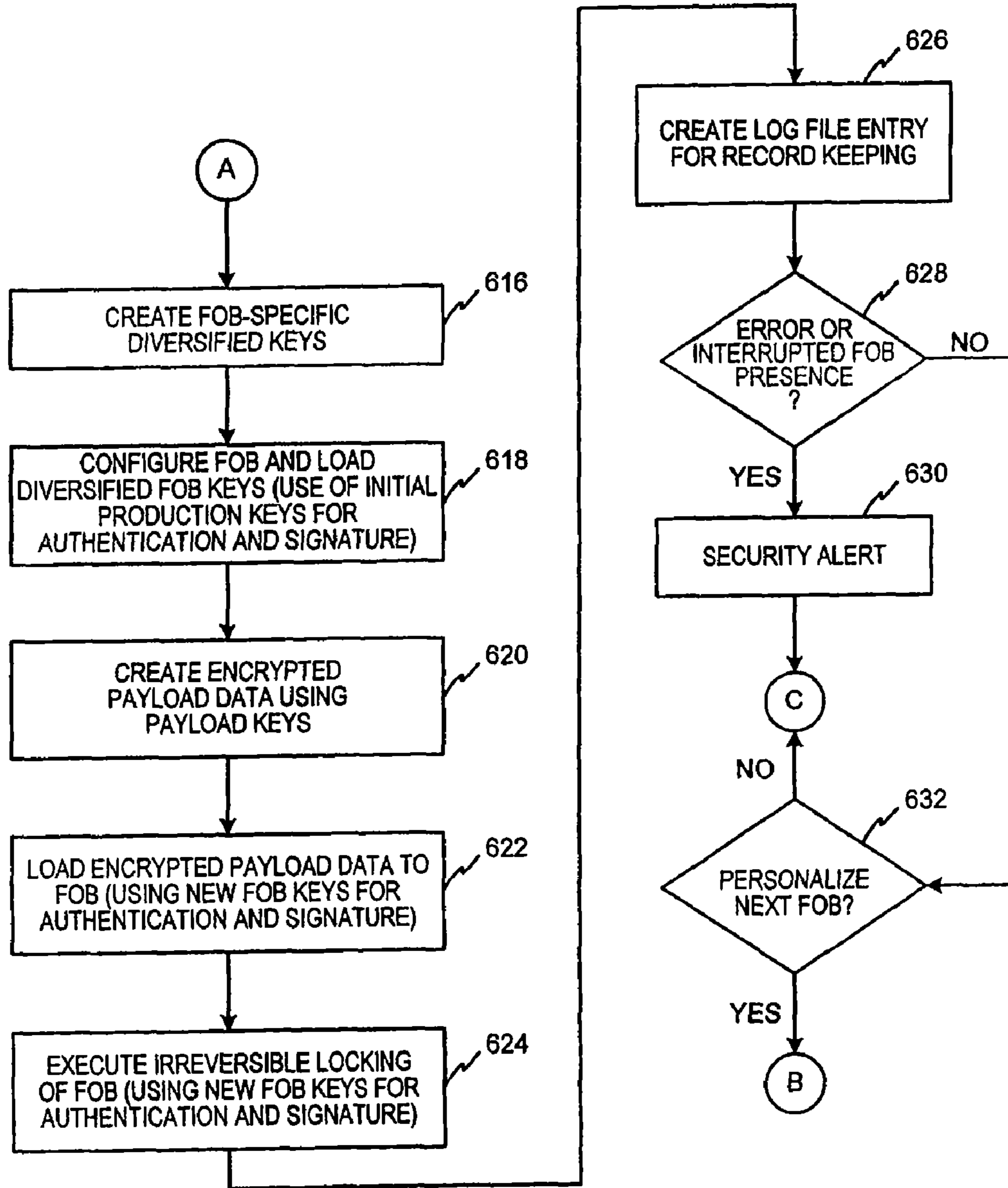
FIG. 6B
