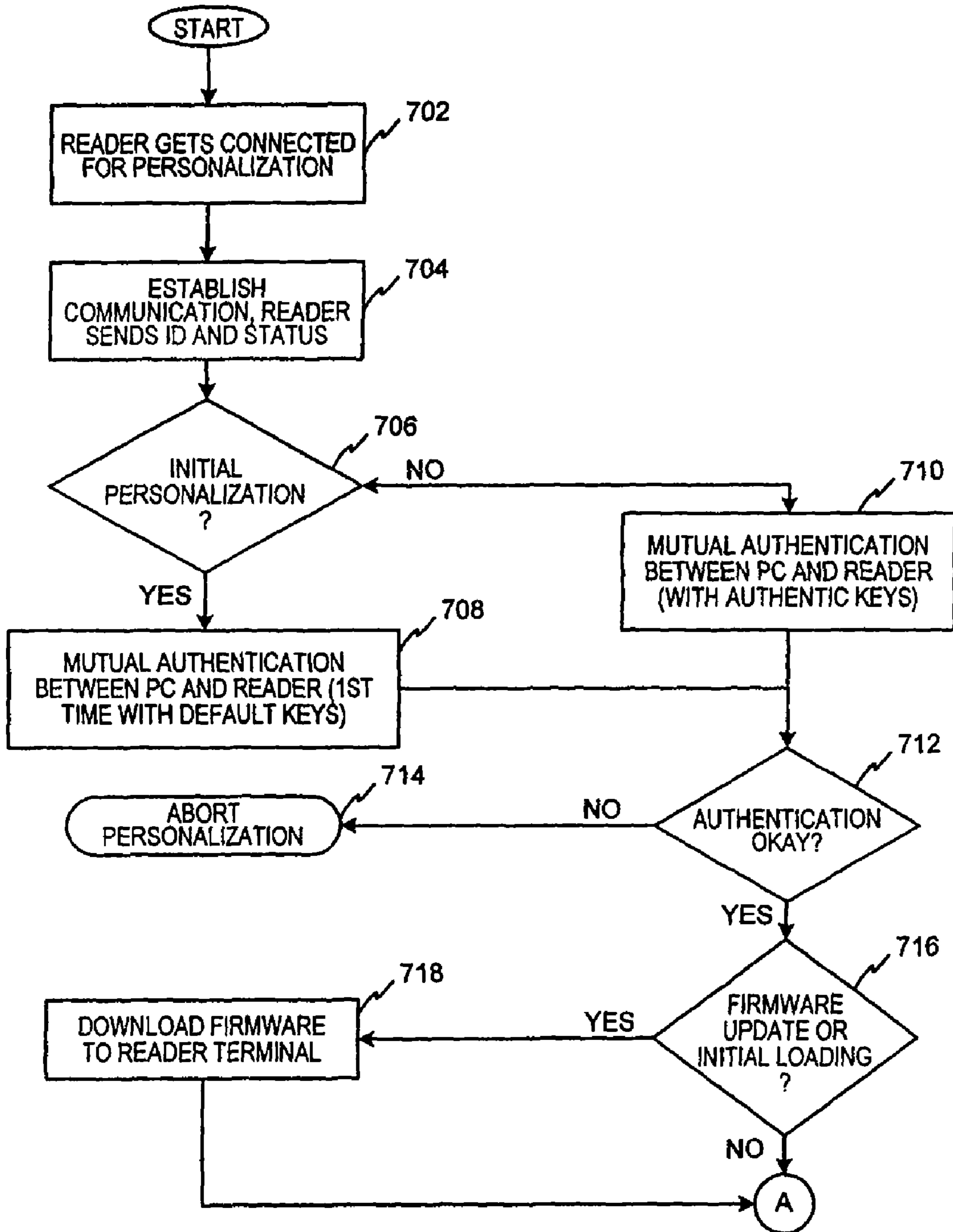
FIG. 7A
