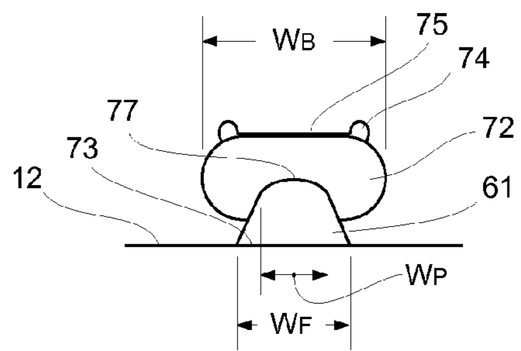
FIG. 7D
