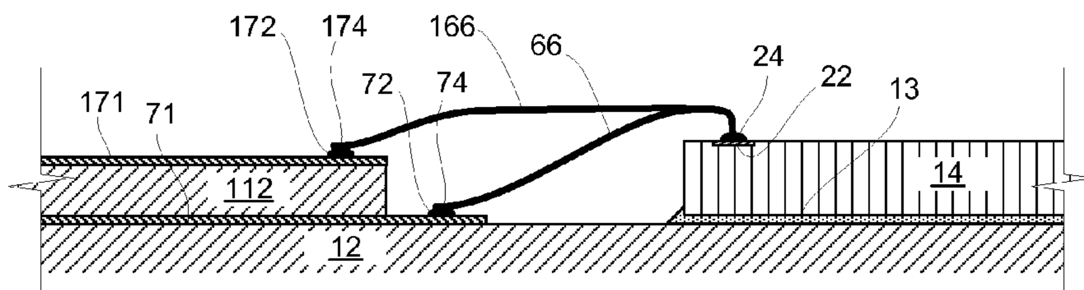
FIG. 10A
