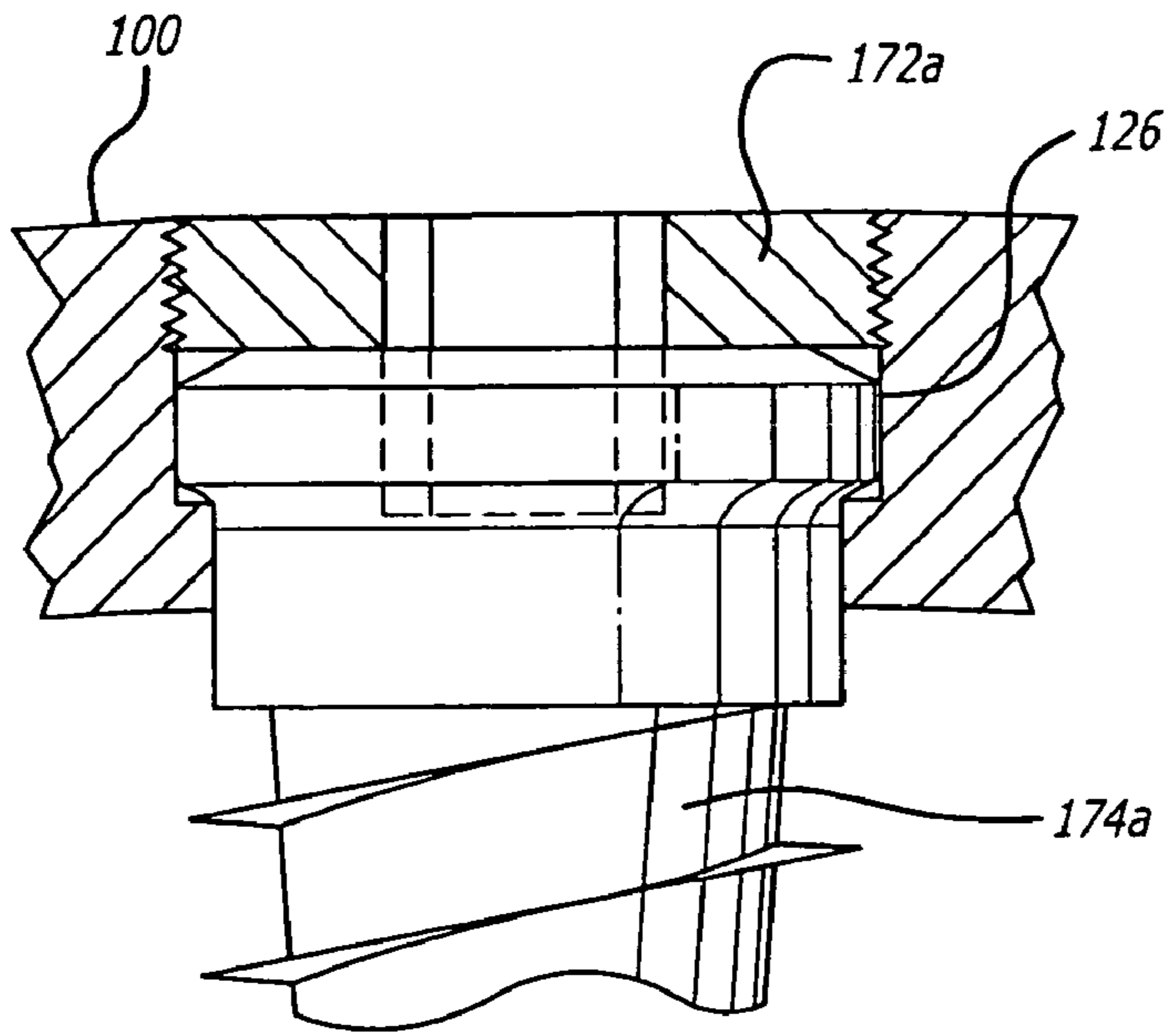
FIG. 41a
