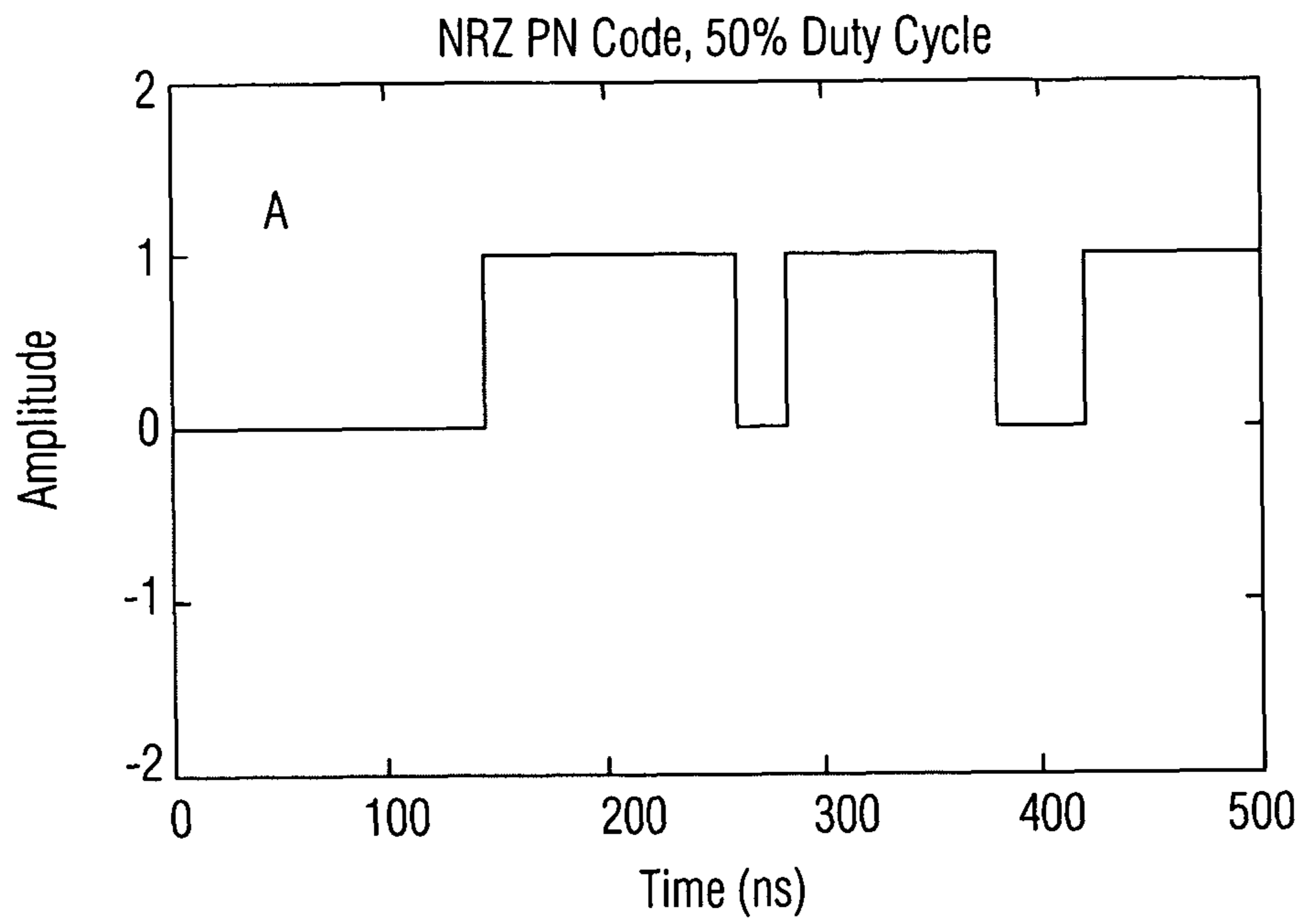
PRIOR ART Fig. 2E
