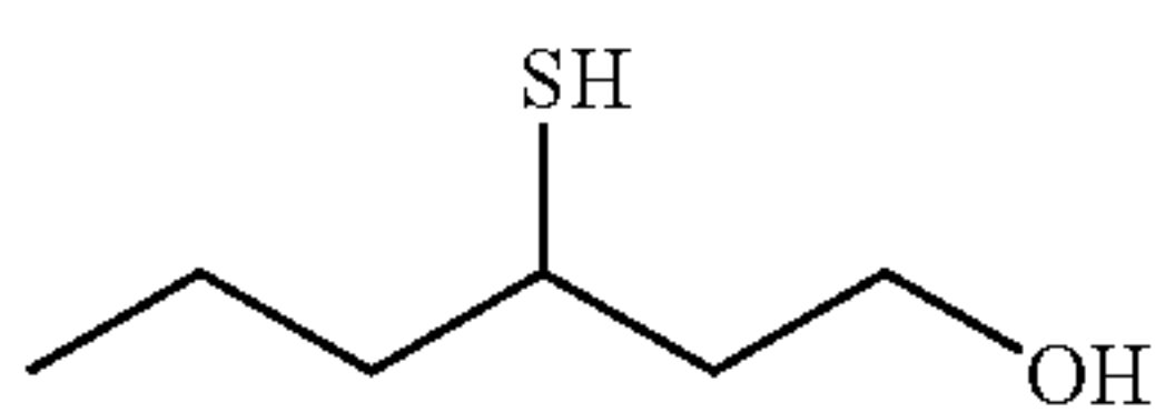
3-mercaptohexanol
