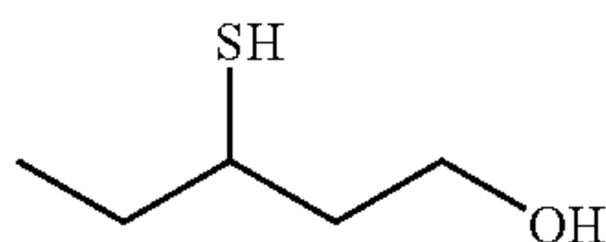
3-mercaptopentanol
