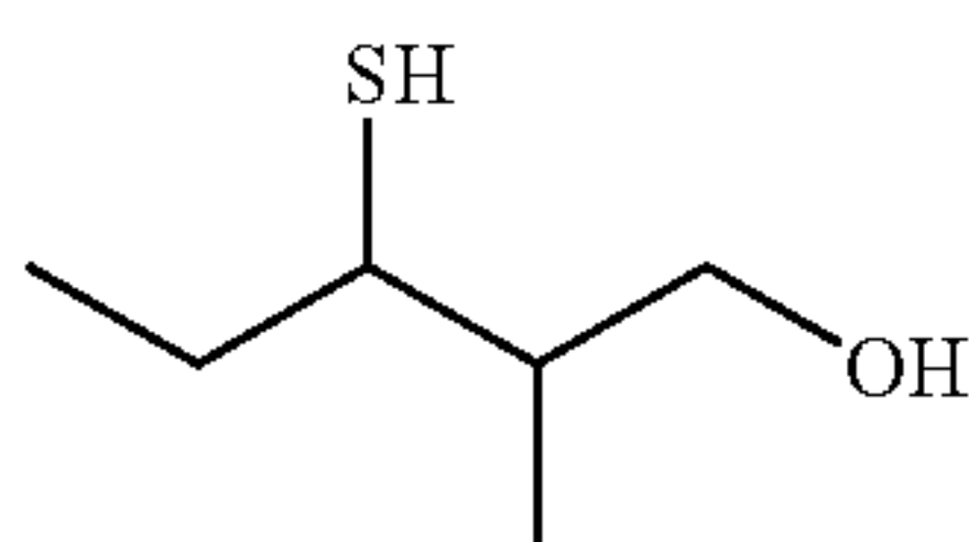
3-mercapto-2-methylpentanol
