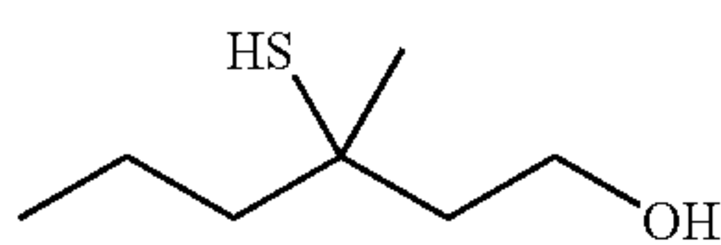
3-mercapto-3-methylhexanol
